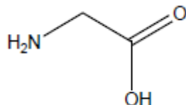
Слика 1.5 Хемијска структура глицина
