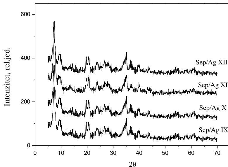
Slika 56. Difraktogrami uzoraka sepiolita modificovanih srebrom dobijenog redukcijom metil-alkoholom
