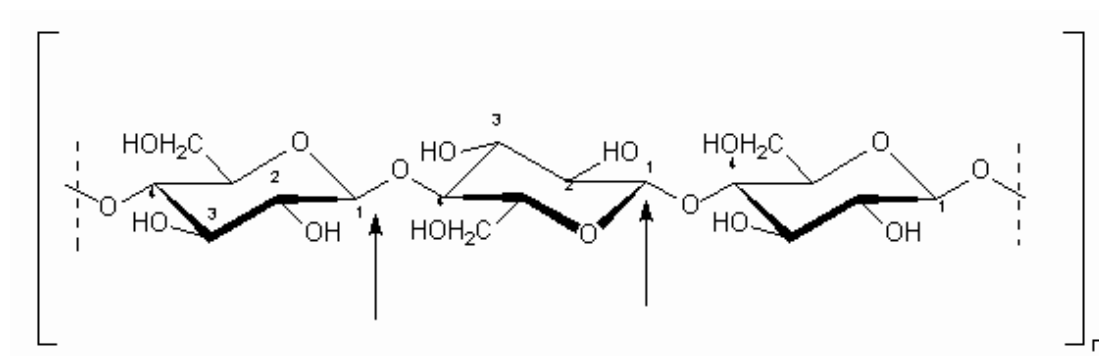
Slika 7. Strukturna formula molekula celuloze
