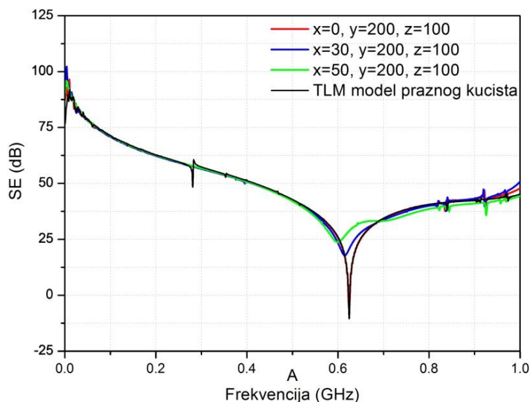
Slika 7.5 SE kućišta sa jednim otvorom dimenzija (50x10) mm 2 pobuđeno ravanskim talasom vertikalne polarizacije i normalne incidencije za različite udaljenosti Cu-štampane dipol antene od zida sa otvorima
