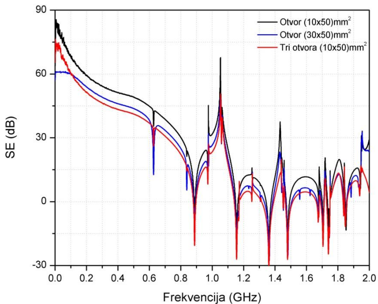
Slika 6.27 SE kućišta sa monopol antenom opterećenom impedansom koaksijalnog kabla za tri vrste otvora za slučaj kose incidencije ravanskog talasa (azimuth 60^\circ , elevacija 90^\circ i polarizacija 30^\circ )
