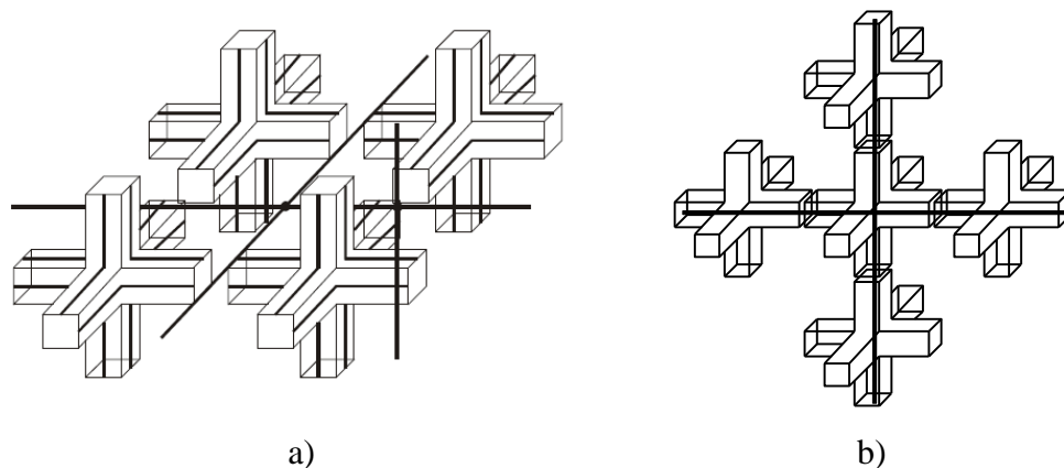
Slika 3.7 Dodatna žičana mreža ubačena a) između čvorova i b) unutar čvorova
