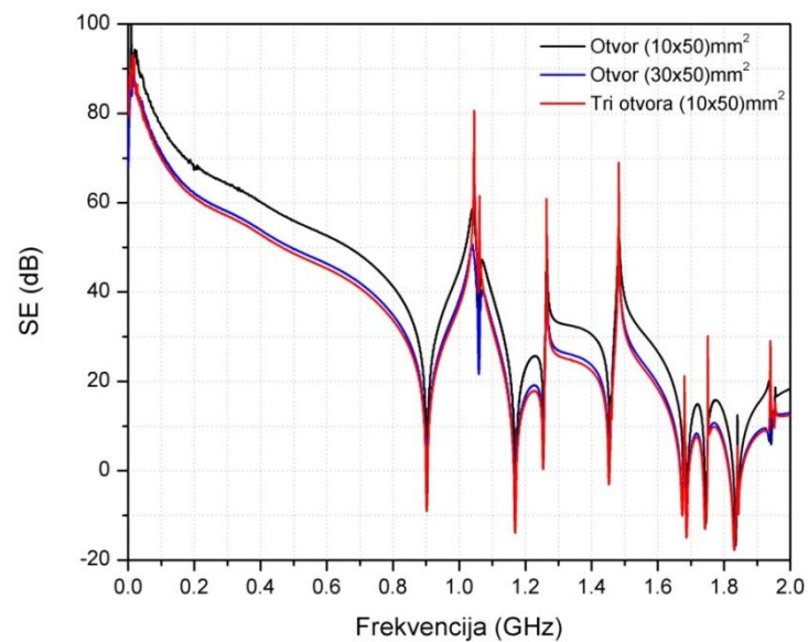
Slika 6.21 SE praznog kućišta sa različitim konfiguracijama otvora na prednjem zidu
