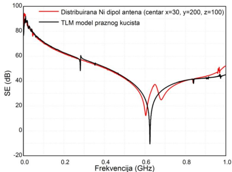
Slika 7.9 SE kućišta sa jednim otvorom ( 50 \times 10 ) \text{mm}^2 pobuđeno ravanskim talasom vertikalne polarizacije Ni-štampana dipol antenna sa distribuiranom otpornošću i TLM model praznog kućišta
