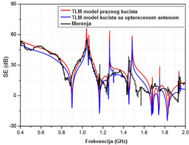
Slika 6.30 SE kućišta sa jednim otvorom dimenzija (10 \times 50) mm 2 na prednjem zidu - TLM model kućišta sa antenom, sa opterećenom antenom i merenja [43]
