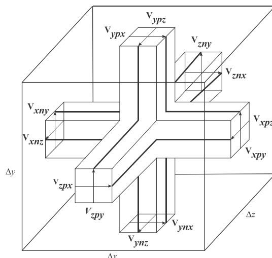
Slika 3.4 Simetrični kondenzovani čvor - SCN
