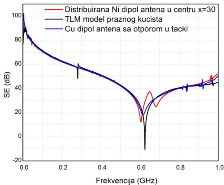
Slika 7.10 SE kućišta sa jednim otvorom ( 50 \times 10 ) \text{mm}^2 pobuđeno ravanskim talasom vertikalne polarizacije - Ni-štampana dipol antenna sa distribuiranom otpornošću, 50 \Omega otporno opterećena Cu-štampana dipol antenna i TLM model praznog kućišta
