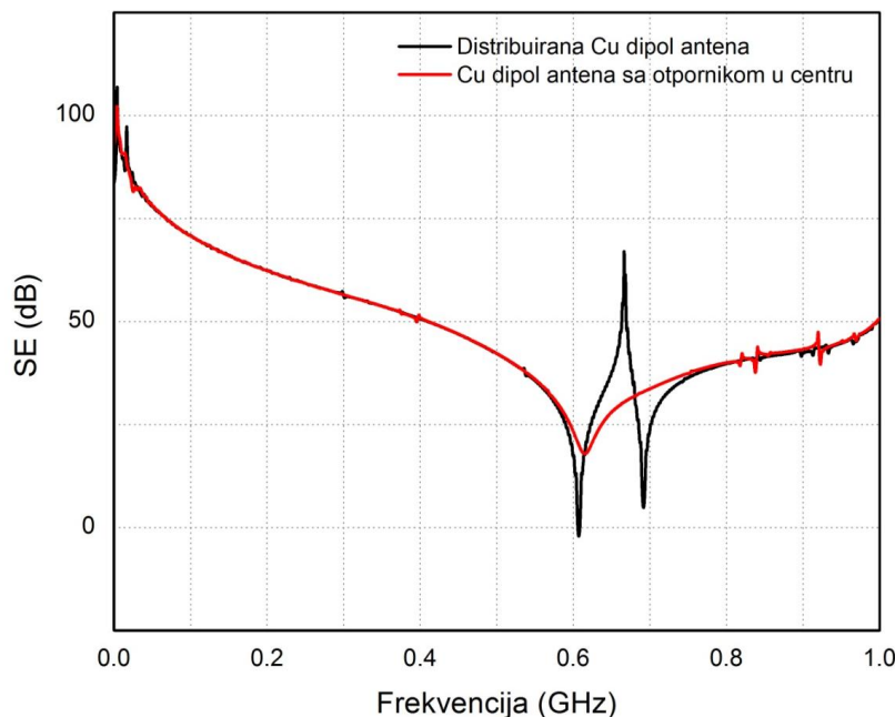
Slika 7.8 SE kućišta sa jednim otvorom dimenzija (50 \times 10) \text{ mm}^2 pobuđeno ravanskim talasom vertikalne polarizacije i normalne incidencije – 50 \Omega otporno opterećena Cu-štampana dipol antenna i Cu-štampana dipol antenna sa distribuiranom otpornošću od 1.5 \Omega po kvadratu
