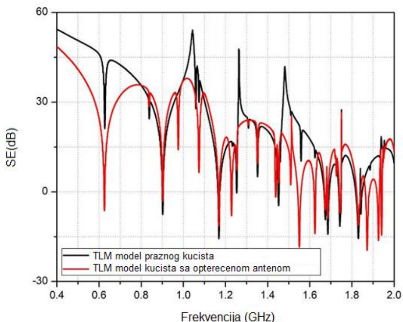
Slika 6.35 SE praznog kućišta i kućišta opterećenom antenom uz ravanski talas kose incidencije (azimutnim uglom 60^\circ , elevacionim uglom 90^\circ i polarizacionim uglom 30^\circ ) kao pobuda
