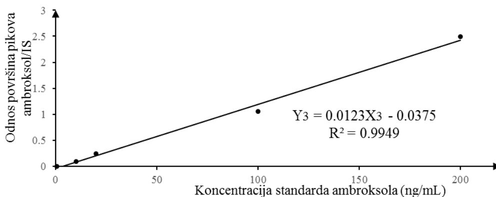
Slika 4.1.2.3. Kalibraciona kriva 3STD standarda ambroksola (0.5-10-20-100-200 ng/mL) u odnosu na IS (20 ng/mL verapamila); UHPLC-MS/MS
