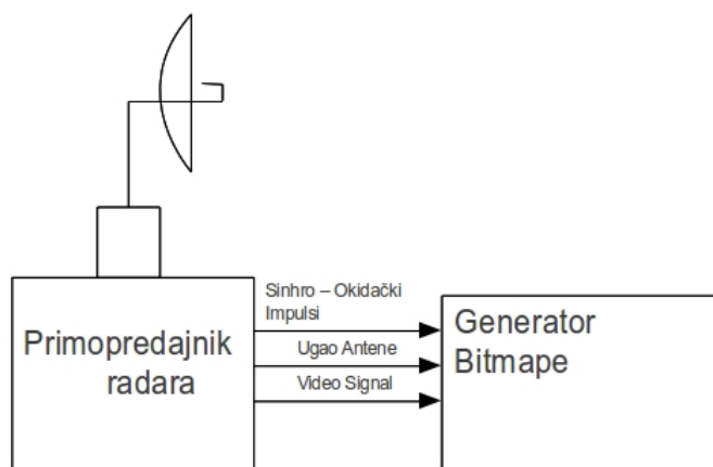
Slika 1.8: Pricipijelna blok šemu platforme na kojoj su vršeni experimenti pomenuti u ovoj tezi
