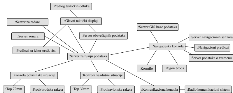
Slika 5.2: Dijagram razmeštaja celina za komandno informacijski sistem ratnog broda
