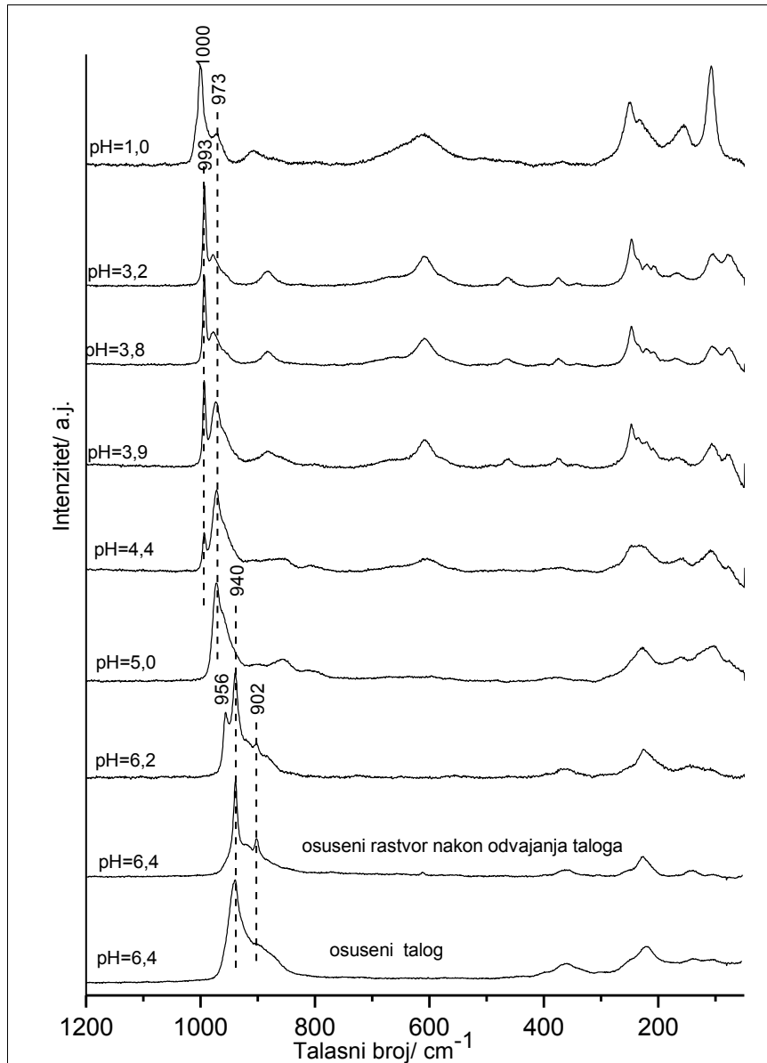
Slika 43. Ramanski spektri suvih ostataka rastvora MoPA polazne koncentracije 5 \cdot 10^{-2} \text{ mol dm}^{-3} u rastvaraču sa početnom koncentracijom metanola 50 %, na različitim pH vrednostima
