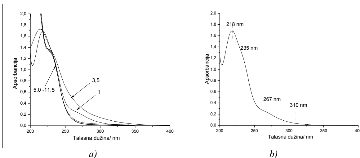
Slika 33. a) ULj spektri rastvora MoPA polazne koncentracije 2 \cdot 10^{-5} \text{ mol dm}^{-3} , na različitim pH vrednostima, b) ULj spektar na pH = 1,0
