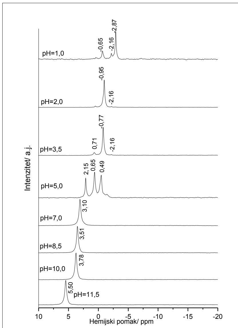
Slika 34. 31 P NMR spektri vodenih rastvora MoPA polazne koncentracije 5 \cdot 10^{-2} \text{ mol dm}^{-3} pri različitim pH vrednostima
