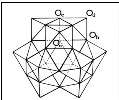
Slika 9. Četiri različita tipa atoma kiseonika u Keggin -ovom anjonu
