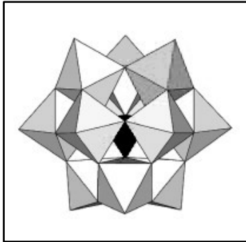
Slika 3. Keggin-ov anjon
