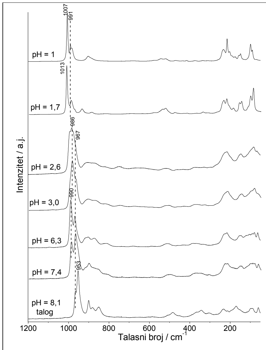
Slika 30. Ramanski spektri suvih ostataka rastvora WPA polazne konc. 5 \cdot 10^{-2} \text{ mol dm}^{-3} u rastvaraču sa polaznim udelom metanola 25 %, na različitim pH vrednostima
