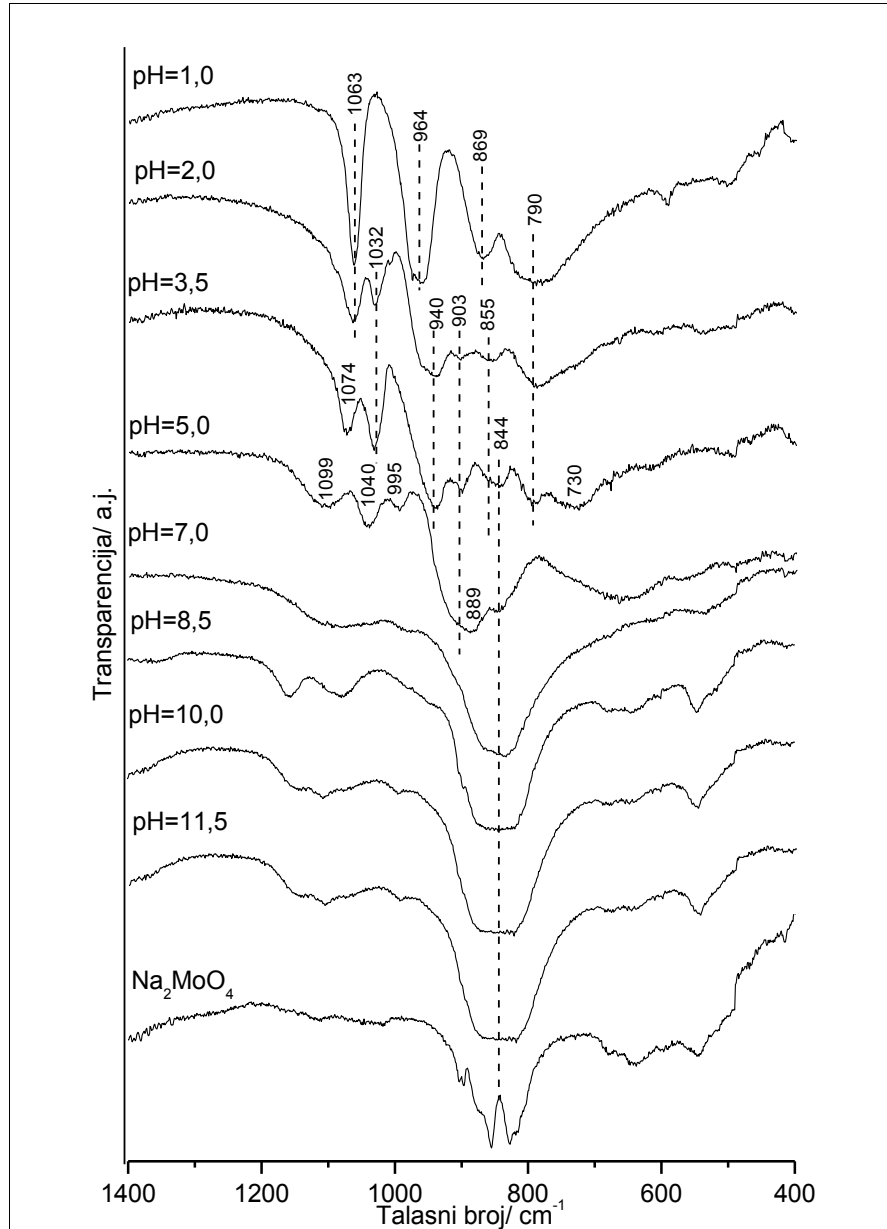
Slika 36. IC spektri suvih ostataka vodenih rastvora MoPA polazne koncentracije 5 \cdot 10^{-2}\text{ moldm}^{-3} na različitim pH vrednostima
