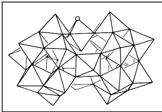
Slika 6. X^n_2W_{21}O_{71}^{(2n-16)-} anjon
