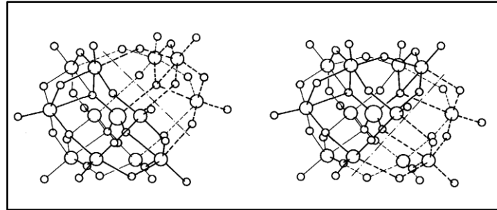
Slika 4. X^nM_9O_{31}^{(8-n)-} struktura izvedena iz Keggin-ove strukture, levo: uklanjanjem 3 atoma metala iz jedne M_3O_{13} grupe (A-tip), desno: uklanjanjem 3 atoma metala iz susednih grupa (B-tip)
