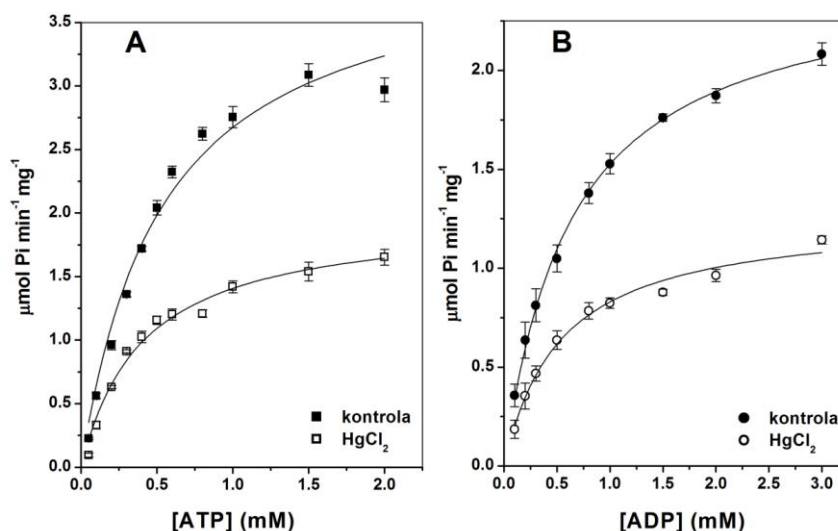
Slika 3.26 Aktivnost E-NTPDaza u zavisnosti od koncentracije ATP (A) i ADP (B) bez (■, ●) i u prisustvu 1×10 -3 M HgCl 2 (□, ○). Rezultati predstavljaju srednje vrednosti specifične aktivnosti enzima \pm se, n=3
