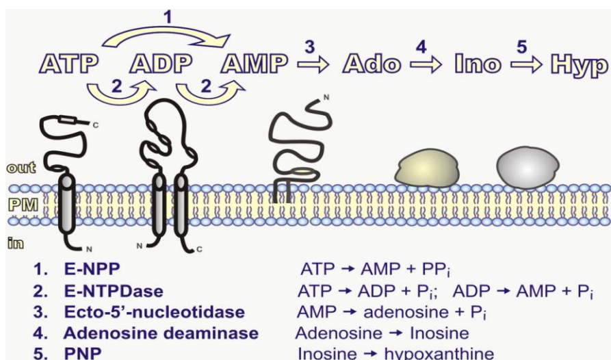
Slika 1.4 Enzimi uključeni u inaktivaciju purinskih nukleotida, sa prikazanim odgovarajućim reakcionim shemama (Yegutkin, 2008)
