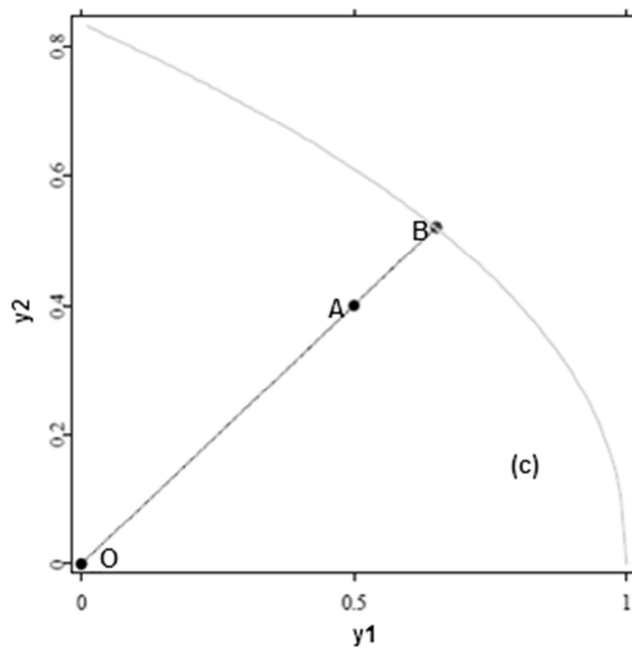
Sl.2.1(c) Reprezentacija izlaznog skupa Y(x) , za dati nivo ulaza x ( s=2 ), [Hardle and Jeong, 2005]
