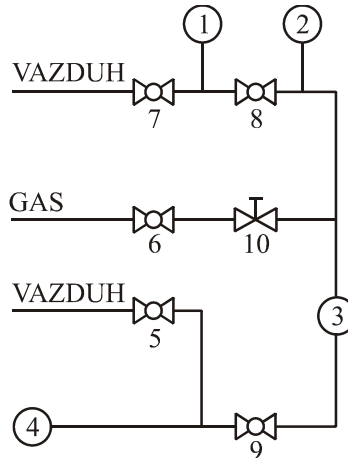
Slika 4.2 Dijagram ispitnog kruga-gasnog kola (1 –apsolutni instrument, 2 – relativni instrument, 3 – komora , 4 – vakuum pumpa, 5, 6, 7, 8 i 9 su dvo-pozicioni ventili, 10 - ventil za mikrometarsko doziranje)
