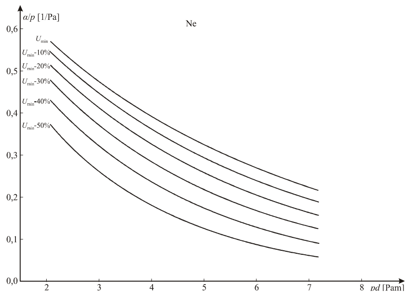
Slika 5.19 \frac{\alpha}{p}(pd) za različite vrednosti probojnog napona za neon
