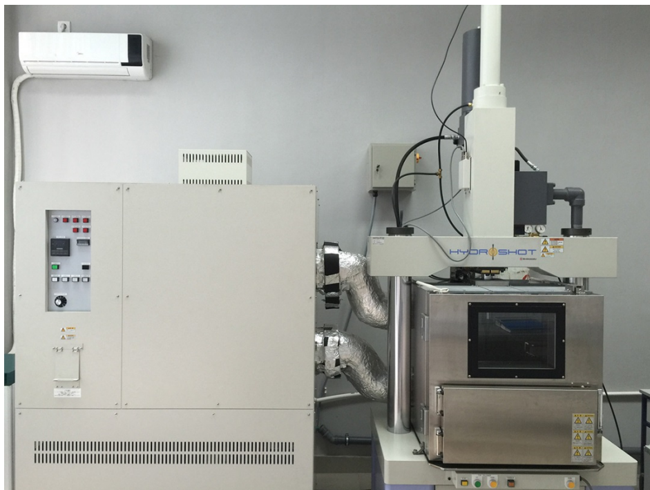
Слика 5.19. Термостатичка комора (лево) и спољашњост импакт тестера
