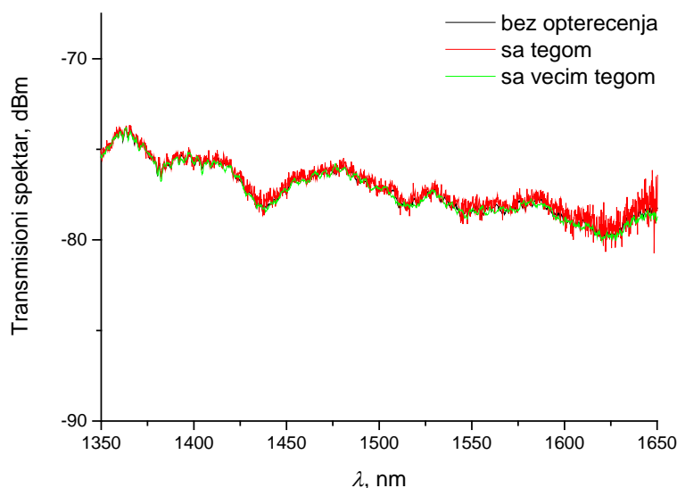
Слика 6.32. Трансмисиони спектар оптичког влакна Т5 без оптерећења и при статичком оптерећењу узорка ПЕВГ-СМ-ЛПГ-1 са две врсте тега
