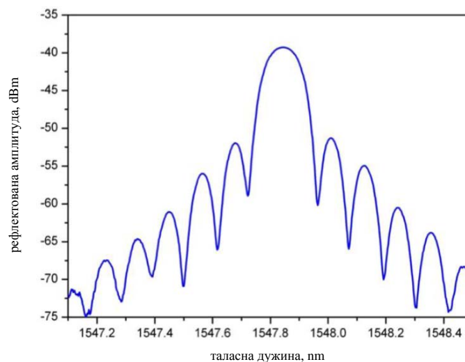
Слика 4.4. Спектар рефлектоване светлости код униформне Брагове решетки дужине 1 cm [41]
