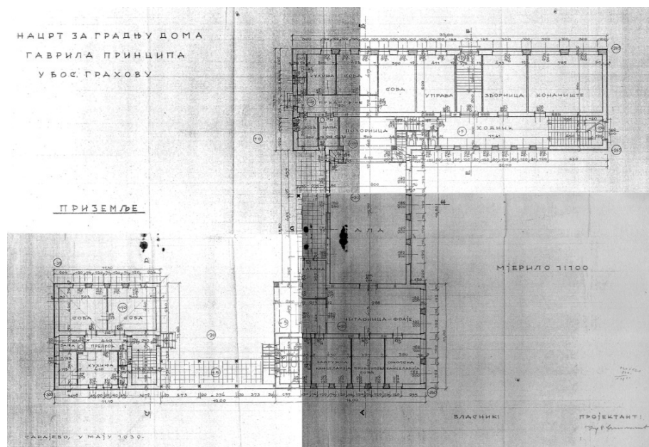
Слика 141 - Пројекат Соколског дома у Босанском Грахову, основа приземља, 1937. (АЈ, Фонд МФВ)
