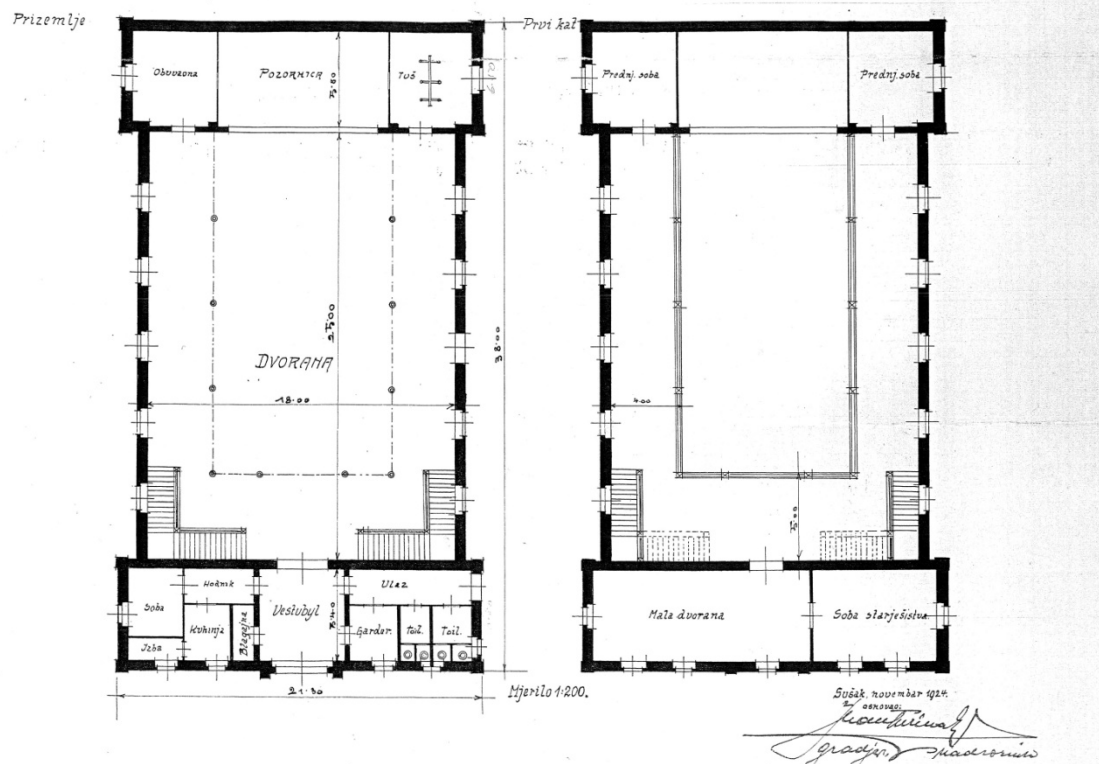
Слика 86 - Пројекат Соколског дома на Сушаку, основа приземља и спрата, 1924. (АЈ, Фонд МП)
