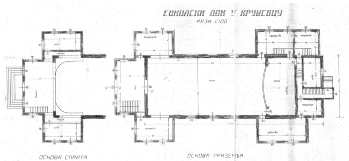
Слика 35 - Пројекат Соколског дома у Крушевцу, основа приземља и спрата, 1927. (АЈ, Фонд МП)
