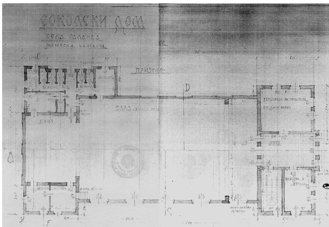
Слика 71 - Тома П. Живановић, Пројекат Соколског дома у Белој Паланци, основа приземља, 1938. (АЈ, Фонд МФВ)
