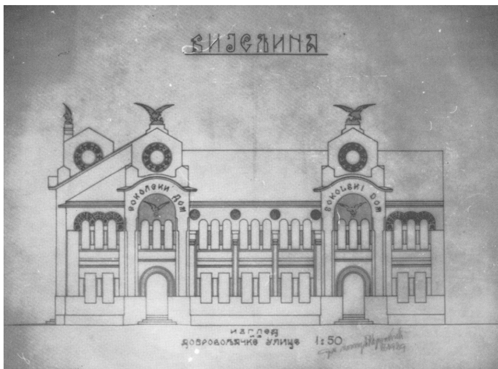
Слика 130 - Момир Коруновић, Пројекат Соколског дома у Бијељини, нацрт прочеља, 1928. (колекција Александра Кадијевића)
