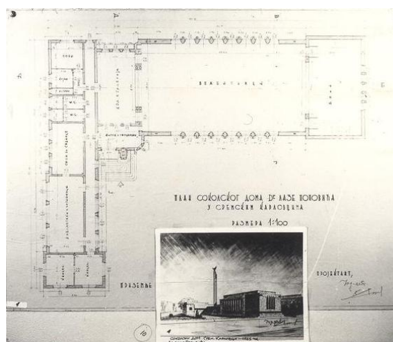
Слика 53 - Светомир Лазић, Пројекат за Соколски дом у Сремским Карловцима, 1937. (колекција Александра Кадијевића)
