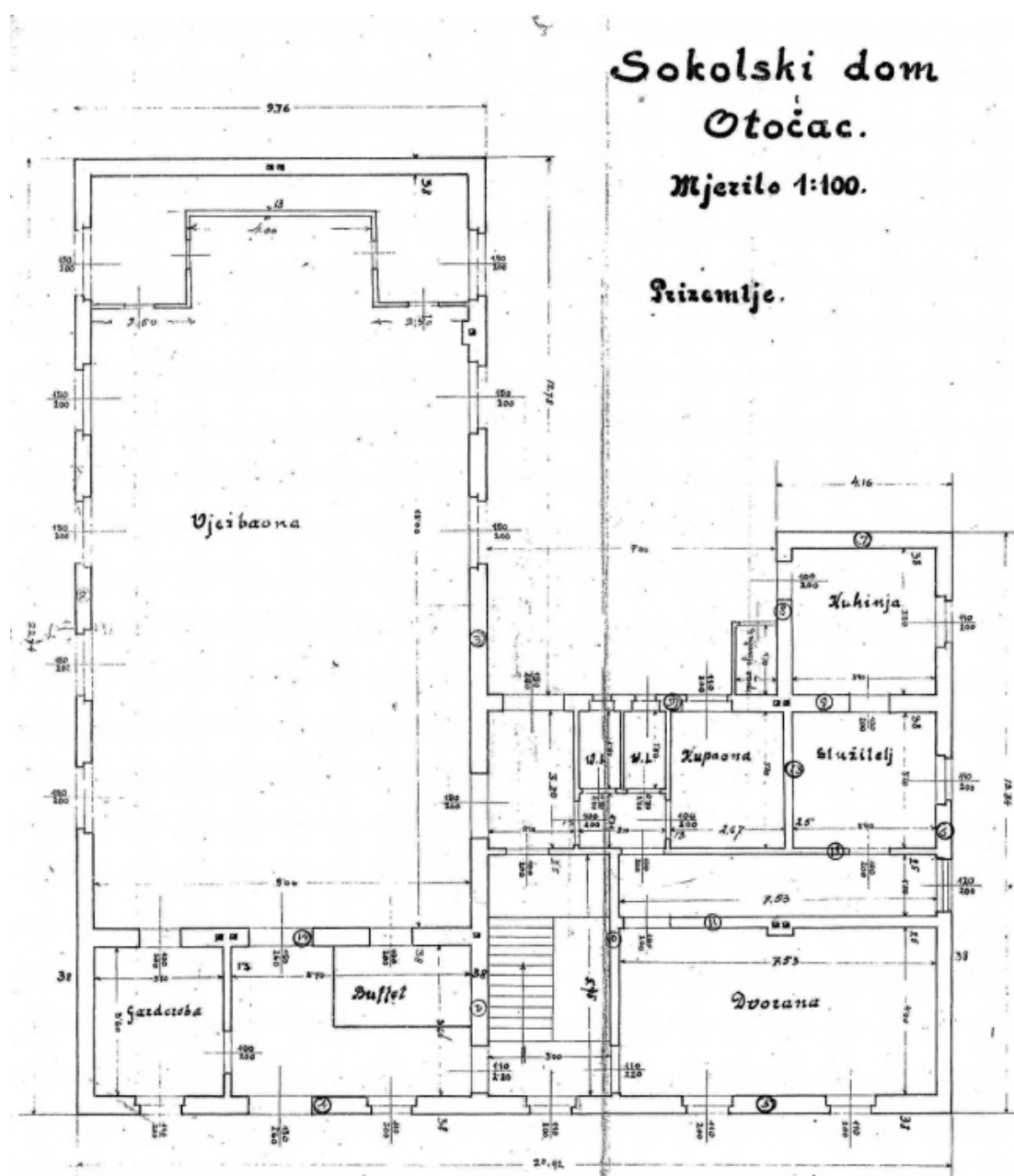
Слика 7 - Соколски дом у Оточцу, основа приземља, 1938. (АЈ, Фонд МФВ)
