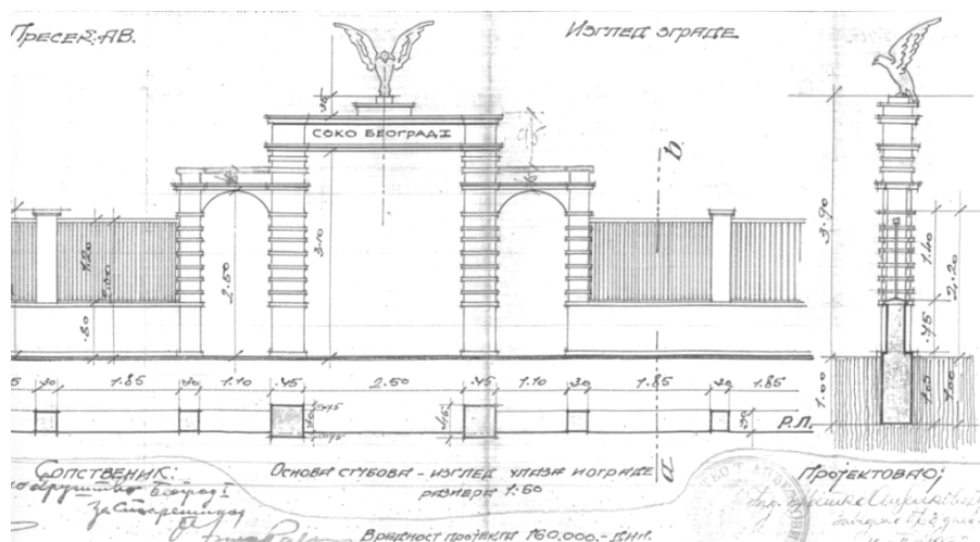
Слика 42 - Цветко Анђелковић, Нацрт капије летњег вежбалишта Соколског друштва Београд I, 1932. (ИАБ)
