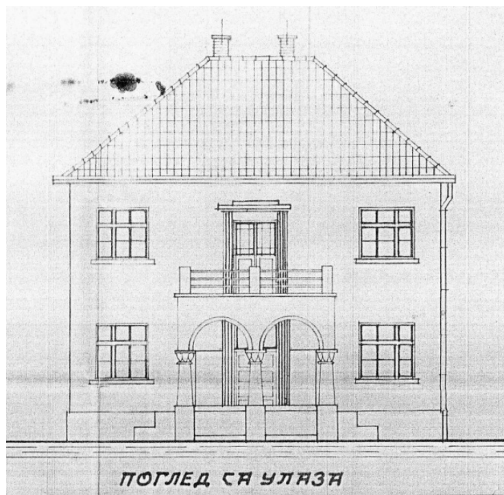
Слика 169 - Иван Грбац, Пројекат Соколског дома у Бољанићу, нацрт прочеља, 1936. (АЈ, Фонд МФВ)
