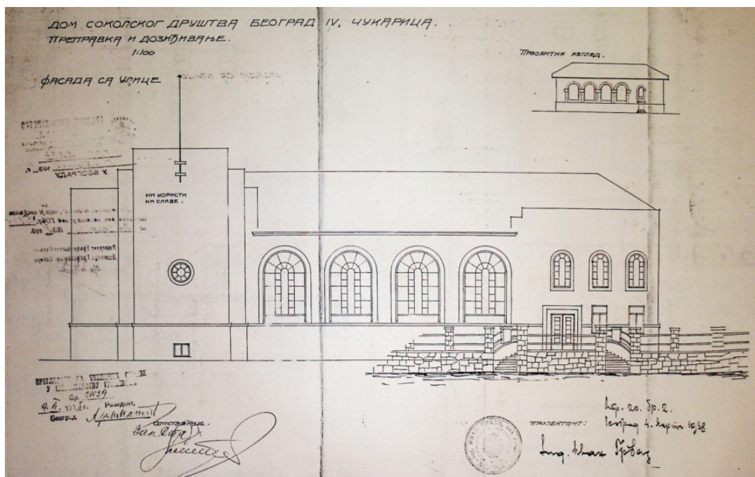
Слика 60 - Иван Грбац, Пројекат доградње Соколског дома Београд IV, 1938. (ИАБ)
