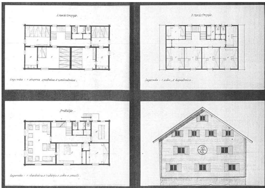
Слика 123 - Пројекат Соколског планинског дома на Похорју, 1939. (АЈ, Фонд МФВ)
