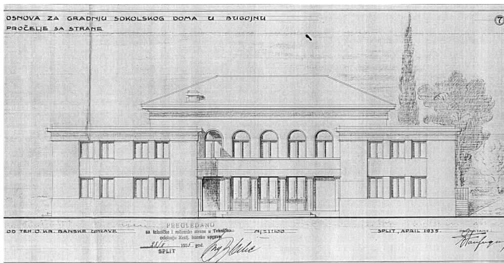
Слика 1366 - Пројекат Соколског дома у Бугојну, нацрт бочне фасаде, 1935. (АЈ, Фонд МФВ)
