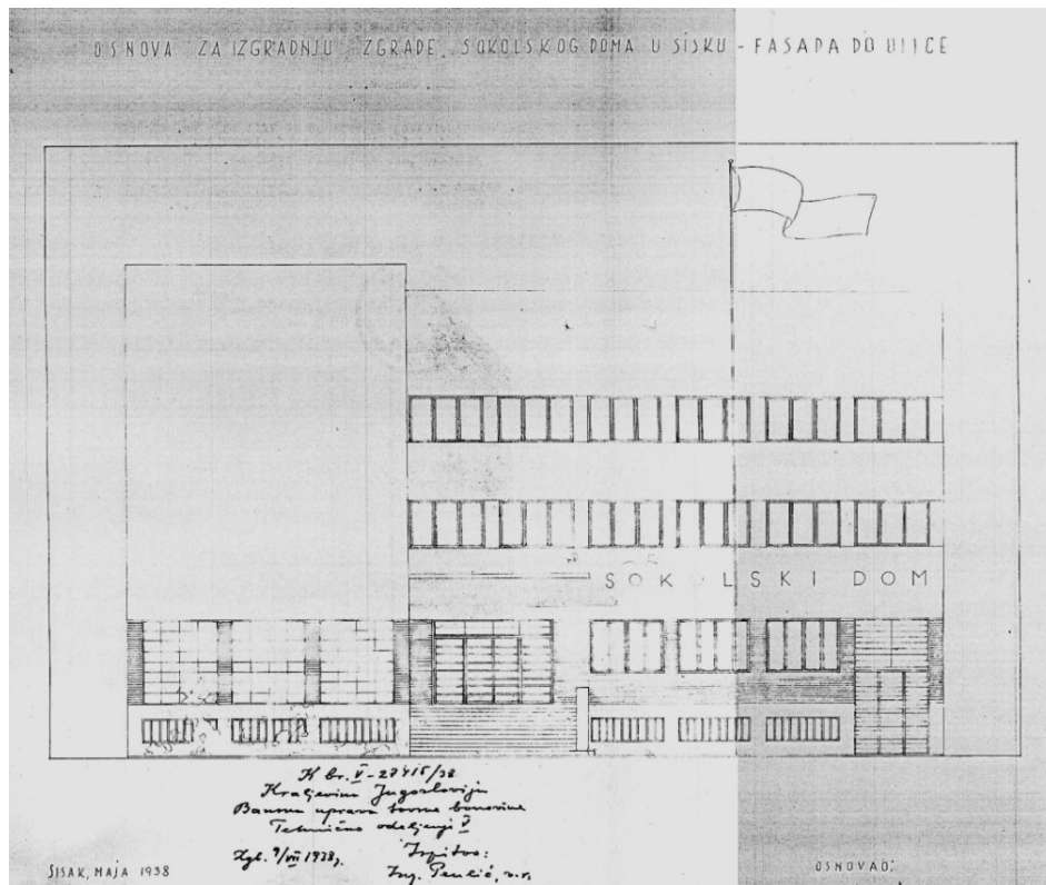
Слика 92 - Стјепан Павлић, Соколски дом у Сиску, нацрт pročеља, 1938. (АЈ, Фонд МФВ)
