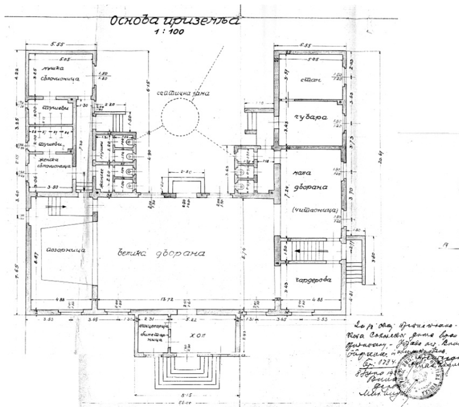
Слика 74 - Пројекат Соколског дома у Вини, основа приземља, 1937. (АЈ, Фонд МФВ)
