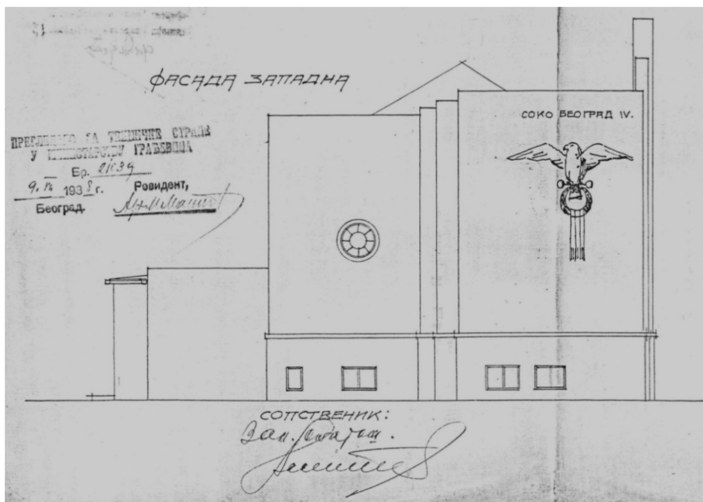
Слика 61 - Иван Грбац, Пројекат доградње Соколског дома Београд IV, западна фасада, 1938. (ИАБ)
