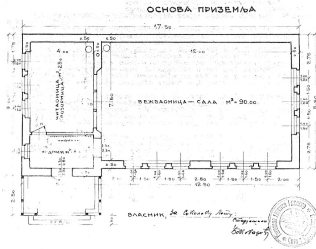
Слика 6 - Соколски дом у Друговићима, основа приземља (АЈ, Фонд МФВ)
