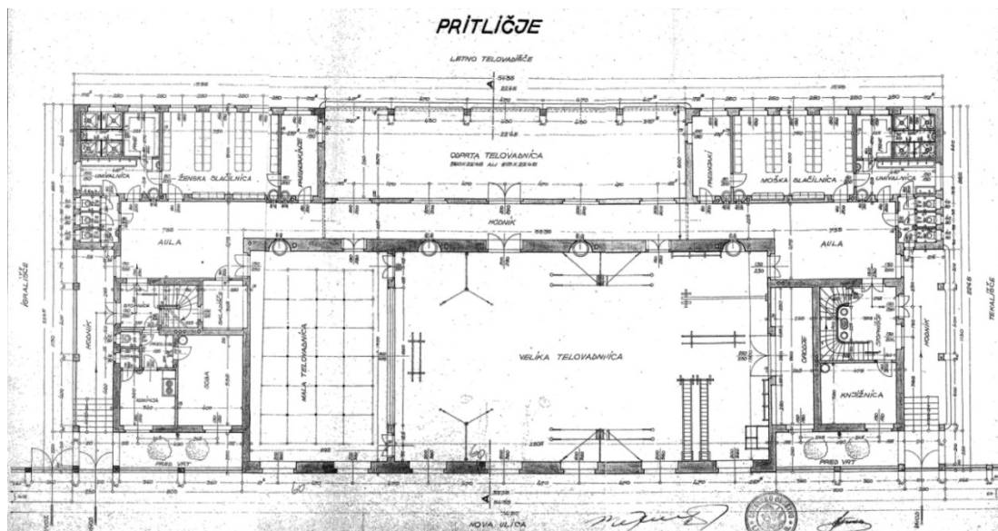
Слика 114 - Пројекат Соколског дома Љубљана II, основа приземља, 1934. (АЈ, Фонд МФВ)
