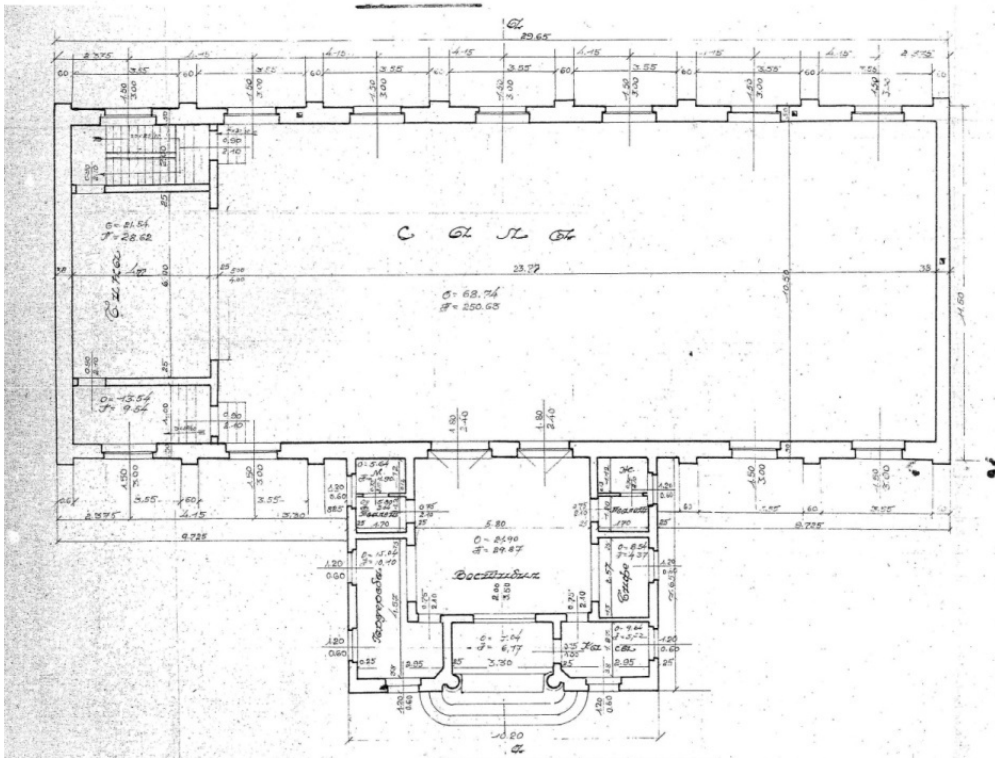
Слика 1516 - Никола Карловић, Пројекат Соколског дома у Гостивару, основа приземља, 1938. (АЈ, Фонд МФВ)
