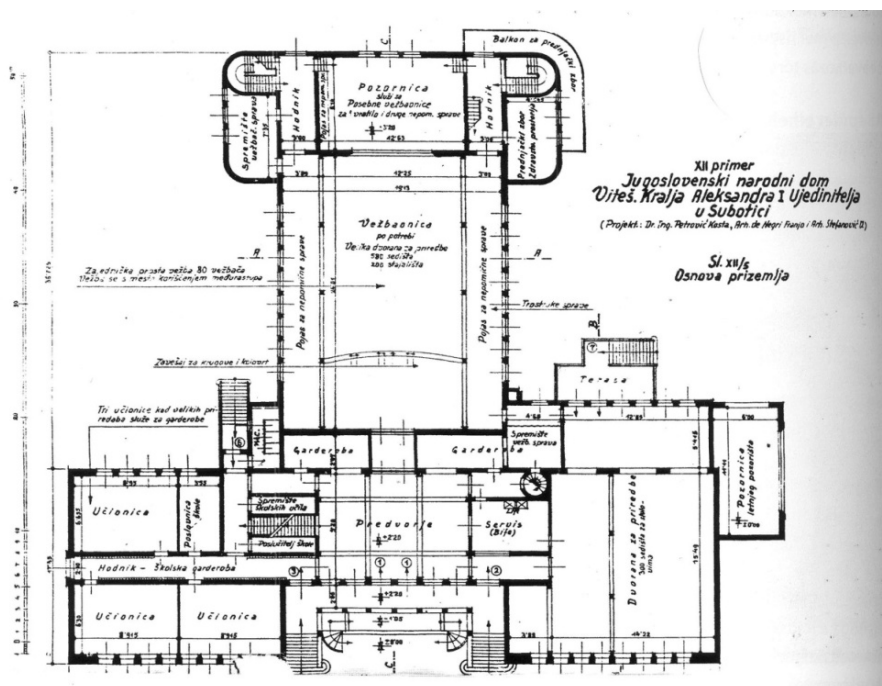
Слика 8 - Југословенски народни дом у Суботици, основа приземља, 1939. (Gabor Demeter, Gordana Prčić-Vujnović, Anka Bratuleanu i Ana Marija Biro, Razvoj urbanizma i arhitekture u periodu od 1918. do 1941. godine u Temišvaru, Segedinu i Subotici - regionalni identitet pod uticajem moderne )
