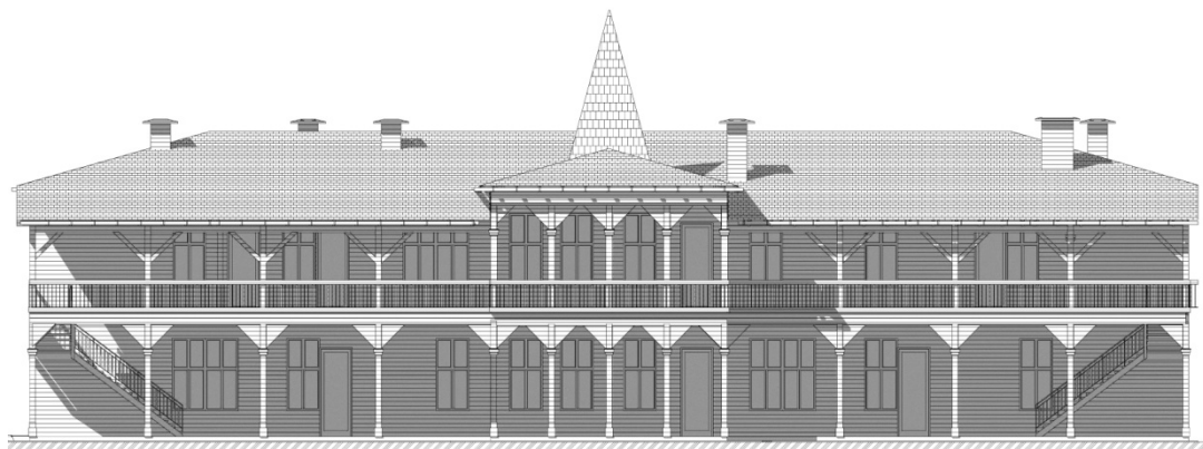
Слика 29 - Нацрт фасаде Соколане у Крагујевцу (Завод за заштиту споменика културе Крагујевац)
