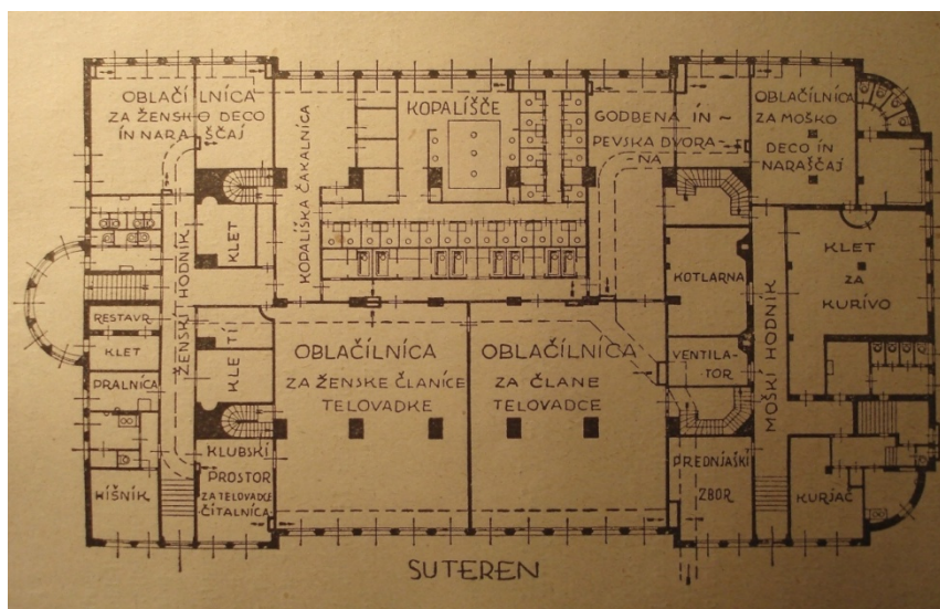
Слика 108 - Иван Вурник, Пројекат Соколског дома „Табор“ у Љубљани, основа сутерена, 1926. ( Соколски гласник )
