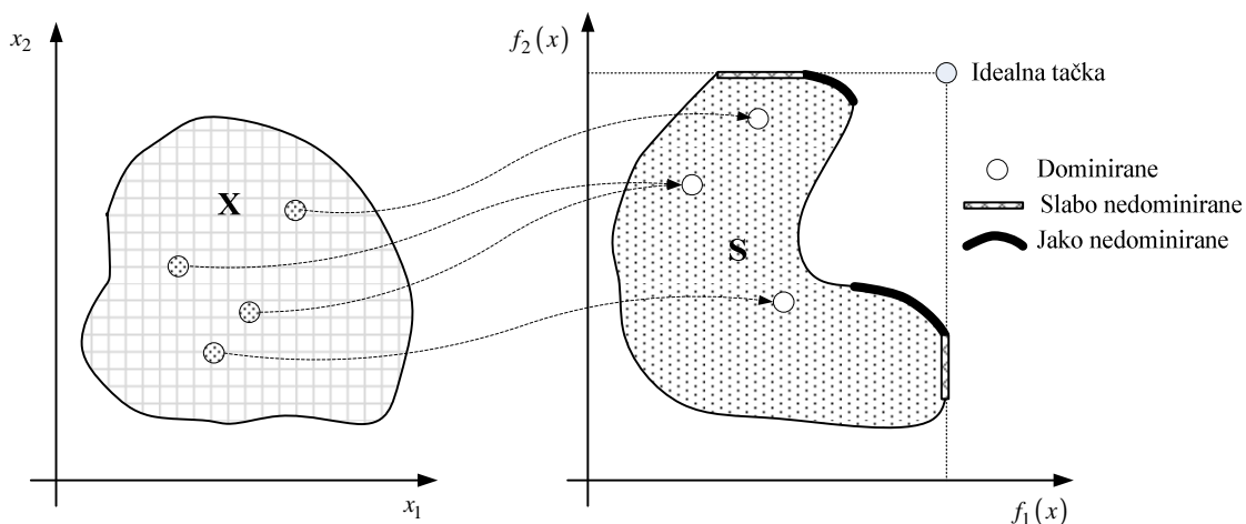
Slika 26. Pareto optimalnost u kriterijumskom prostoru
