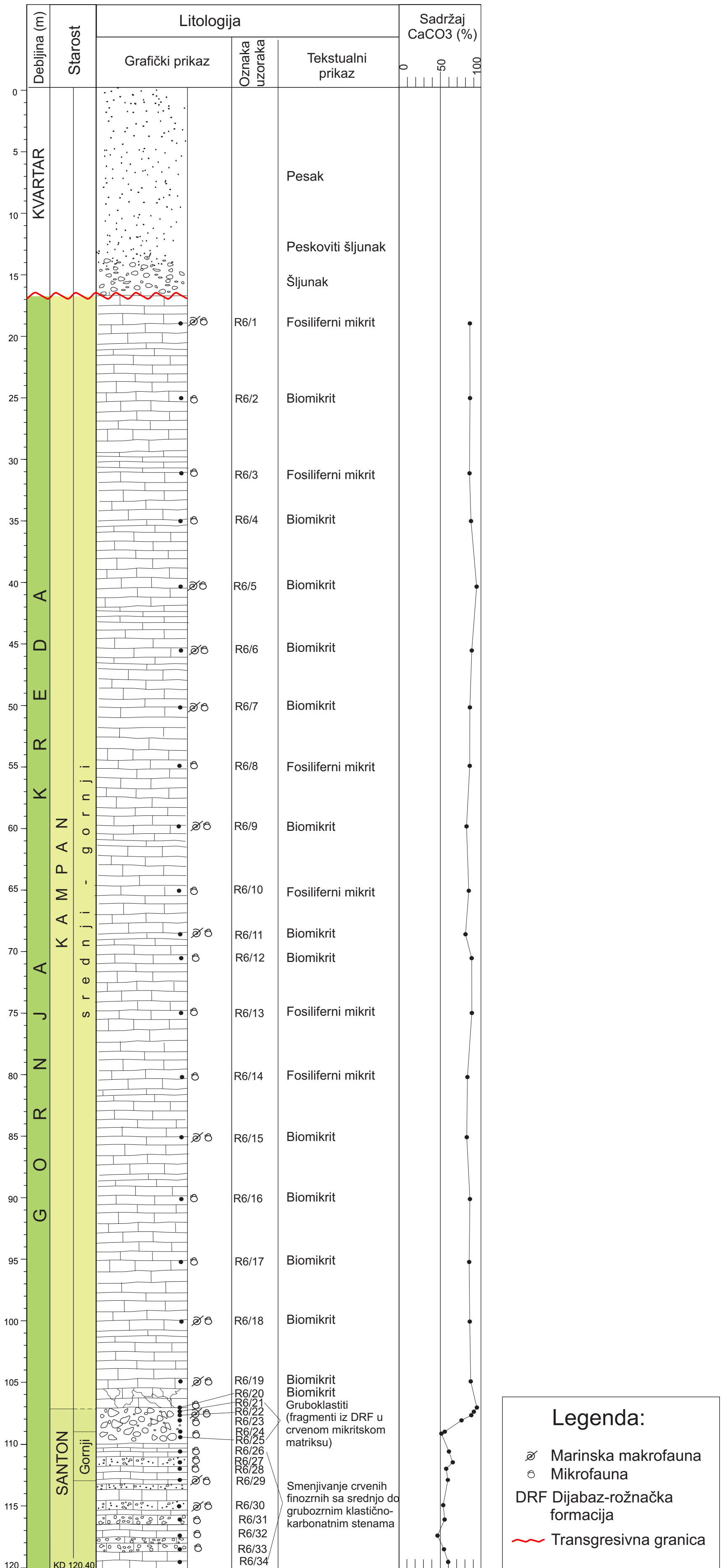
Slika 8.37. Litostratigrafski stub bušotine na Rajcu, kod planinarskog doma.
