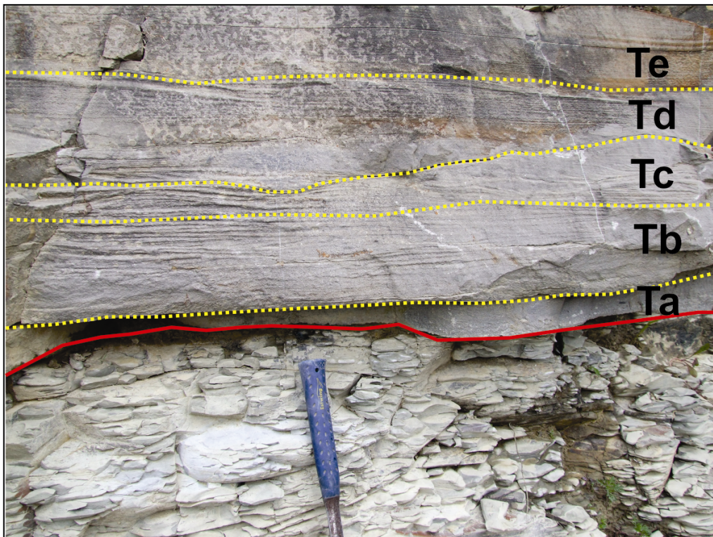
Slika 9.3. Kalkarenit sa kompletno razvijenom Bouminom turbiditnom sekvencom sa intervalima od Ta do Te. U podini je laminirani laporac.
