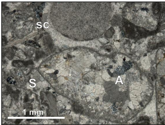
Slika 7.33. Biosparrudit ( rudstone ). Biogena alohema komponenta sa mikritskim omotačima potpuno je prekristalisala (A). sc - sintaksijalni rast kalcita oko fragmenta koral. S - sparitski cement. N+.
