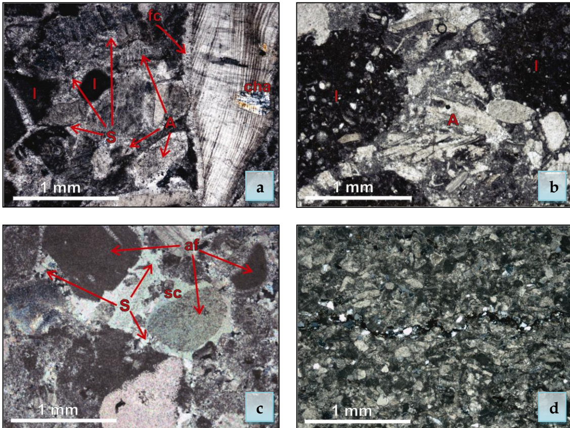
Slika 8.112. Alohemijjski struganički krečnjaci. a. Biosparrudit. U krupnom fragmentu rudista mikrokonkrecije kalcedona (cha). I –intraklasti. A – sitniji biogeni alohem. S – sparikalcit. fc – prekrystalisali fibrozni cement. N+. b. Intra-biomikrurudit. I – krupni složeni intraklasti (odgovaraju mikritima i fosilifernim mikritima). A – sitniji biogeni alohem. NII. c. Krupnozrni biosparit. af – algalni fragmenti. S – sparikalcit. sc – sintaksijalni cement razvijen oko algalnog fragmenta. N+. d. Sitnozrni intra-biosparit. Na sredini slike je stilolitski šav markiran nagomilanjem peskovite komponente. NII.
