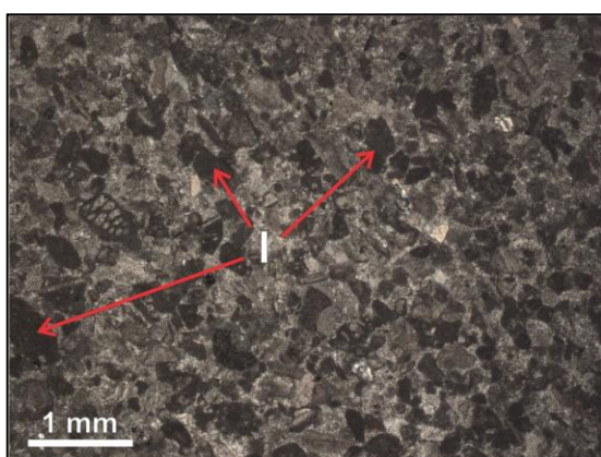
Slika 8.69. Biointrasparit ( grainstone ). Dobra sortiranost alohemijjskih sastojaka u sparitskom cementu. I – intraklasti mikritskog tipa. N+.
