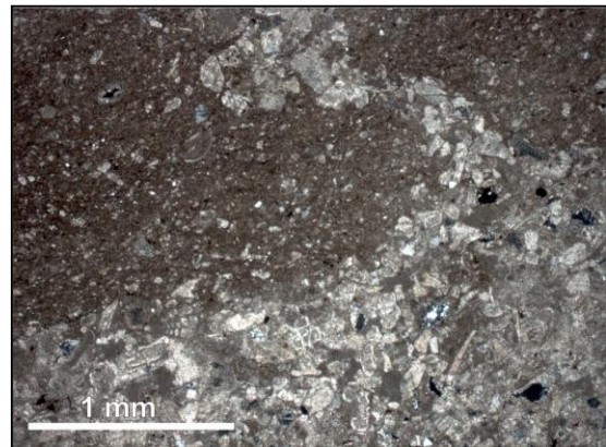
Slika 8.45. Mešanje dve mikrofocije mikritskih krečnjaka. N+.
