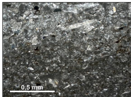
Slika 8.19. Laminirani biomikrit ( wackestone ) N+.
