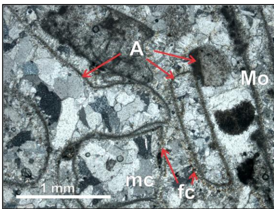
Slika 6.5. Biosparrudit ( rudstone ) izgrađen od bioklasta kao alohema (A) i sparitskog cementa mozaičnog tipa (mc) koji popunjava porni prostor. Konture bioklasta su markirane mikritskim omotačima (Mo), dok je njihov primarni aragonitski sastav zamenjen kristalastim kalcitom. fc – ranodijagenetski fibrozni cement na zidovima alohema. N+.
