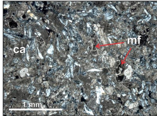
Slika 8.39. Peskoviti krečnjak/litarenit izgrađen od fragmentiranog serpentinskog materijala u mikrokristalastom kalcitskom cementu (ca). mf - ljušturice foraminifera. N+.
