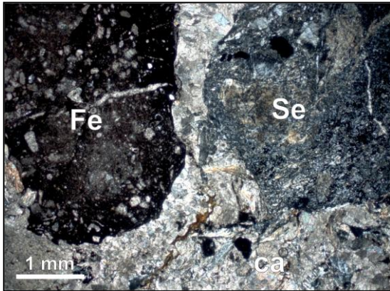
Slika 8.38. Serpentiniski brečo-konglomerat. Se - odlomak serpentinisanog peridotita. Fe - fragment sa kore raspadanja. ca - kristalasti kalcitski cement. N+.
