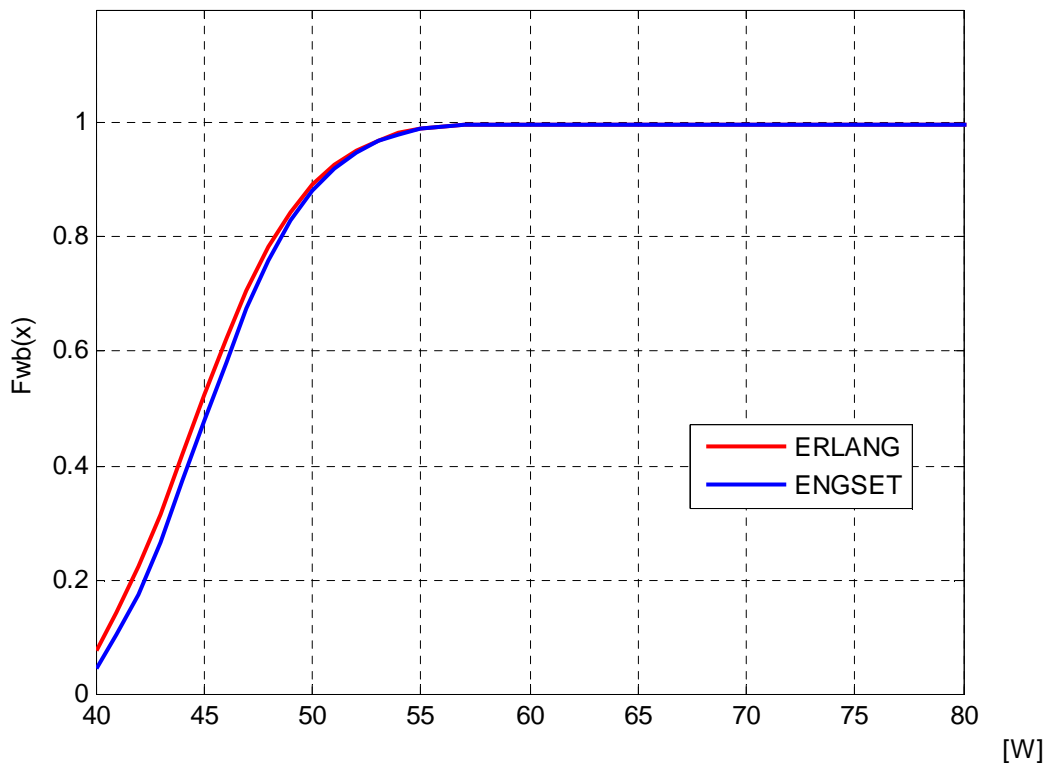
Сл. 6.33 CDF излазне снаге базе станице (поређење модела) (N = 6, A = 4,62, w_{max} = 40 W, R = 10 \text{ km}, \gamma = 4, M = 9) .
