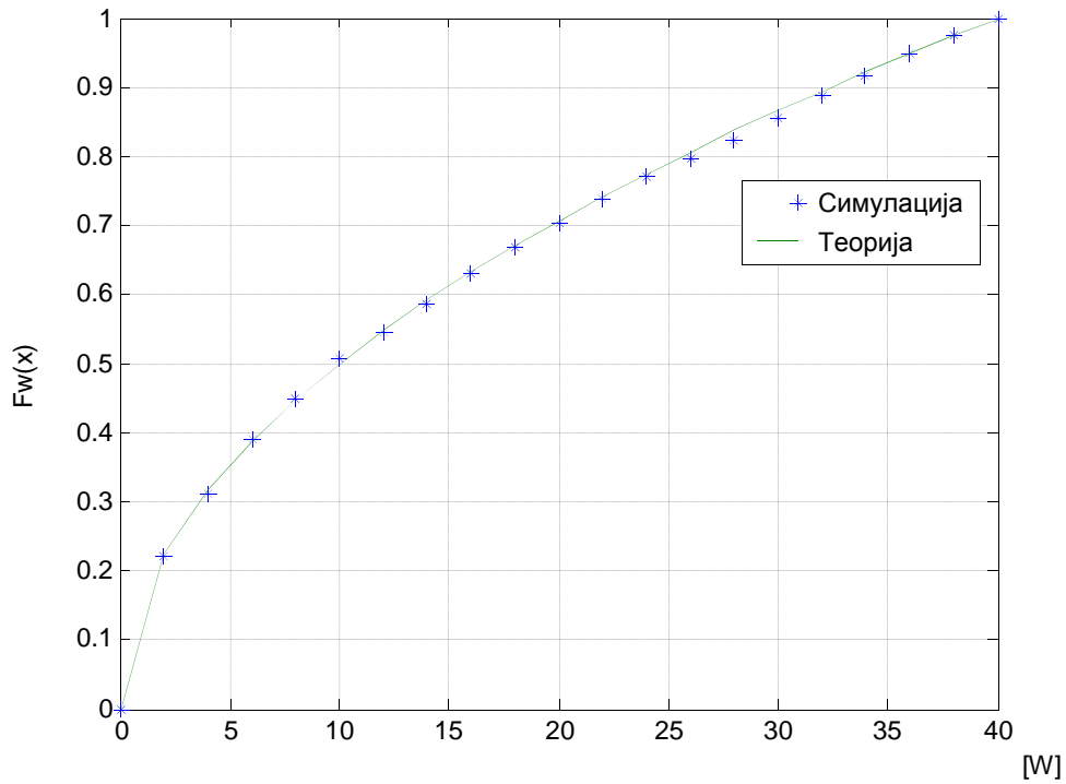
Сл. 6.5 CDF снаге једног канала за случај симулације и теоријског прорачуна ( N = 16, A = 10E, w_{max} = 40 W, R = 12 km, \gamma = 4 ).
