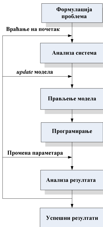
Сл. 4.1 Процес симулације.
