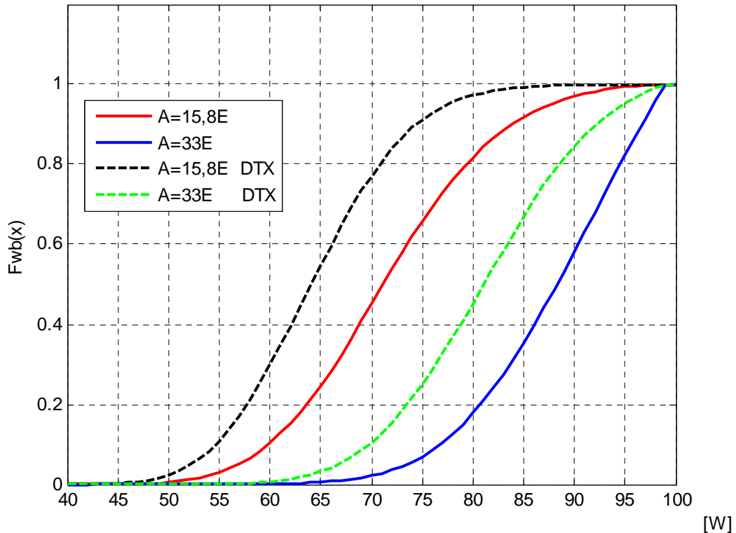
Сл. 6.37 CDF излазне снаге базе станице за мали број корисника ( N = 32 , M = 45 , w_{max} = 40 W , \alpha = 5 , \beta = 1 , R = 10 km , \gamma -линеарно растућа густина).
