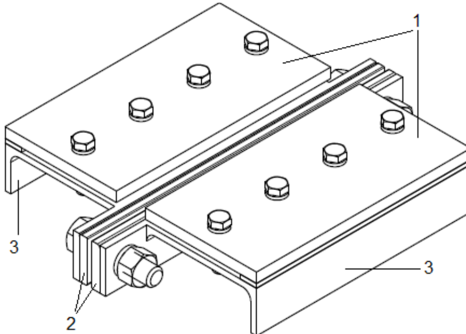
Слика 4.5 Конструкција стезног помоћног прибора коришћеног при заваривању Т-спојева од алуминијумске легуре 5052-Н32, 1-главне стезне плоче, 2-плоче са радијусима, 3- носачи
