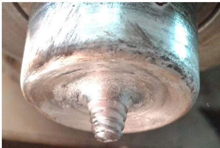
Слика 4.4 Фотографија алата на завршетку процеса заваривања
