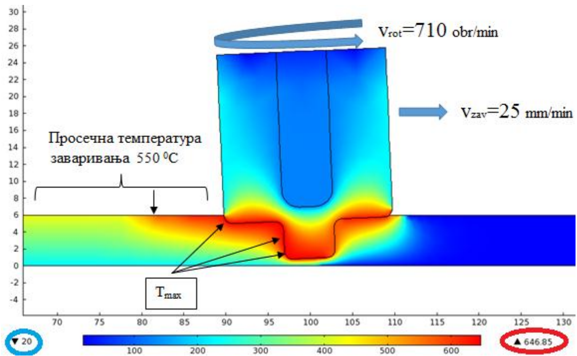
Слика 6.8 Метода коначних елемената коришћена за симулацију процеса ЗТМ.
