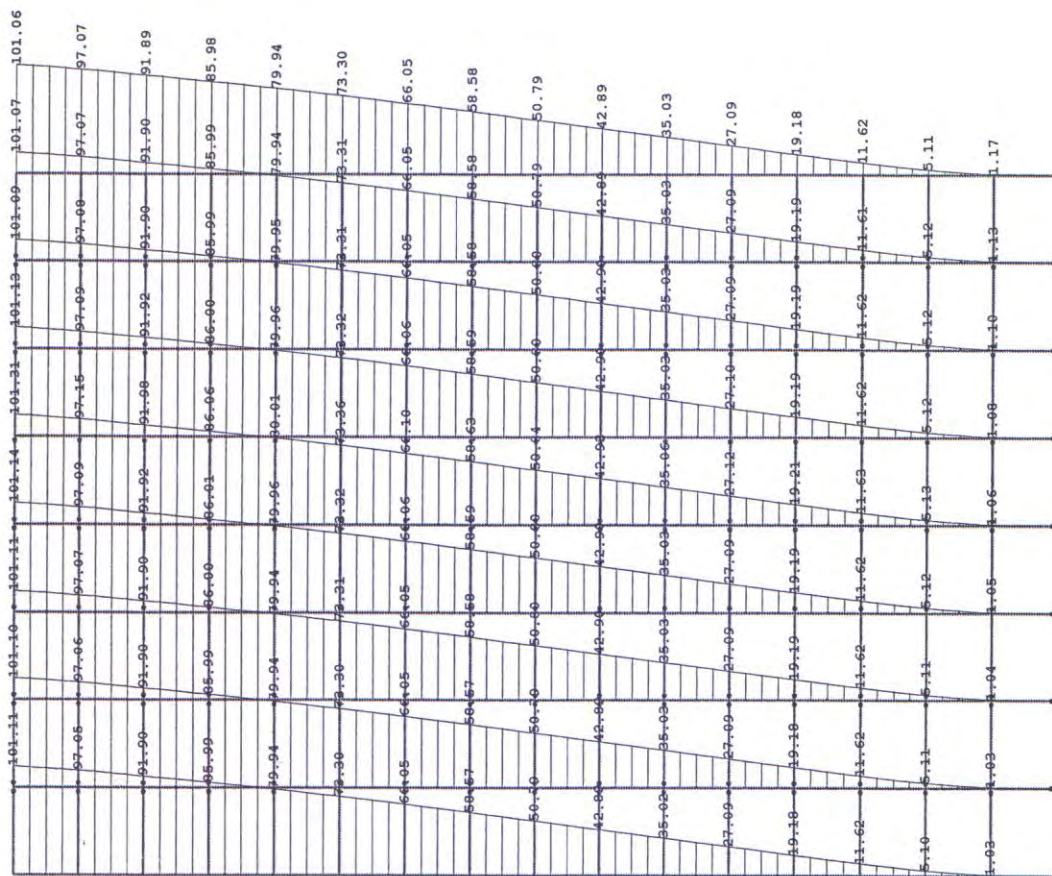
Model 9, Maksimalni horizontalni ugib u X-pravcu [mm]
