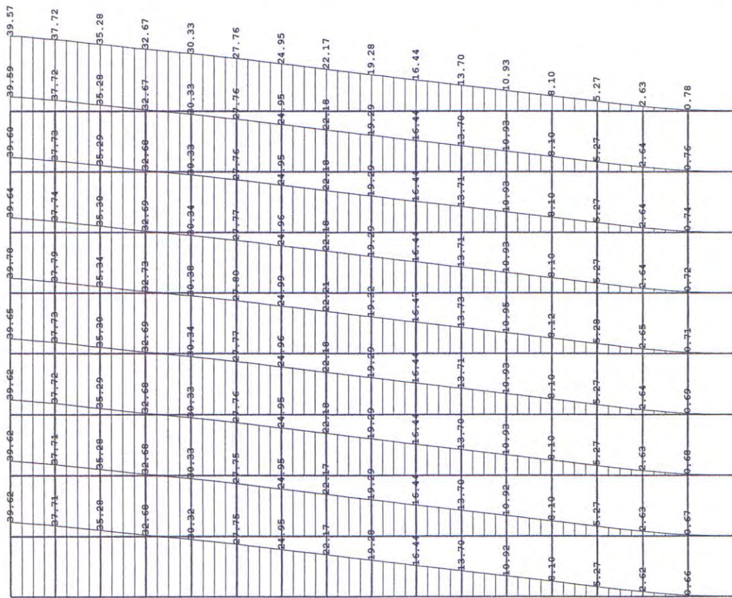
Model 1, Maksimalni horizontalni ugib u X-pravcu [mm]
