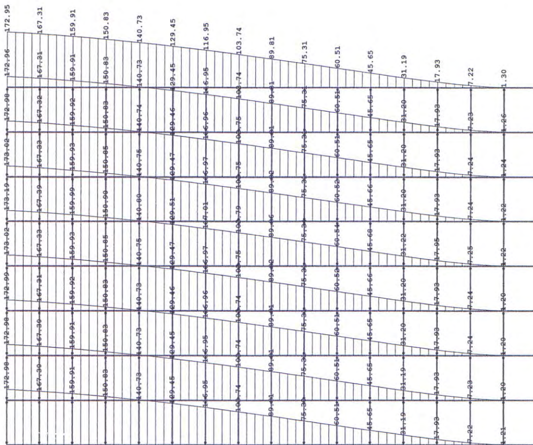
Model 13, Maksimalni horizontalni ugib u X-pravcu [mm]
