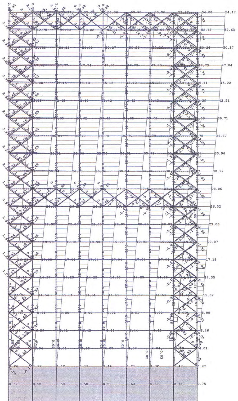
Model 2, Maksimalni horizontalni ugib u X-pravcu [mm]
