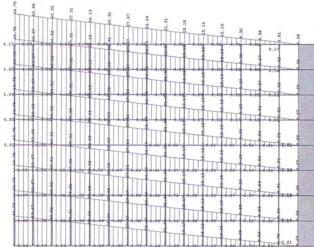
Model 12, Maksimalni horizontalni ugib u X-pravcu [mm]
