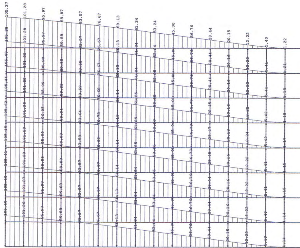
Model 10, Maksimalni horizontalni ugib u X-pravcu [mm]
