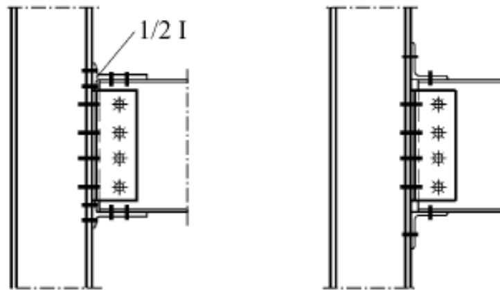
Slika 37 Momentne veze [44]
