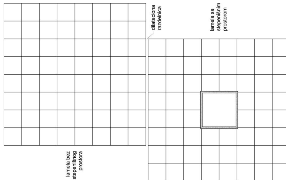
Slika 41 Lamelle zgrada odvojene dilatacionom razdelnicom
