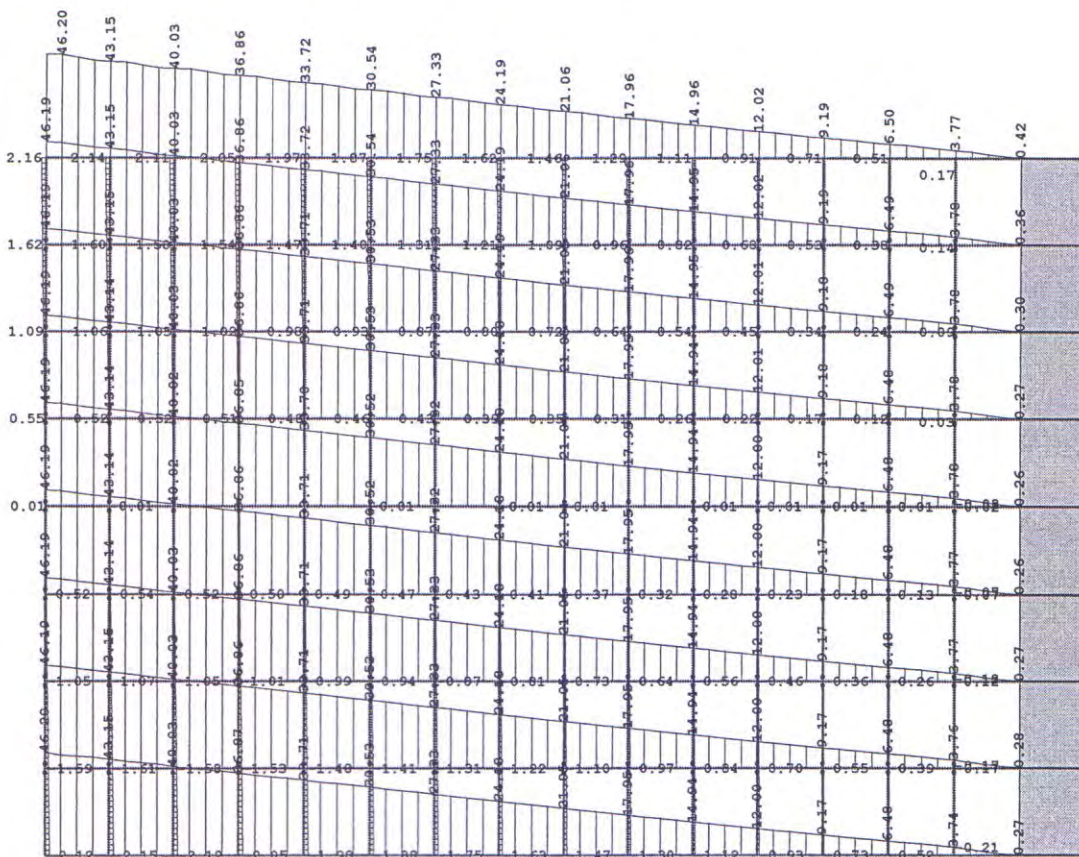
Model 11, Maksimalni horizontalni ugib u X-pravcu [mm]
