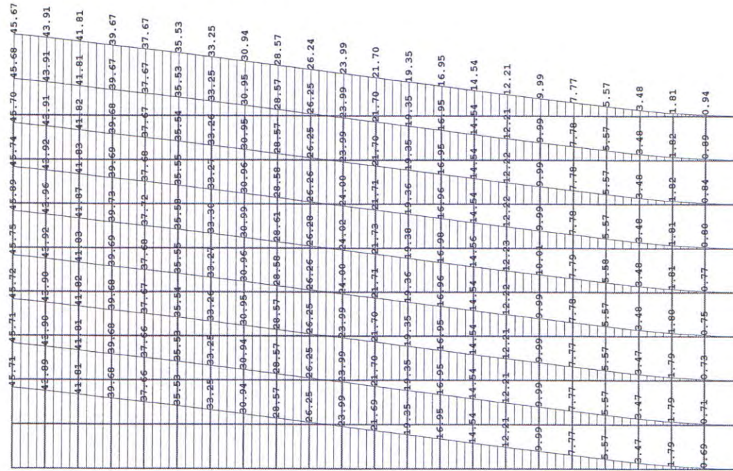
Model 2, Maksimalni horizontalni ugib u X-pravcu [mm]
