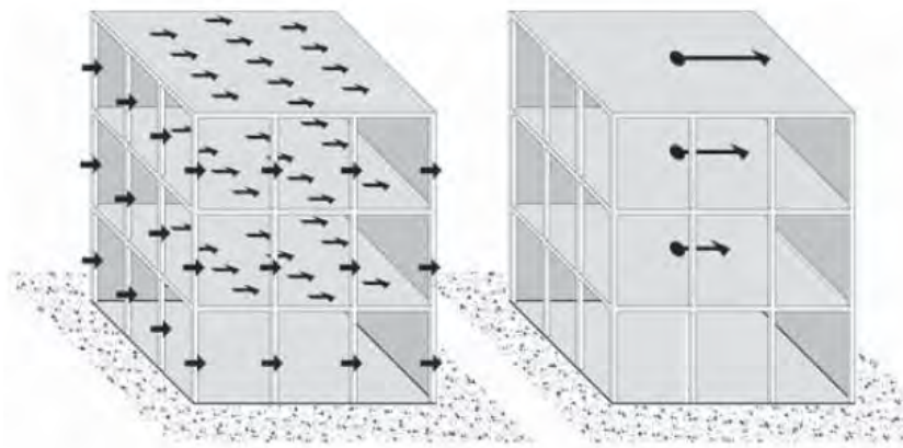
Slika 8 Dejstvo sila inercije u zgradi tokom zemljotresa [51]
