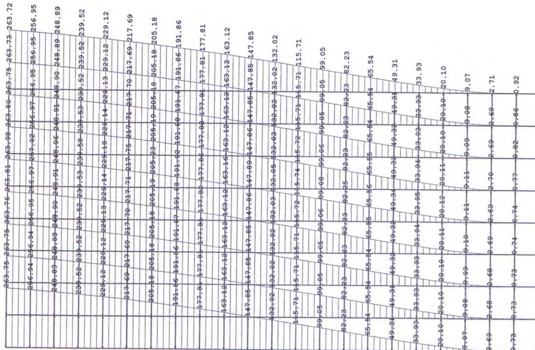
Model 12, Maksimalni horizontalni ugib u X-pravcu [mm]
