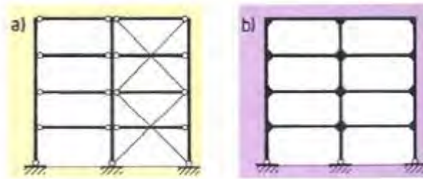
Slika 3 Skeletni noseći sistemi a) Zglobni b) Okvirni [49]
