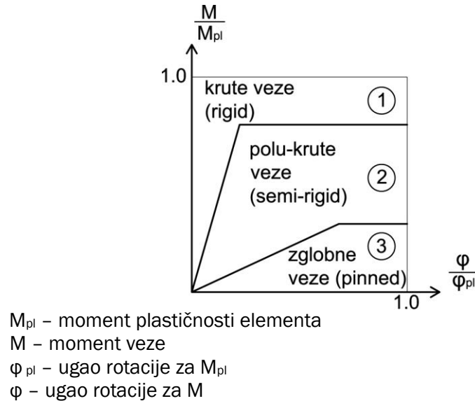
Slika 18 Podela veza
