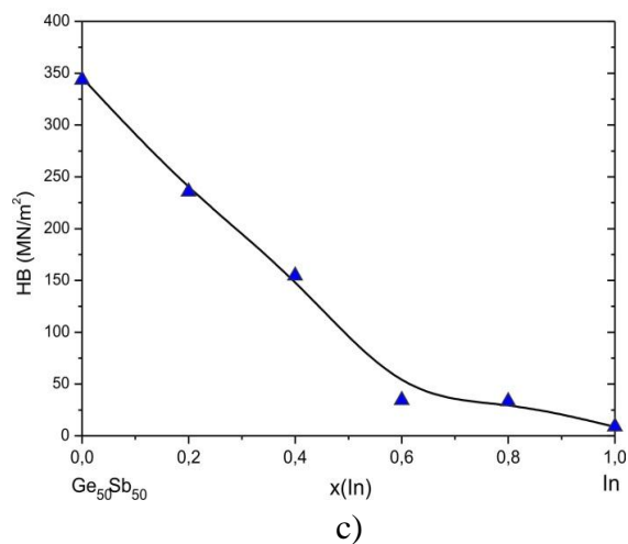
Slika 6.31. Tvrdoća po Brinelu za ispitivane uzorke sa izotermalnog preseka na 300\text{ }^\circ\text{C} : a) \text{Ge-In}_{50}\text{Sb}_{50} , b) \text{Sb-Ge}_{50}\text{In}_{50} i c) \text{In-Ge}_{50}\text{Sb}_{50} .
