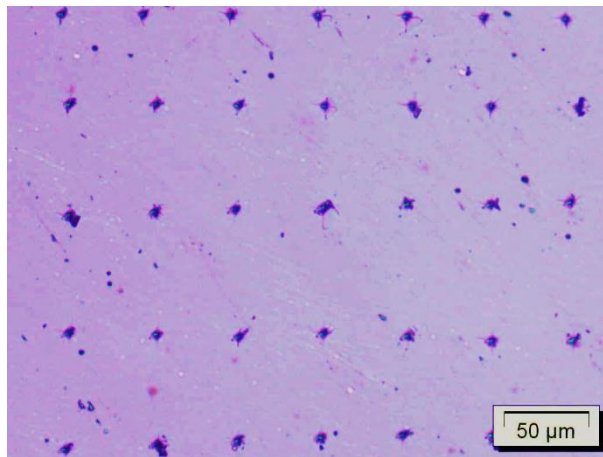
Slika 6.13. Mikrostruktura germanijuma posle merenja tvrdoće po Vickers metodi.
