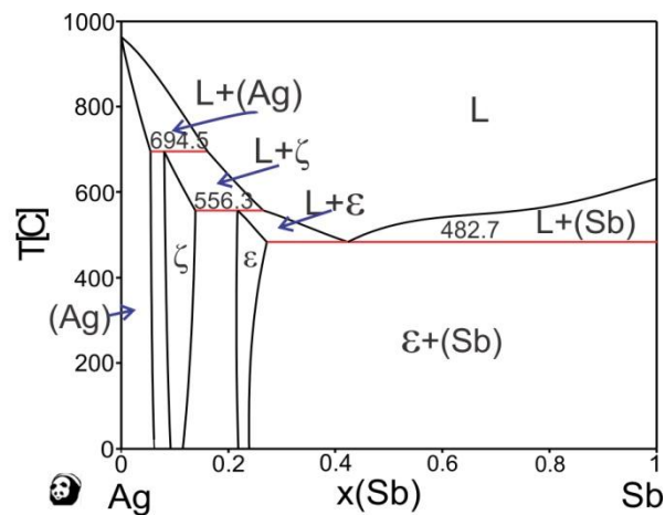
Slika 2.6. Proračunati ravnotežni dijagram stanja dvojnog Ag-Sb sistema po Zoro i saradnicima [78].
