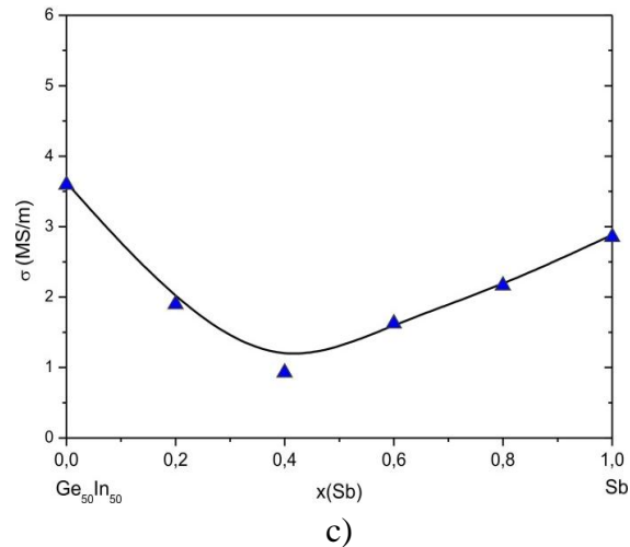
Slika 6.32. Elektroprovodljivost ispitivanih uzoraka iz izotermalnog preseka na 300 °C: a) Ge-In 50 Sb 50 , b) In-Ge 50 Sb 50 i c) Sb-Ge 50 In 50 .
