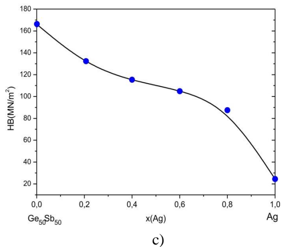
Slika 6.14. Tvrdoća po Brinelu za ispitivane uzorke sa izotermalnog preseka na 300 °C: a) Ge-Ag 50 Sb 50 , b) Sb-Ag 50 Ge 50 i c) Ag-Ge 50 Sb 50 .
