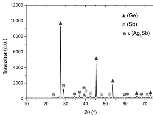
Slika 6.8. Difraktogram za uzorak 1 (Ag 37,33 Ge 29,03 Sb 33,64 (at. %)).
