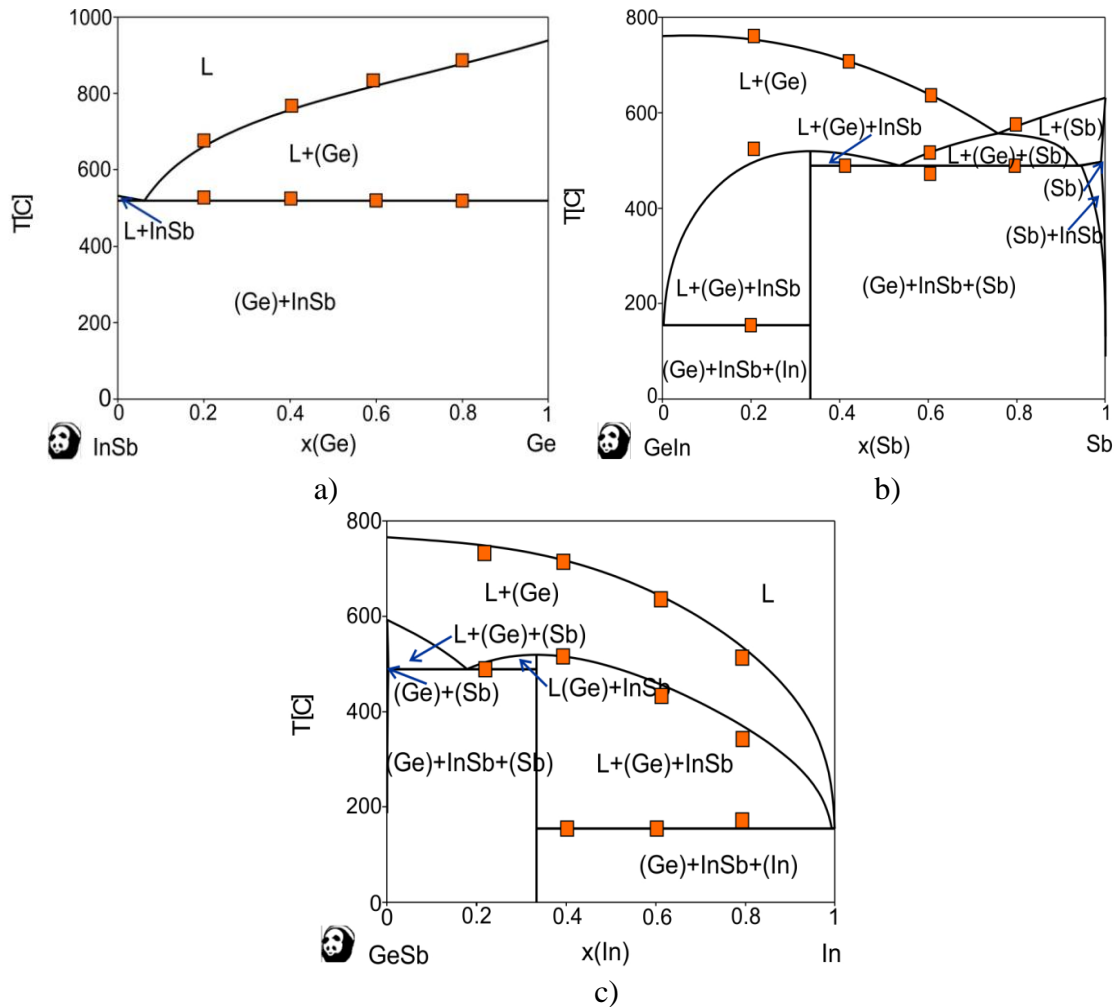
Slika 6.18. Predviđeni vertikalni preseći upoređeni sa DTA rezultatima iz ovog rada (narandasti kvadrat): a) Ge-InSb, b) Sb-InGe i c) In-GeSb.
