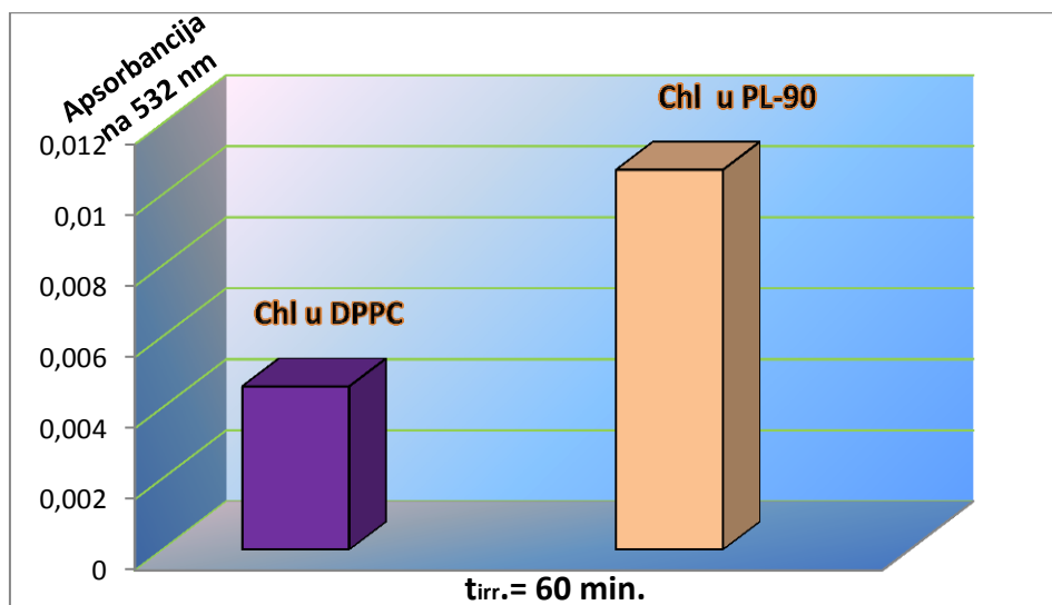
Slika 71. Razlika apsorbancije „kontrolne” i „uzorka” na 532 nm, dobijene TBA-MDA-testom za Chl-a-SUV-liposome pripremljene od DPPC-(levo) i PL-90-(desno) lipida. Iniciranje lipidne peroksidacije je vršeno (UV-B) ozračivanjem uzoraka u periodu od 60 min.
