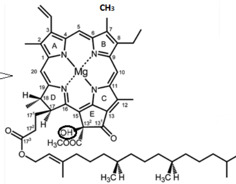
OH-Chla
