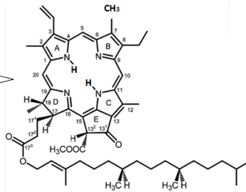
Pheoa
