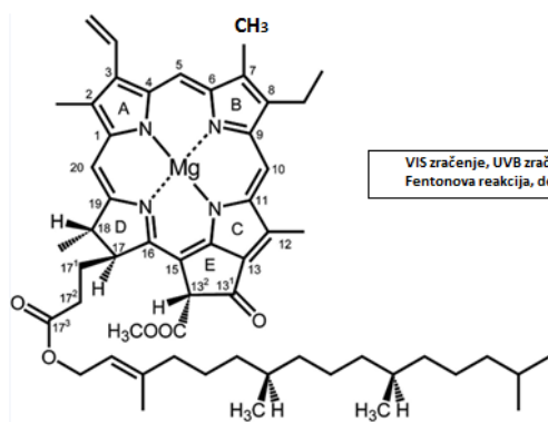
Chla
