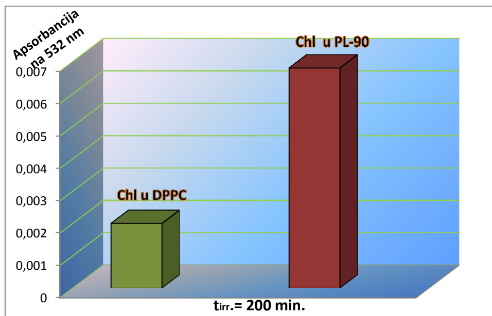
Slika 75. Promene apsorbancije „kontrolne” i uzorka (na 532 nm) dobijene TBA-MDA testom za hlorofile inkorporisane unutar SUV-DPPC i SUV-PL-90 lipozoma. Iniciranje lipidne peroksidacije je vršeno dejstvom vidljive svetlosti na uzorke, u trajanju od 200 min.
