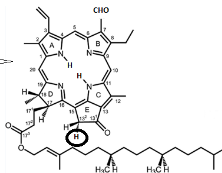
piroPheob
