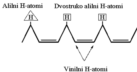
Slika 17. Raspored vinilnih, alilnih (trougao) i dvostruko alilnih (kvadrat) H-atoma u antikongjugovanoj strukturi nezasićene masne kiseline.
