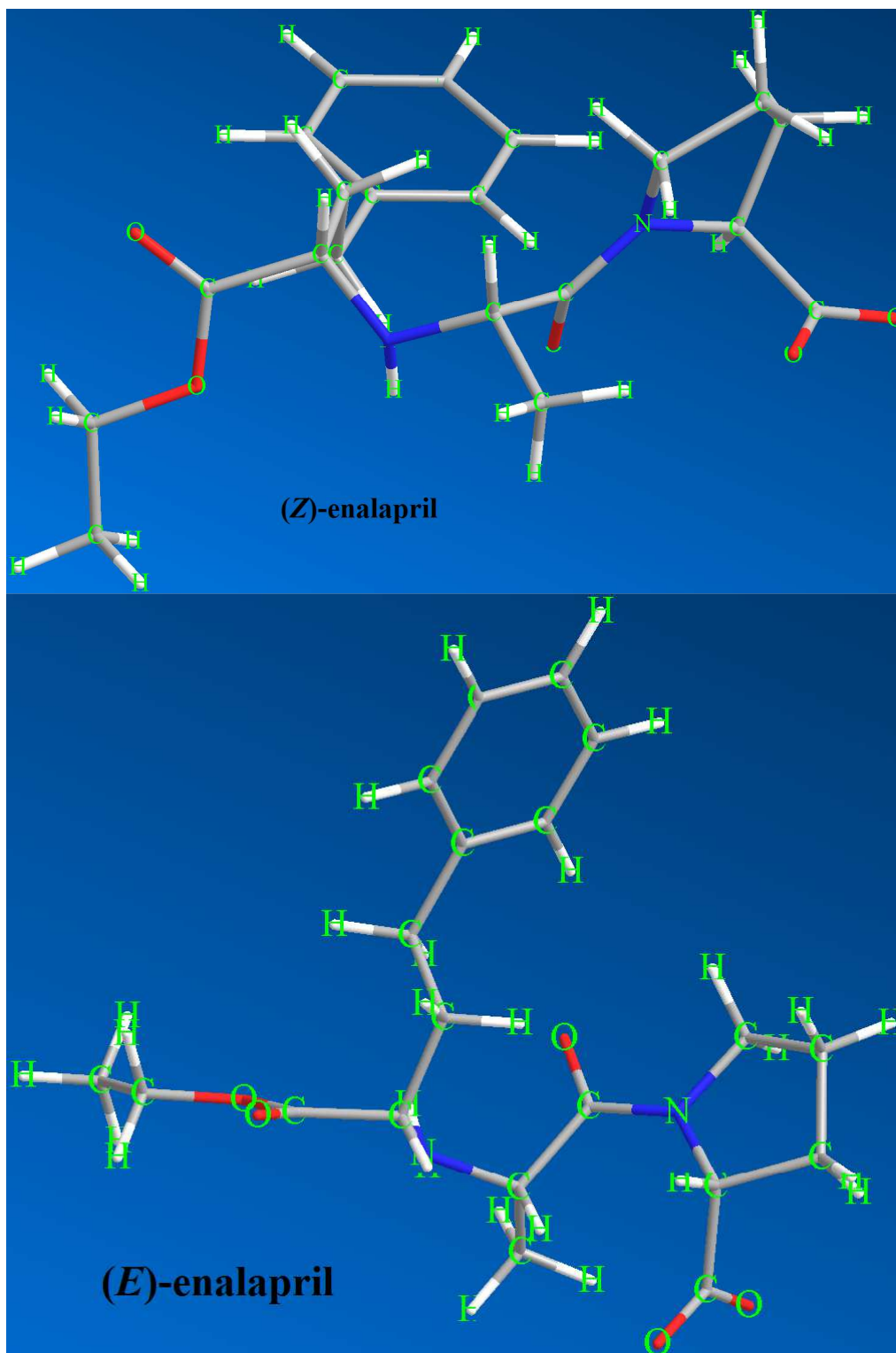
Slika 49. Geometrijski optimizovane strukture (Z)- i (E)-diastereoizomera enalaprila primenom B3LYP/6-31G (d,p) metoda u okviru Density Functional Theory (DFT), pomoću Gaussian 09 programa.
