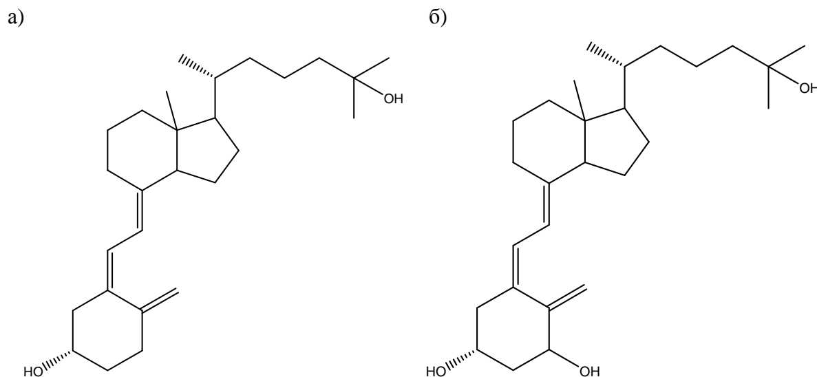
Слика 3. Хемијска структура а) 25-хидрокси витамина Д 3 и б) 1,25- дихидрокси витамина Д 3
