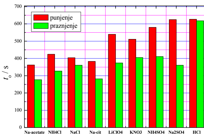
Слика 4.31. Однос времена пуњења и пражњења у првом циклусу.
