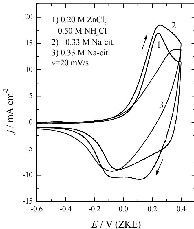
Слика 4.45. Циклични волтамограми ( 20 \text{ mV s}^{-1} ) електроде полианилина синтетисан са ( 0.6 \text{ mAh cm}^{-2} ) у 1) хлоридном, 2) хлоридно/цитратном и 3) цитратном електролиту
