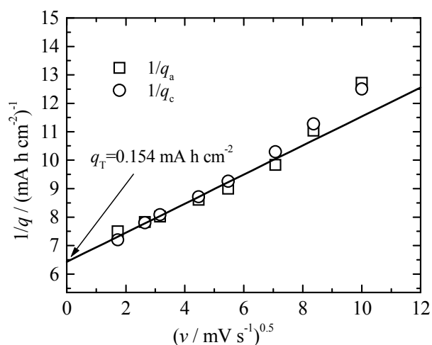
Слика 4.6. Зависност реципрочне вредности количине наелектрисања од квадратног корена брзине промене потенцијала
