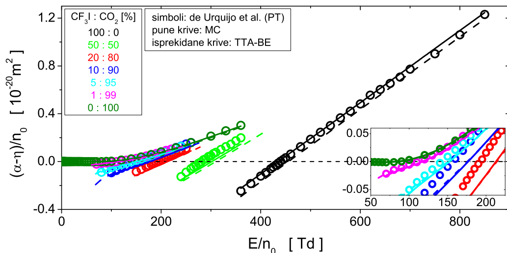
Slika 3.14: Efektivan koeficijent jonizacije u \text{CF}_3\text{I}-\text{CO}_2 smešama u funkciji E/n_0 . Poređenje eksperimentalnih vrednosti sa proračunima Monte Karlo simulacija i rešenjima Bolcmanove jednačine u aproksimaciji dva člana.
