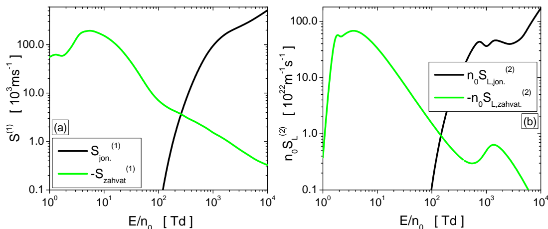
Slika 7.5: Koeficijenti prvog (panel (a)) i drugog reda (panel (b)) za zahvat elektrona i jonizaciju u razvoju izvornog člana transportne jednačine za elektrone u korigovanom modelu. Rezultati su dobijeni Monte Karlo simulacijama transporta elektrona u CF 3 I.
