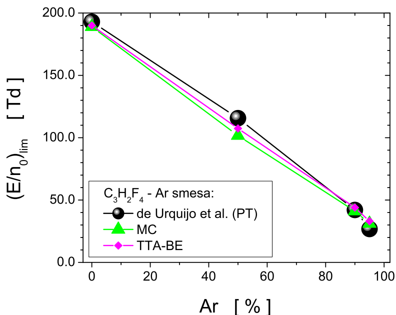
Slika 5.7: Kritično polje gasne smeše \text{C}_3\text{H}_2\text{F}_4 -Ar u funkciji koncentracije argona. Rezultati su dobijeni na osnovu eksperimentalnih i numerički izračunatih efektivnih koeficijenata jonizacije prikazanih na slici 5.6.
