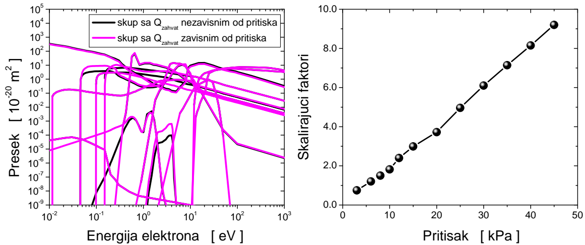
Slika 5.14: Poređenje skupova preseka za rasejanje elektrona u \text{C}_3\text{H}_2\text{F}_4 koji sadrže presek za zahvat elektrona nezavisan i zavisn od pritiska (a) i skalirajući faktori preseka za zahvat elektrona koji je zavisn od pritiska (b).
