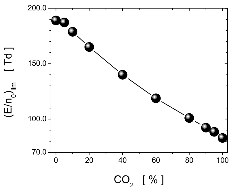
Slika 5.18: Kritično polje gasne smeše C_3H_2F_4 - CO_2 u funkciji koncentracije ugljen-dioksida. Rezultati su dobijeni na osnovu efektivnih koeficijenata jonizacije izračunatih Monte Karlo simulacijama.
