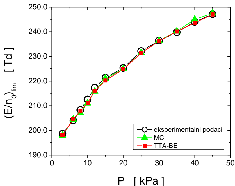
Slika 5.17: Kritično polje C_3H_2F_4 u funkciji pritiska gasa. Eksperimentalni podaci A. Čáčereua dobijeni u PT eksperimentu su upoređeni sa našim proračunima baziranim na Monte Karlo simulacijama i aproksimaciji dva člana za rešavanje Bolcmanove jednačine.
