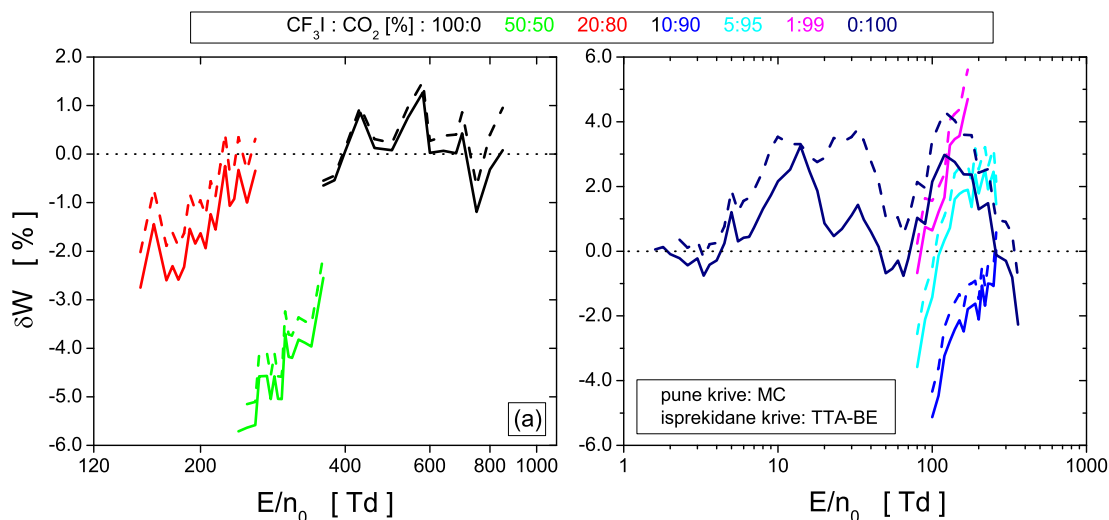
Slika 3.13: Procentualno odstupanje brzine drifta elektrona u CF 3 I-CO 2 smešama od eksperimentalnih podataka De Urkiha i saradnika izmerenih u PT eksperimentu. Proračuni su izvršeni na osnovu Monte Karlo rezultata i rešenja Bolcmanove jednačine u aproksimaciji dva člana. Panel (a) prikazuje rezultate u smešama sa koncentracijom CO 2 do 80%, dok panel (b) prikazuje rezultate u smešama sa većom koncentracijom CO 2 . Oznake krivih sa panela (b) se odnose i na panel (a).
