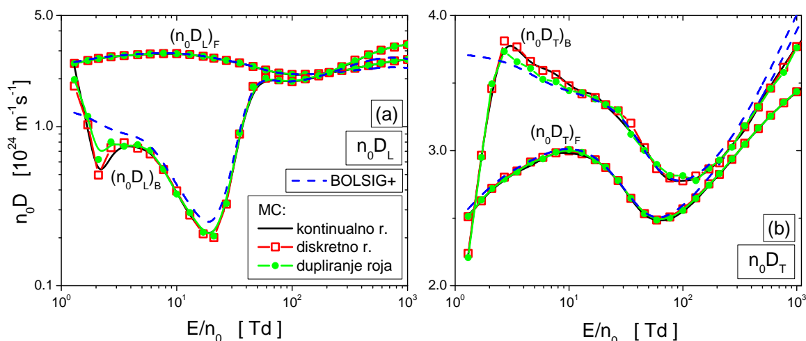
Slika 4.12: Promena longitudinalnog (a) i transverznog koeficijenta difuzije (b) za elektrone u SF 6 u funkciji E/n_0 . Rezultati su dobijeni Monte Karlo simulacijama sa razliĉitim tehnikama reskaliranja i upoređeni sa rezultatima koda BOLSIG+. Oznake krivih sa panela (a) odnose se i na panel (b).
