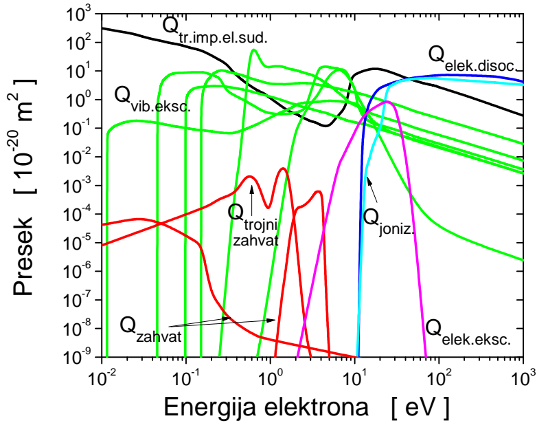
Slika 5.13: Skup preseka za rasejanje elektrona u C_3H_2F_4 koji sadrži presek za zahvat elektrona zavisian od pritiska. Skup sadrži: Q_{tr.imp.el.sud.} presek za transfer impulsa u elastičnim sudarima, šest Q_{vib.eksc.} preseka za vibracionu ekscitaciju, Q_{elek.eksc.} presek za elektronsku ekscitaciju, Q_{elek.disoc.} presek za elektronsku disocijaciju, dva Q_{zahvat} preseka za zahvat elektrona nezavisna od pritiska, Q_{trojni\ zahvat} presek za zahvat elektrona zavisian od pritiska i Q_{joniz.} presek za jonizaciju.
