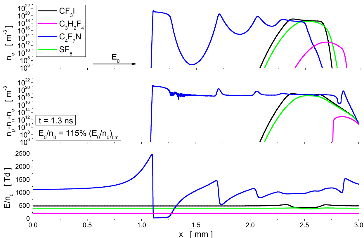
Slika 8.7: Propagacija negativnih strimera u \text{CF}_3\text{I} , \text{C}_3\text{H}_2\text{F}_4 , \text{C}_4\text{F}_7\text{N} i \text{SF}_6 pri spoljašnjim poljima koja su, za svaki gas, za 15% veća od kritičnog polja posmatranog gasa. Prikazani su rezultati korigovanog fluidnog modela u 1.5D konfiguraciji uz korišćenje transportnih koeficijenata elektrona izračunatih Monte Karlo simulacijama. Rezultati u vremenskom trenutku 1.3 ns. Oznake krivih sa gornjeg panela se odnose na sve panele.
