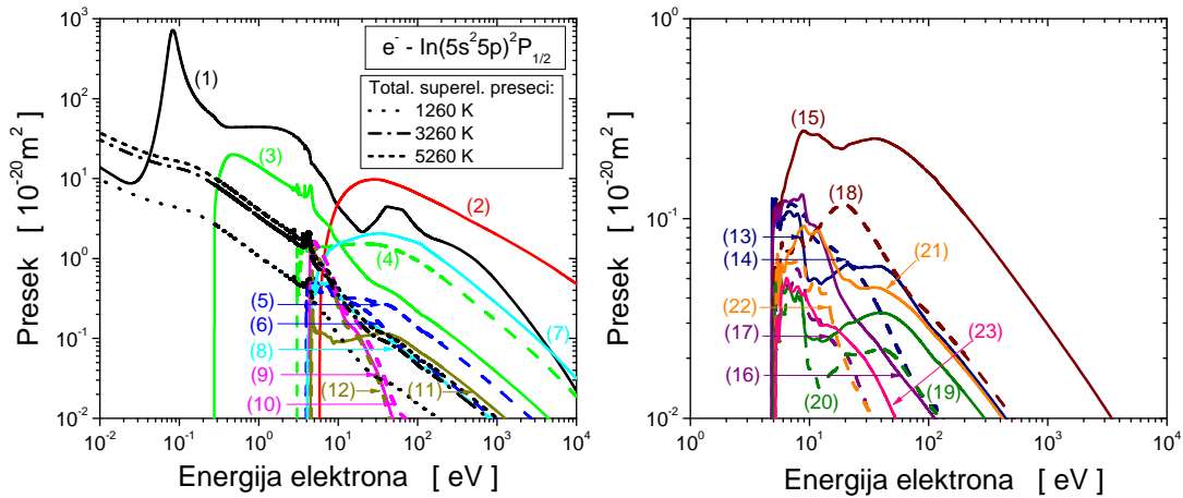
Slika 9.8: Integralni preseki za rasejanje elektrona u parama indijuma sa atomima na osnovnom nivou (5s^25p)^2P_{1/2} . Na levom panelu su prikazni preseki za transfer impulsa u elastičnim sudarima (1), totalnu jonizaciju (2) i veličina koje su dobijene množenjem totalnih preseka za superelastične sudare frakcionim populacijama osnovnog nivoa na temperaturi 1260 K, 3260 K odnosno 5260 K. Pored njih, prikazani su diskretni ekscitacioni prelazi sa osnovnog nivoa na nivo (5s^25p)^2P_{3/2} (3), (5s^26s)^2S_{1/2} (4), (5s^26p)^2P_{1/2} (5), (5s^26p)^2P_{3/2} (6), (5s^25d)^2D_{3/2} (7), (5s^25d)^2D_{5/2} (8), (5s^24p)^2P_{1/2} (9), (5s^24p)^2P_{3/2} (10), (5s^27s)^2S_{1/2} (11) i (5s^24p)^2P_{5/2} (12). Na desnom panelu su prikazani diskretni ekscitacioni prelazi sa sa osnovnog nivoa na nivo (5s^27s)^2P_{1/2} (13), (5s^27s)^2P_{3/2} (14), (5p^26d)^2D_{3/2} (15), (5p^26d)^2D_{5/2} (16), (5p^24f)^2F_{7/2} (17), (5p^24f)^2F_{5/2} (18), (5p^28s)^2S_{1/2} (19), (5p^28s)^2P_{1/2} (20), (5s^27d)^2D_{3/2} (21), (5s^27d)^2D_{5/2} (22) i (5s^28p)^2P_{3/2} (23).
