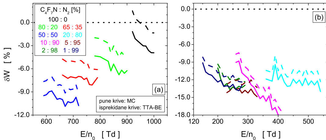
Slika 6.10: Procentualno odstupanje brzine drifta elektrona u C_4F_7N-N_2 smešama od eksperimentalnih podataka De Urkiha i saradnika izmerenih u PT eksperimentu. Proračuni su izvršeni na osnovu Monte Karlo simulacija i rešavanja Bolcmanove jednačine u aproksimaciji dva člana. Panel (a) prikazuje rezultate u smešama sa koncentracijom N_2 do 50% dok panel (b) prikazuje rezultate u smešama sa većom koncentracijom N_2 . Oznake krivih sa panela (a) se odnose i na panel (b).
