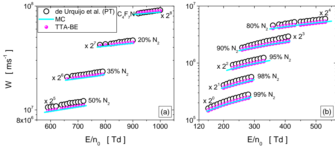
Slika 6.9: Brzina drifta elektrona u C_4F_7N-N_2 smešama u funkciji E/n_0 . Poređenje eksperimentalnih vrednosti sa rezultatima Monte Karlo simulacija i rešenjima Bolcmanove jednačine u aproksimaciji dva člana. Panel (a) prikazuje rezultate u smešama sa koncentracijom N_2 do 50% dok panel (b) prikazuje rezultate u smešama sa većom koncentracijom N_2 . Oznake krivih sa panela (a) se odnose i na panel (b). Radi preglednosti, rezultati su skalirani faktorom 2^n .
