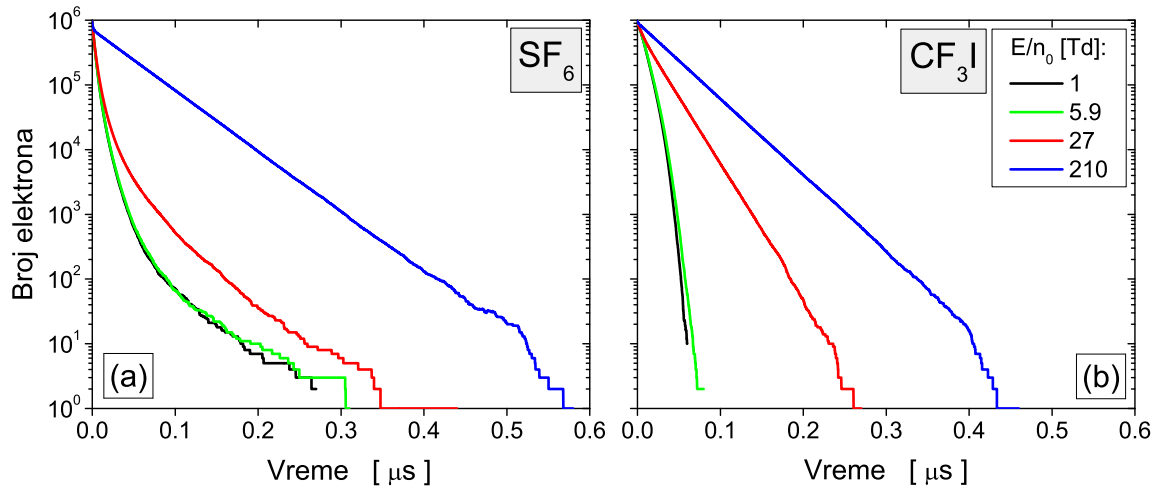
Slika 4.2: Opadanje broja elektrona u funkciji vremena u SF 6 (a) i CF 3 I (b). Rezultati su dobijeni Monte Karlo simulacijama na različitim vrednostima spoljašnjeg redukovanog električnog polja su dobijeni bez primene tehnika reskaliranja elektrona. Oznake krivih sa panela (b) se odnose i na panle (a).
