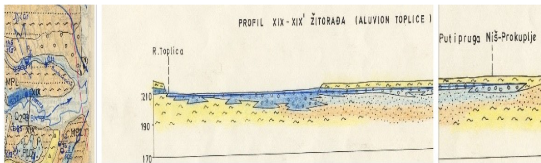
Слика 7. Локација и карактеристике хидрогеолошког профила Житорађа (Модификовано према извору: Хидрогеолошка карта слива Јужне Мораве 1:200000).
