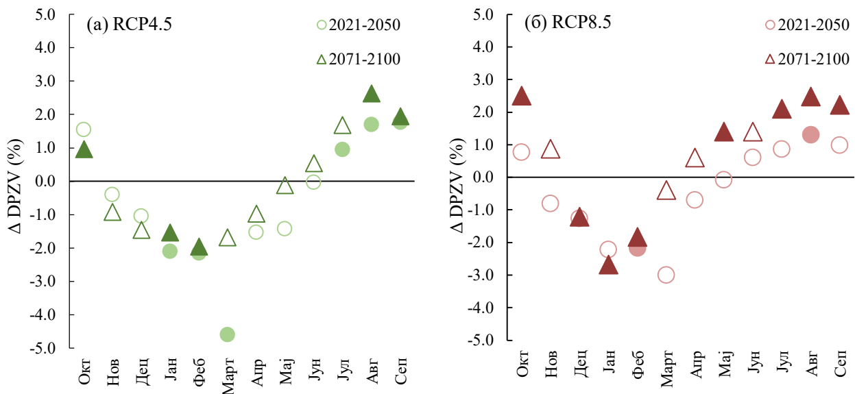
Слика 33. Унутаргодишња расподела релативног одступања медијане дубине подземне воде (DPZV) у блиској и далекој будућности по RCP4.5 (а) и RCP8.5 (б), у односу на референтни период. Испуњене ознаке означавају статистички значајну промену према Mann-Whitney тесту ( p=0,05 ).
