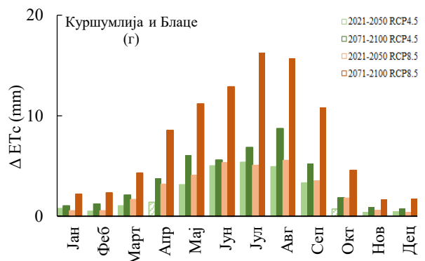
Слика 46. Потребне за водом (ET c ) за детелину у референтном и будућим периодима и промена (Δ ET c ) у односу на референтни период по месецима за подручје Прокупље и Житорађа (а) и (в) и Куршумлија и Блаце (б) и (г). Испуњени полигони ((в) и (г)) означавају статистички значајну промену према Mann-Whitney тесту (p=0,05).
