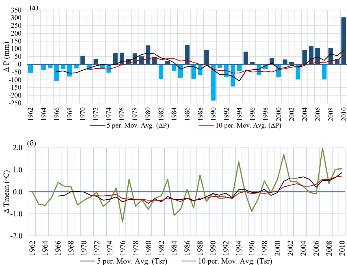
Слика 17. Одступање од нормале пондерисане годишње суме падавина (P) (a) и средње годишње температуре ( T_{mean} ) (b) на подручју слива реке Топлице и 5-годишњи и 10-годишњи покретни просек, период 1961-2010. година.
