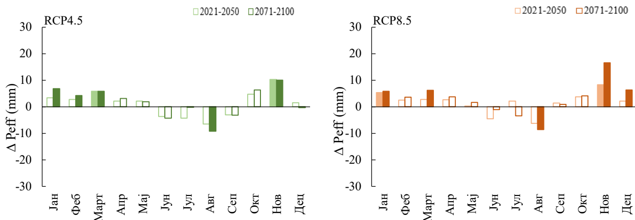
Слика 40. Промена медијане ефективних падавина ( P_{\text{eff}} ) у односу на референтни период, метеоролошка станица Прокупље. Испуњени полигони означавају статистички значајну промену према Mann-Whitney тесту ( p=0,05 ).
