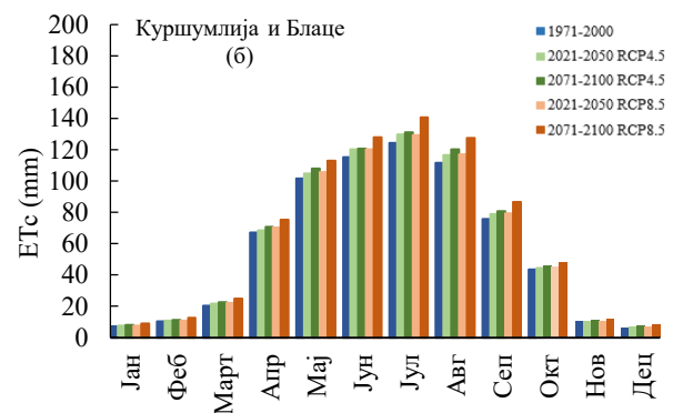
Слика 45. Потребне за водом (ET c ) за луцерку у референтном и будућим периодима и промена (Δ ET c ) у односу на референтни период по месецима за подручје Прокупље и Житорађа (а) и (в) и Куршумлија и Блаце (б) и (г). Испуњени полигони ((в) и (г)) означавају статистички значајну промену према Mann-Whitney тесту (p=0,05).
