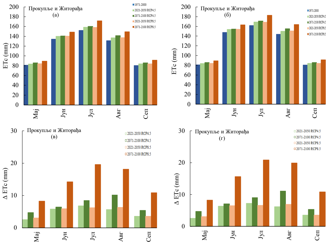
Слика 53. Потребне за водом (ETc) у референтном и будућим периодима и промена ( \Delta ETc) у односу на референтни период по месецима за паприку (а) и (в) и парадајз (б) и (г) за подручје Прокупље и Житорађа. Испуњени полигони ((в) и (г)) означавају статистички значајну промену према Mann-Whitney тесту ( p=0,05 ).
