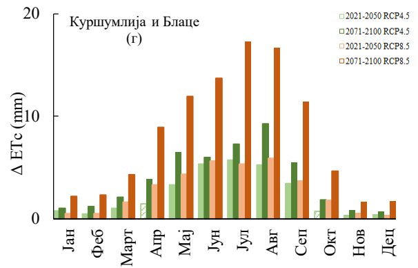
Слика 45. Потребне за водом (ET c ) за луцерку у референтном и будућим периодима и промена (Δ ET c ) у односу на референтни период по месецима за подручје Прокупље и Житорађа (а) и (в) и Куршумлија и Блаце (б) и (г). Испуњени полигони ((в) и (г)) означавају статистички значајну промену према Mann-Whitney тесту (p=0,05).
