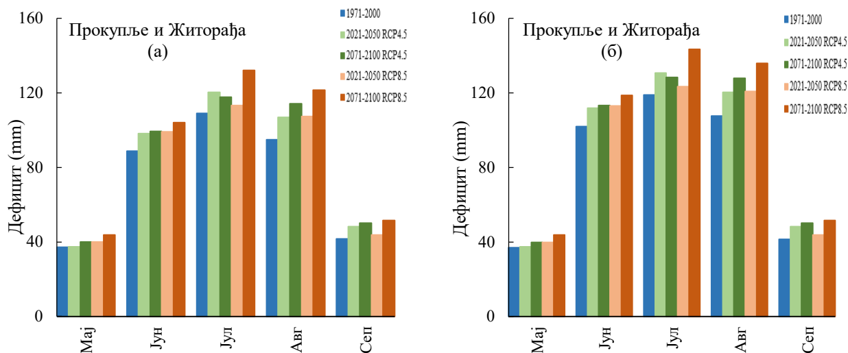
Слика 77. Дефицит воде за паприку (а) и парадајз (б) у референтном и будућим периодима, за подручје Прокупље и Житорађа.
