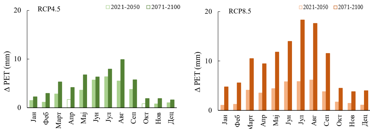
Слика 36. Промена медијане потенцијалне евапотранспирације (РЕТ) у односу на референтни период, метеоролошка станица Прокупље. Испуњени полигони означавају статистички значајну промену према Mann-Whitney тесту ( p=0,05 ).
