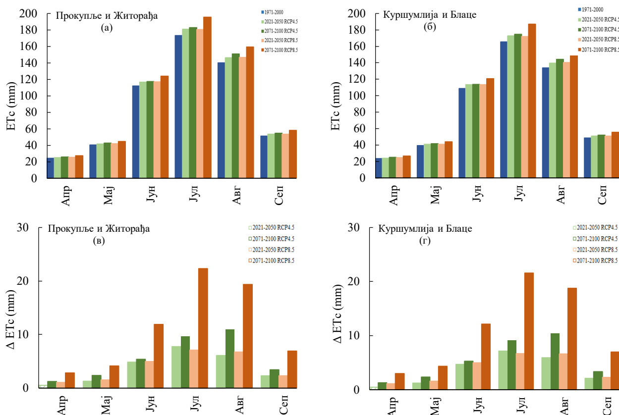
Слика 43. Потребне за водом (ЕТс) за кукуруз у референтном и будућим периодима и промена ( \Delta \text{ETc} ) у односу на референтни период по месецима за подручје Прокупље и Житорађа (а) и (в) и Куршумлија и Блаце (б) и (г). Испуњени полигони ((в) и (г)) означавају статистички значајну промену према Mann-Whitney тесту ( p=0,05 ).
