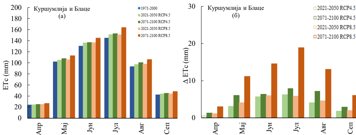
Слика 49. Потребне за водом (ETc) за малину у референтном и будућим периодима (а) и промена ( \Delta ETc) у односу на референтни период по месецима (б) за подручје Куршумлија и Блаце. Испуњени полигони (б) означавају статистички значајну промену према Mann-Whitney тесту ( p=0,05 ).
