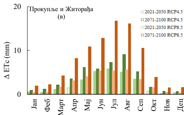
Слика 46. Потребне за водом (ET c ) за детелину у референтном и будућим периодима и промена (Δ ET c ) у односу на референтни период по месецима за подручје Прокупље и Житорађа (а) и (в) и Куршумлија и Блаце (б) и (г). Испуњени полигони ((в) и (г)) означавају статистички значајну промену према Mann-Whitney тесту (p=0,05).
