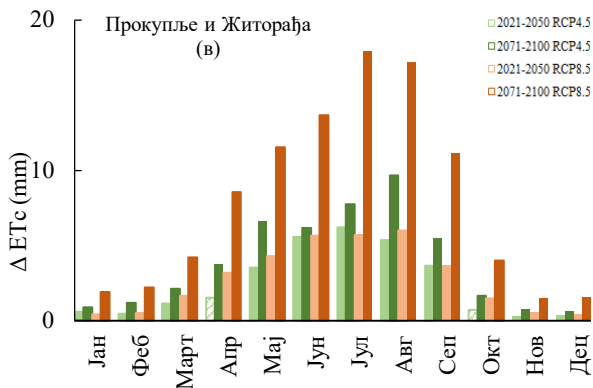
Слика 45. Потребне за водом (ET c ) за луцерку у референтном и будућим периодима и промена (Δ ET c ) у односу на референтни период по месецима за подручје Прокупље и Житорађа (а) и (в) и Куршумлија и Блаце (б) и (г). Испуњени полигони ((в) и (г)) означавају статистички значајну промену према Mann-Whitney тесту (p=0,05).
