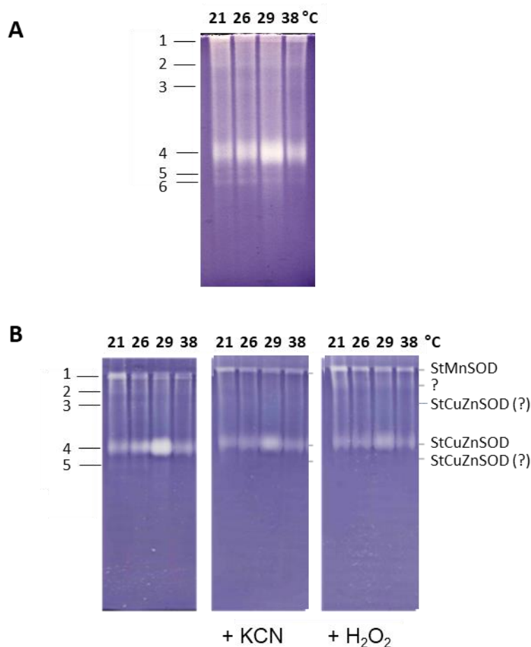
Slika 35. Esej aktivnosti StSOD izolovanih iz listova in vitro gajenih biljaka sorte Désirée. Biljke su izložene temperaturama od 21 °C, 26 °C, 29 °C u trajanju od tri nedelje, ili 38 °C tokom 4 h. ( A ) Aktivnost svih StSOD. ( B ) Identifikacija različitih StSOD korišćenjem selektivnih inhibitora KCN (3 mM) i H 2 O 2 (3 mM).
