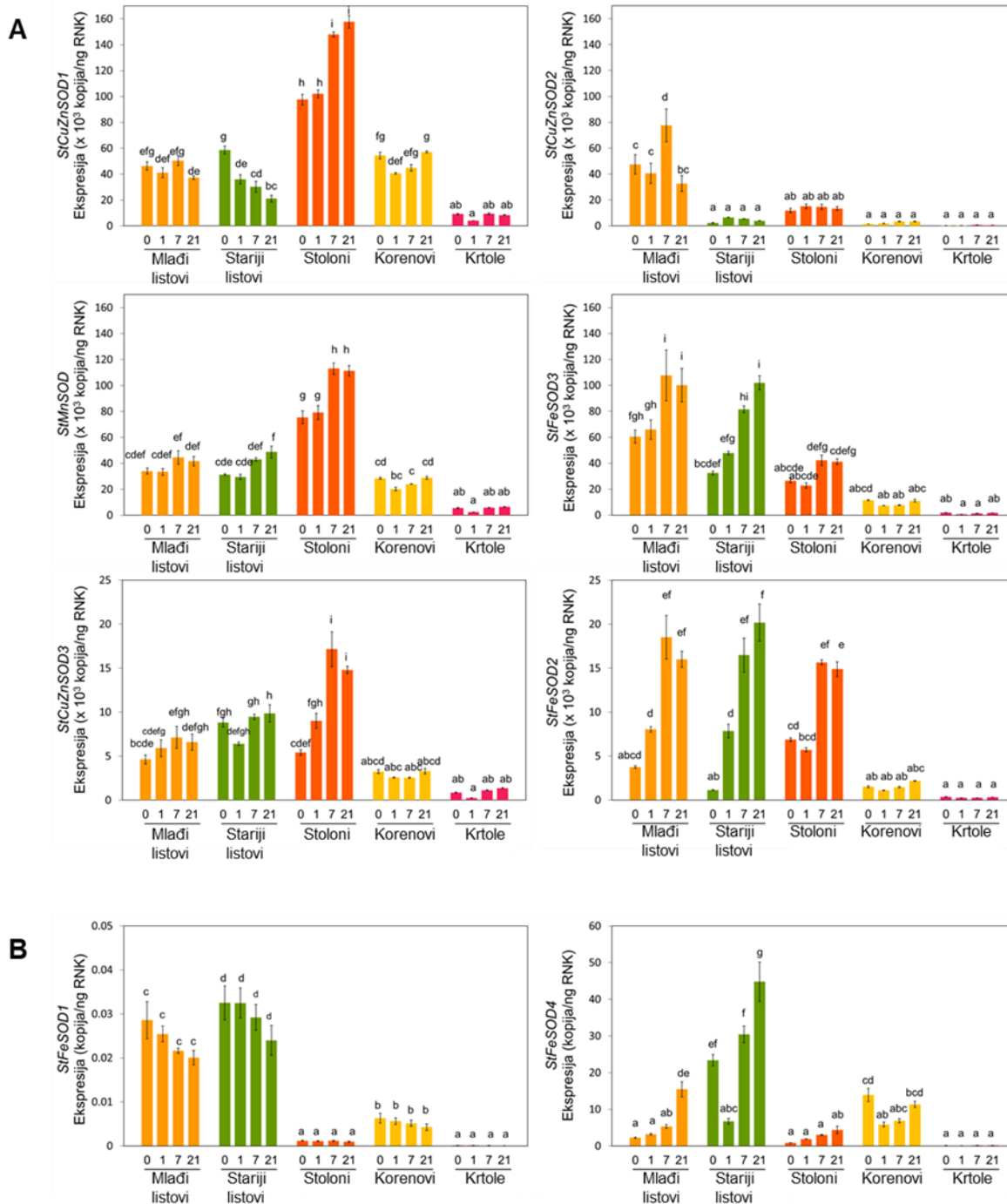
Slika 47. Apsolutni broj kopija transkripata visoko (A) i nisko (B) ekspimiranih StSOD gena u različitim organima sorte Désirée gajene ex vitro tokom dugotrajnog tretmana visokom temperaturom (30/20 °C, dan/noć). Efekat temperature praćen je u četiri vremenske tačke: (0) dan pre tretmana visokom temperaturom, (1) prvi dan, (7) sedmi dan i (21) 21. dan tretmana visokom temperaturom. Apsolutne vrednosti broja transkripata su normalizovane prema kontrolnim genima ( 60SL36 i CYC ). Rezultati na graficima predstavljaju srednje vrednosti tri tehnička ponavljanja \pm standardna greška.
