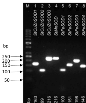
Slika 32. Provera specifičnosti prajmera ispitivanih StSOD gena i određivanje veličine dobijenih amplikona. M, DNK marker; bp, bazni parovi.
