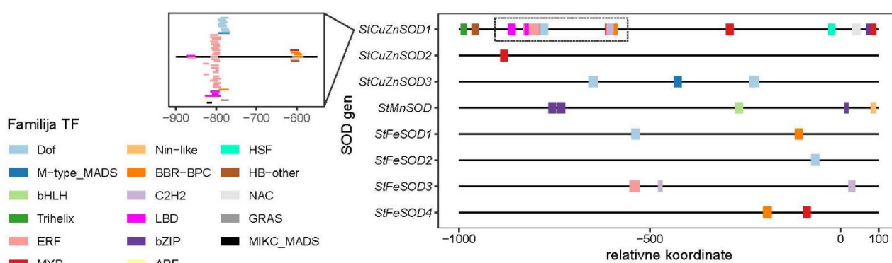
Slika 21. Pretpostavljena mesta vezivanja TF iz različitih familija za promotore StSOD gena. In silico analizom je obuhvaćen region od 100 nukleotida nizvodno i 1000 nukleotida uzvodno od mesta početka transkripcije. TF, transkripcioni faktori. Preuzeto i modifikovano prema Rudić i sar. (2022a).
