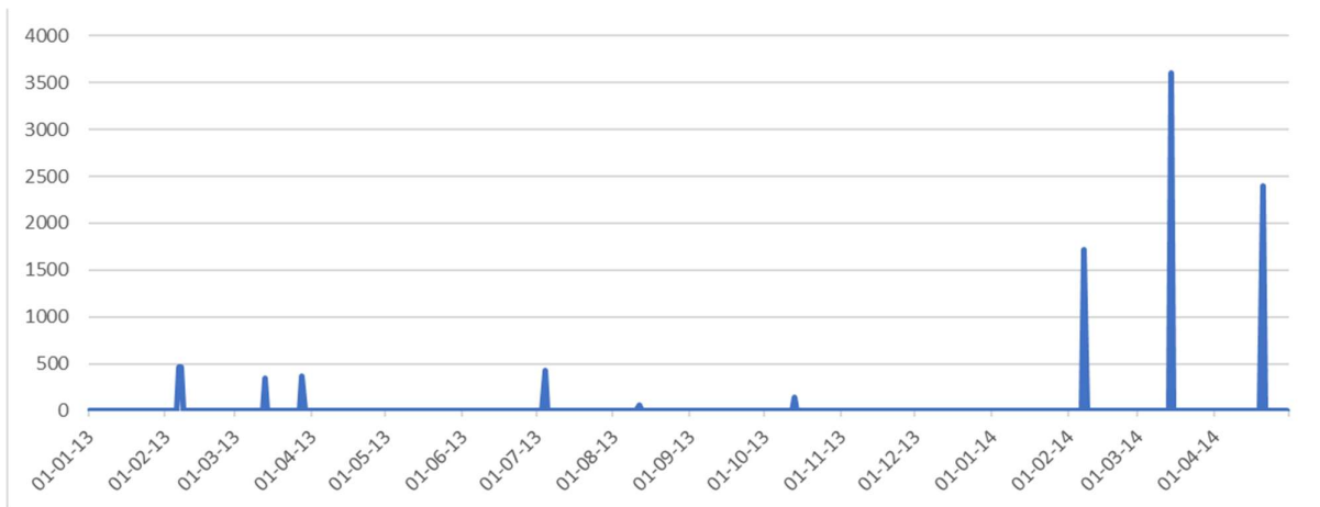
Слика 10 - GDELT догађаји растресити (Украјина)
