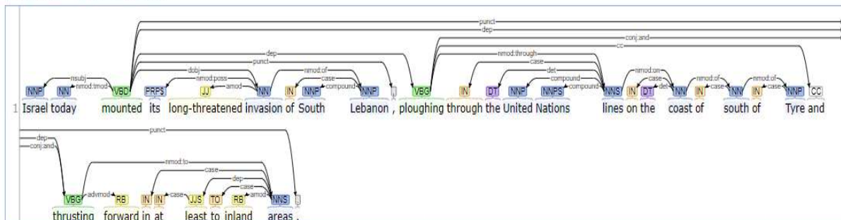
Слика 8 – Пример савременог система за аутоматско процесирање текста Универзитета Стенфорд
