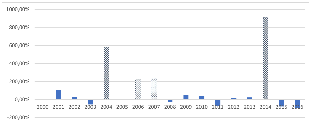
Слика 40 – Промена учесталости секуритизујућих потеза (Украјина). Године које је карактерисала изражена политичка криза обележене су шрафираним ступцима.
