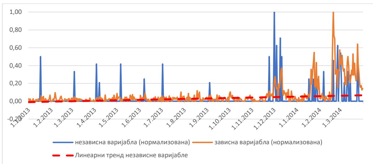
Слика 45 - Однос независне и зависне варијабле на примеру секуритизујућих потеза власти према опозицији
