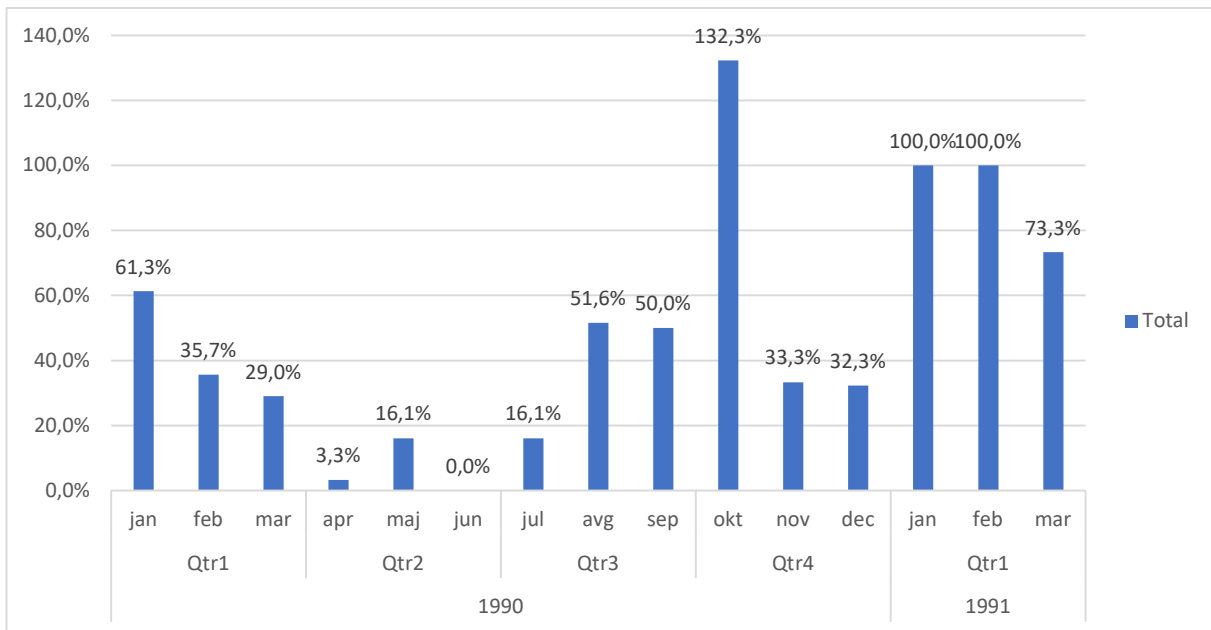
Слика 23 - Просечна површина насловне стране коју су заузимали секуритизујући потези на месечном нивоу (Вечерњи лист)
