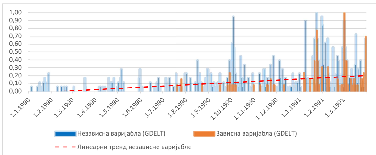
Слика 36 - Однос нормализованих вредности машински генерисане независне и зависне варијабле
