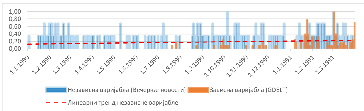
Слика 35 - Однос ручно кодиране независне и машински генерисане зависне варијабле (Вечерње новости)
