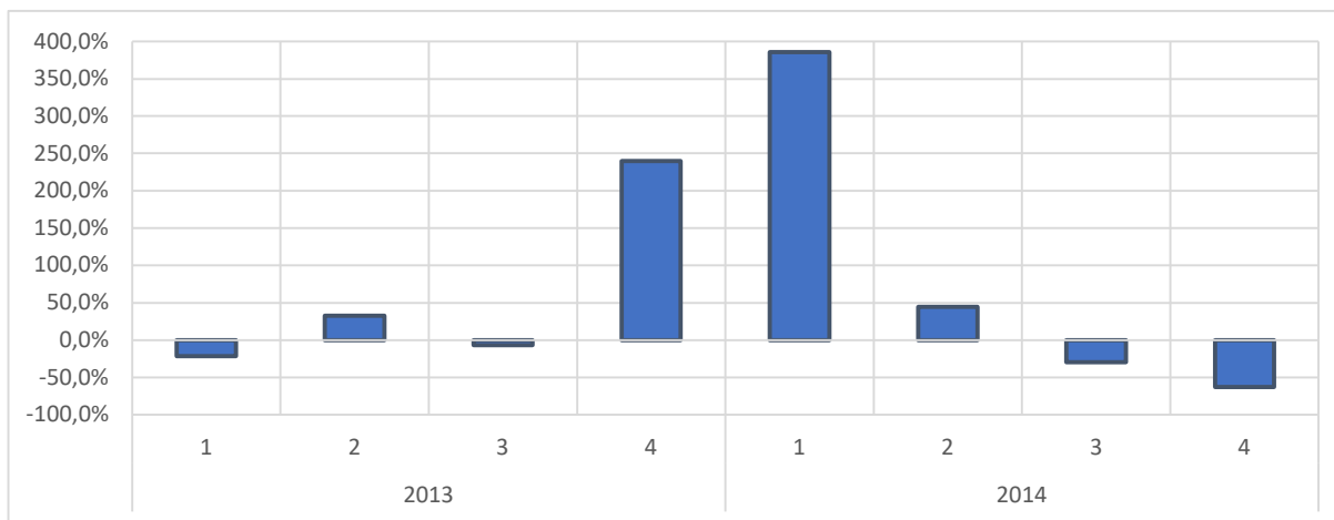
Слика 41 – Процентуална промена броја регистрованих секуритизујућих потеза (Украјина)
