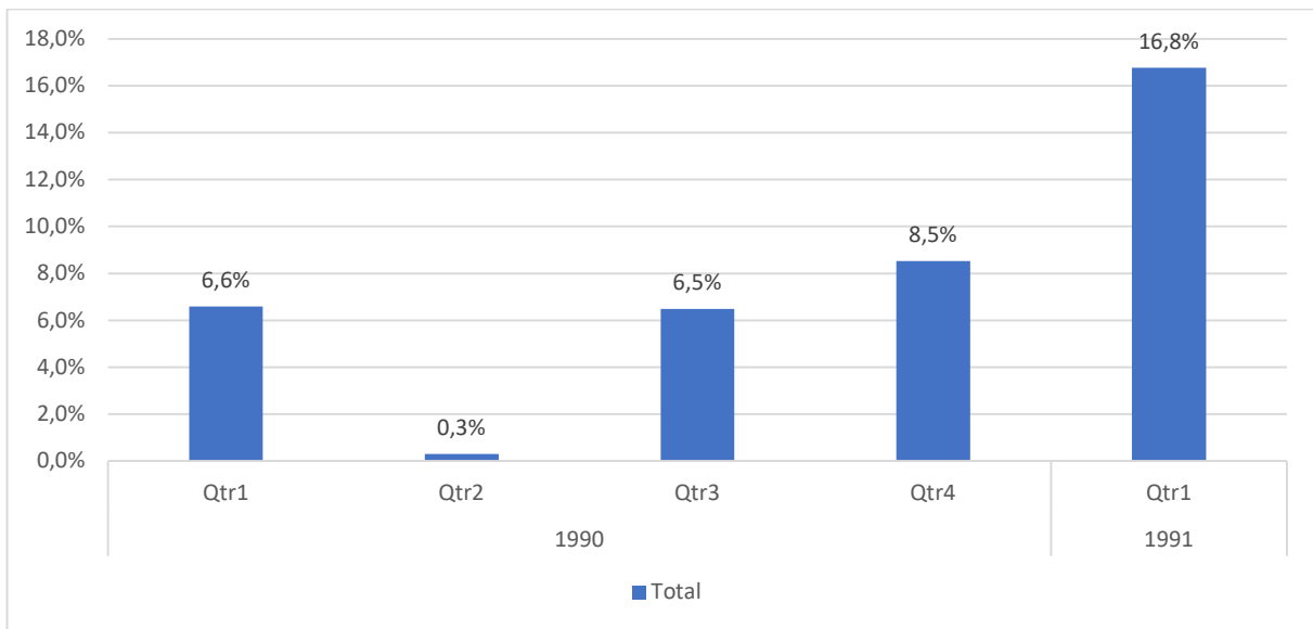
Слика 22 - Просечна површина насловне стране коју су заузимали секуритизујући потези на кварталном нивоу (Вечерњи лист)
