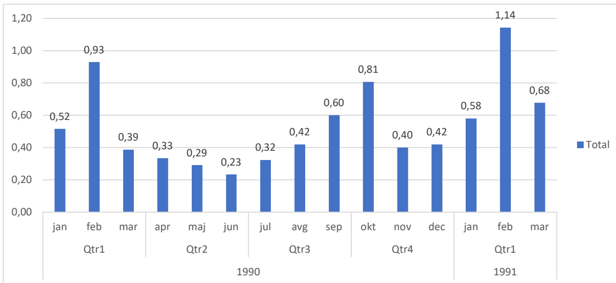
Слика 26 - Просечни број секуритизујућих потеза по дану за сваки месец (Вечерње новости)
