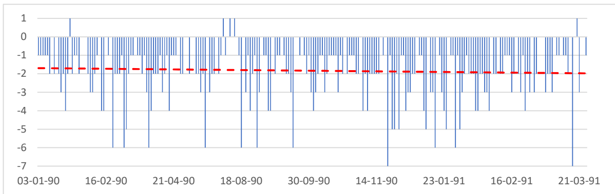
Слика 38 - Сентимент секуритизујућих потеза у Вечерњим новостима
