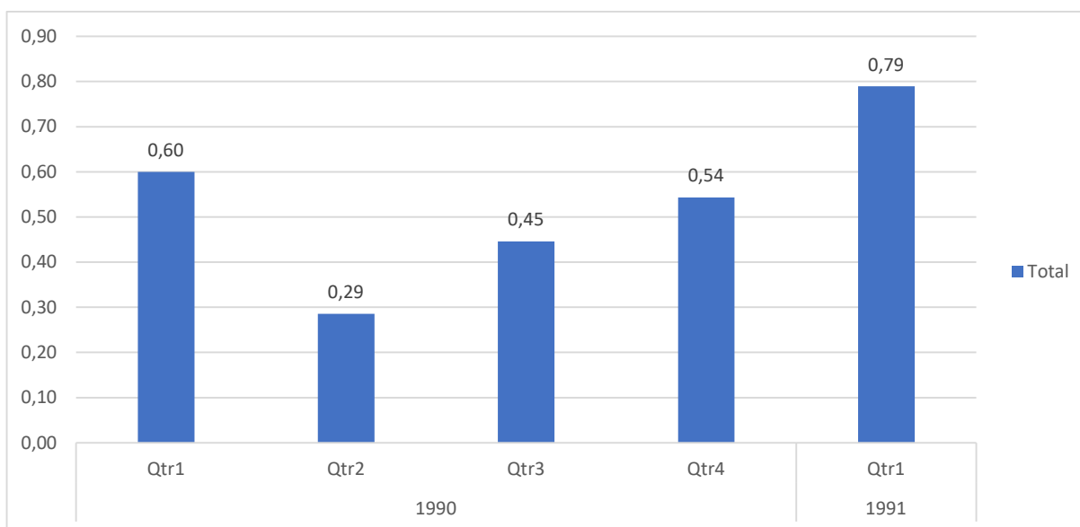
Слика 25 - Просечни број секуритизујућих потеза по дану за сваки квартал (Вечерњи новости)
