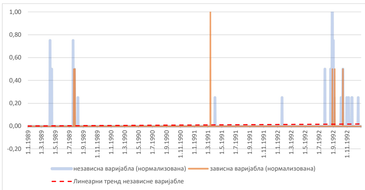
Слика 50 – Однос независне и зависне варијабле у дискурсу локалних актера
