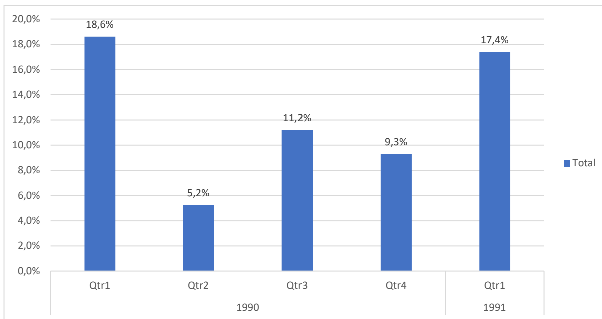
Слика 28 - Просечна површина насловне стране коју су заузимали секуритизујући потези на кварталном нивоу (Вечерње новости)
