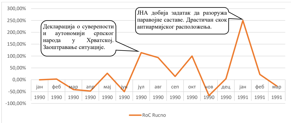
Слика 52 – Просечна промена броја ручно кодираних секуритизујућих потеза на насловним странама Вечерњег листа
