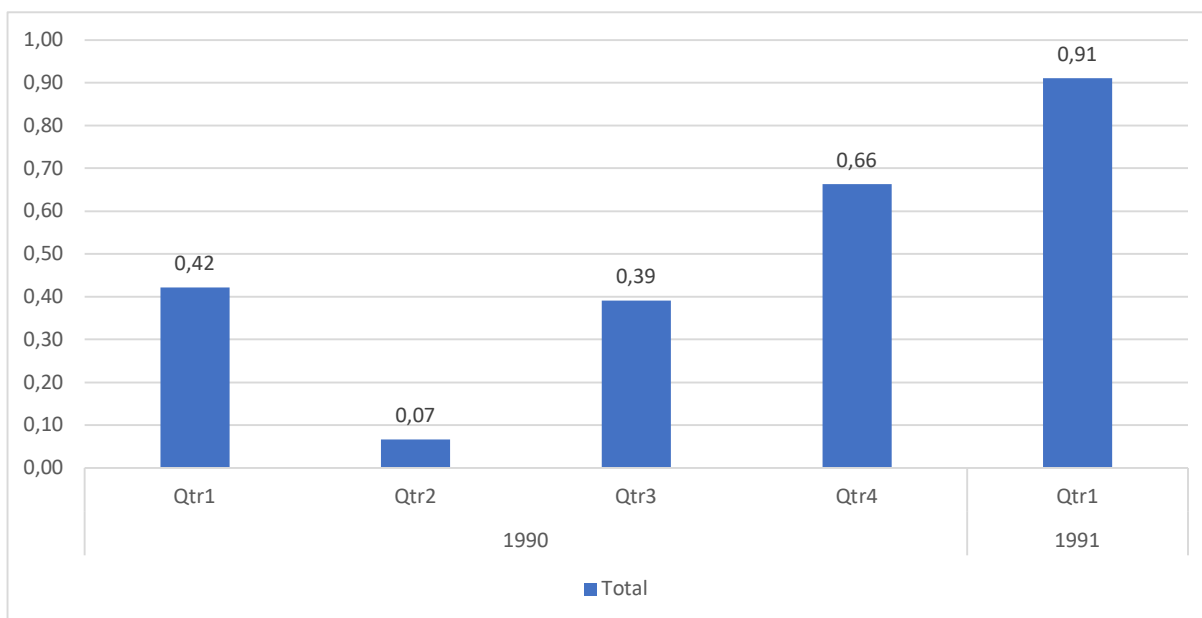
Слика 21 – Просечни број секуритизујућих потеза на кварталном нивоу (Вечерњи лист)
