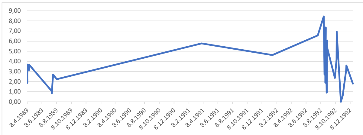
Слика 51 – Просечни тон секуритизујућих потеза (Абхазија)
