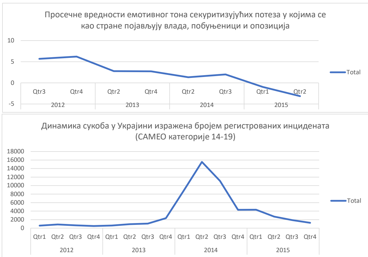
Слика 48 – Просечне вредности тона секуритизујућих потеза наспрам броја забележених инцидената (Украјина)
