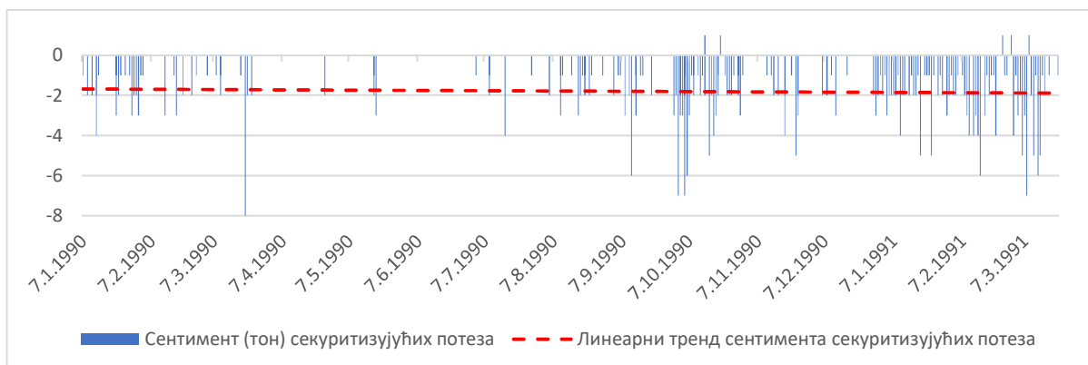
Слика 37 - Сентимент секуритизујућих потеза у Вечерњем листу
