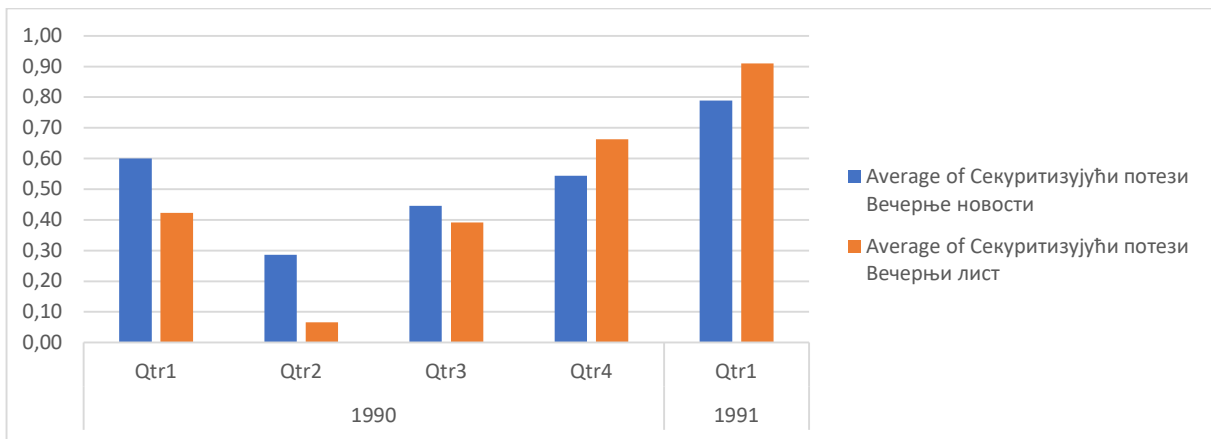
Слика 29 - Упоредни преглед просечног броја секуритизујућих потеза на насловним странама Вечерњег листа и Вечерњих новости током истраживаног периода
