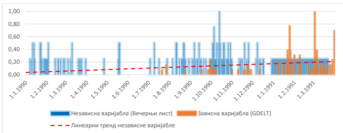
Слика 34 – Однос ручно кодиране независне и машински генерисане зависне варијабле (Вечерњи лист)
