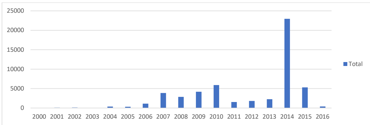
Слика 42 – Укупан број регистрованих секуритизујућих потеза (Украјина)
