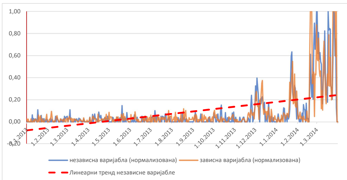
Слика 43 – Однос независне и зависне варијабле без филтрирања актера (Украјина)
