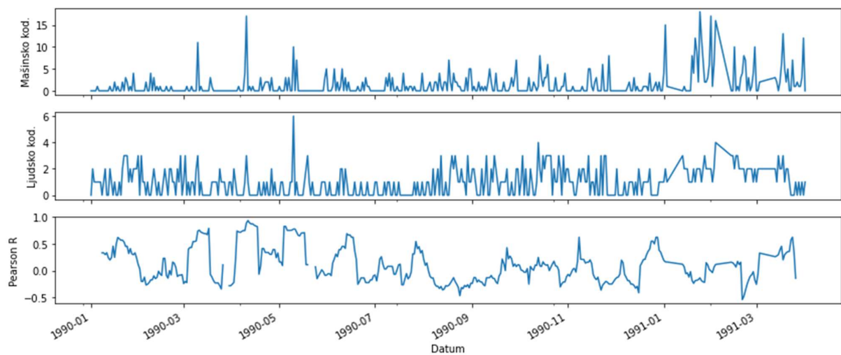
Слика 13 – Ручно наспрам машинског кодирања података (дневни ниво)
