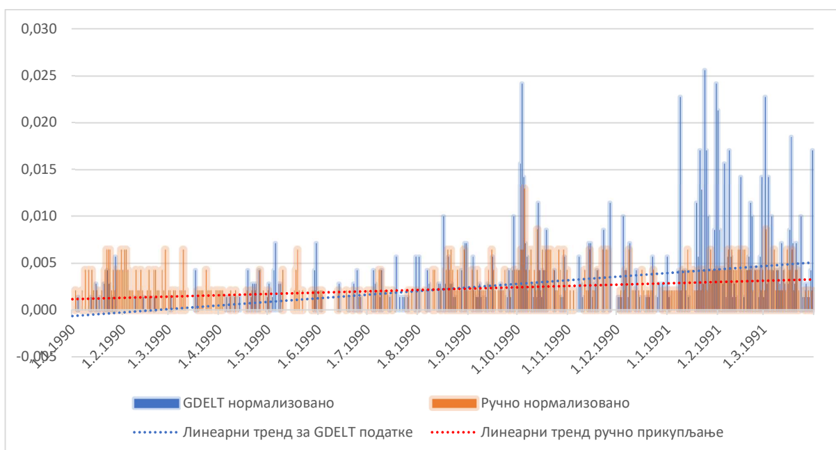
Слика 32 - Упоредни преглед нормализованих вредности машински и мануелно прикупљених података
