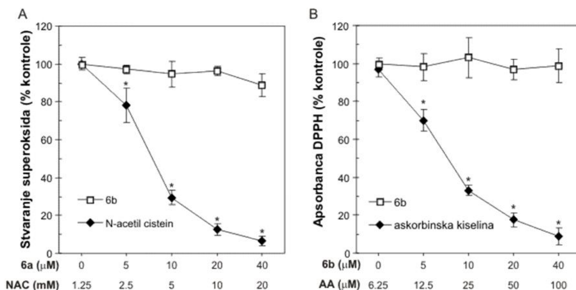
Slika 21. Antiradikalska aktivnost arilpiperazina 6b u odsustvu ćelija. (A, B) Različite koncentracije arilpiperazina 6b (5-40 \mu M) ili standardnog antioksidansa N-acetil cisteina (1.25-20 mM) (A) i
