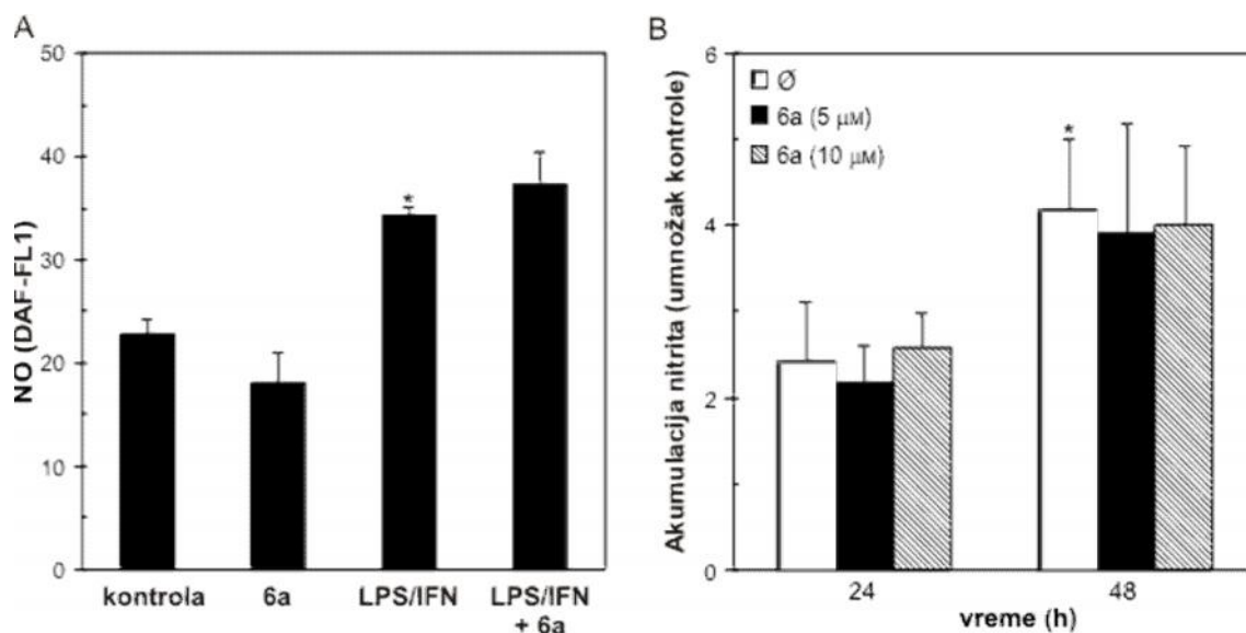
Slika 11. Uticaj arilpiperazina 6a na sintezu NO od strane stimulisanih makrofaga. Pacovski peritonealni makrofagi su stimulisani LPS-om (5 μg/ml) i IFN-γ (10 ng/ml) (A, B) i inkubirani sa arilpiperazinom 6a u jednoj (10 μM) (A) ili u dve koncentracije (5, 10 μM) (B). Nakon bojenja fluorescentnom bojom DAF, protočnom citofluorimetrijom je merena količina NO u stimulisanim makrofagima posle 24 časa (A), dok je akumulacija nitrita određena Grisovom metodom nakon 24 i 48 h (B). Rezultati su predstavljeni kao SV±SD iz 3 nezavisna eksperimenta. (*p < 0.05 označava statistički značajnu razliku u odnosu na kontrolne nestimulisane makrofage (A) ili makrofage stimulisane na produkciju NO u toku 24 časa (B)).
