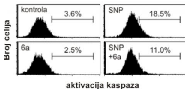
Slika 6. Uticaj arilpiperazina 6a na aktivaciju kaspaza izazvanu natrijum nitroprusidom u kulturi SH-SY5Y ćelija. SH-SY5Y ćelije su tretirane supstancom 6a (10 µM), a zatim izložene dejstvu SNP-a (2 mM) 24 časa. Nakon bojenja sa
