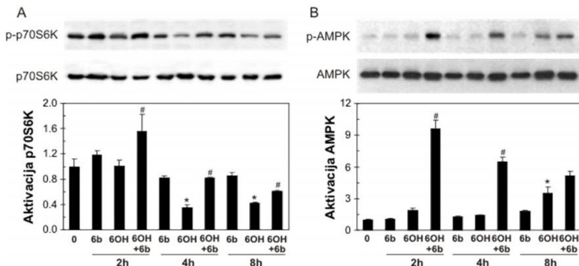
Slika 25. Uticaj arilpiperazina 6b na aktivnost AMPK i p70S6K proteina u SH-SY5Y ćelijama tretiranim 6-hidroksidopaminom. (A, B) SH-SY5Y ćelije su tretirane arilpiperazinom 6b (10 \mu M) i zatim izložene dejstvu 6-OHDA (60 \mu M) u toku 2, 4 i 8 časova. Fosforilisane i totalne forme AMPK i p70S6K proteina su određene imunoblot analizom, a njihova aktivnost je izražena kao odnos fosfo/total formi proteina, nakon kvantifikacije traka u ImageJ softveru (A, B, donji paneli). (* p < 0.05 označava statistički značajnu razliku u odnosu na kontrolu, dok # p < 0.05 označava statistički značajnu razliku u odnosu na ćelije tretirane 6-OHDA-om u odgovarajućem terminu).
