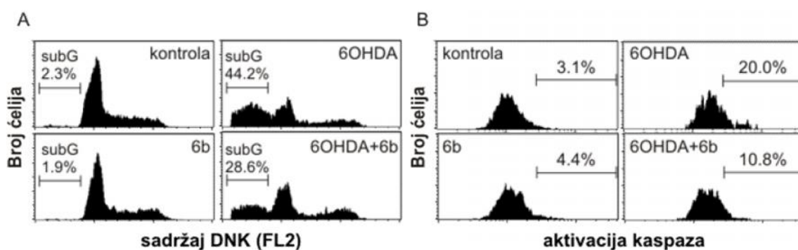
Slika 18. Uticaj arilpiperazina 6b na sadržaj DNK i aktivnost kaspaza u prisustvu 6-hidroksidopamina u kulturi SH-SY5Y ćelija. (A, B) SH-SY5Y ćelije su tretirane arilpiperazinom 6b (10 \mu M), a zatim su izložene dejstvu 6-OHDA (60 \mu M). Nakon 24 časa ćelije su bojene propidijum jodidom (A) ili ApoStat-om (B) i analizirane na protočnom citofluorimetru. Rezultati su prikazani u obliku histograma iz reprezentativnog, od 3 izvedena eksperimenta.
