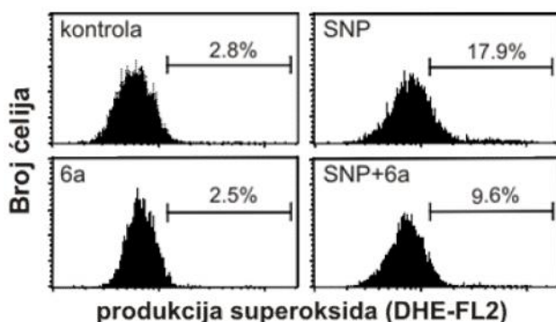
Slika 8. Uticaj arilpiperazina 6a na stvaranje superoksida izazvano natrijum nitroprusidom u kulturi SH-SY5Y ćelija. Kulture su tretirane najpre arilpiperazinom 6a (10 \mu M), a zatim izložene dejstvu SNP-a (2 mM). Nakon 24 ćasa ćelije su bojene fluorescentnom bojom DHE i broj ćelija sa povićanim sadržajem superoksida je praćen
