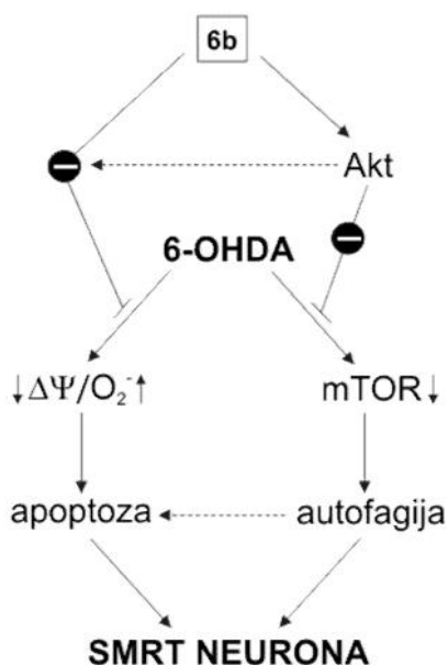
Shema 2. Pretpostavljeni mehanizam dejstva arilpiperazina 6b.
