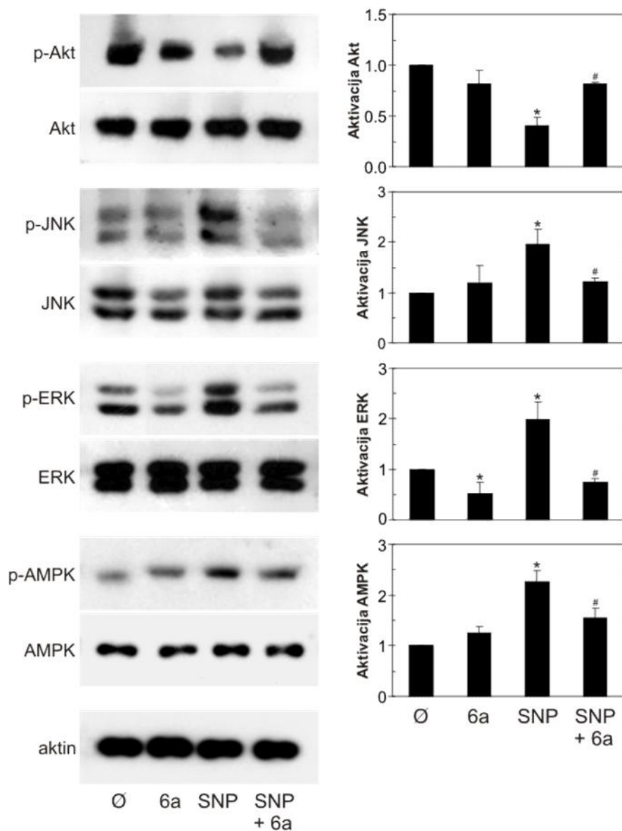
Slika 14. Uticaj arilpiperazina 6a na aktivnost signalnih puteva uključenih u regulaciju smrti SH-SY5Y ćelija tretiranih natrijum nitroprusidom. SH-SY5Y ćelije su tretirane arilpiperazinom 6a (10 \mu M), a zatim u narednih 8 časova izložene dejstvu natrijum nitroprusida (2 mM). Fosforilisane i totalne forme Akt, JNK, ERK, AMPK proteina, kao i aktina su određene imunoblot analizom, a aktivnost ovih signalnih puteva je izražena kao odnos fosfo/total formi proteina, nakon kvantifikacije traka u ImageJ softveru. (* p < 0.05 označava statistički značajnu razliku u odnosu na kontrolu, dok # p < 0.05 označava statistički značajnu razliku u odnosu na ćelije tretirane SNP-om).
