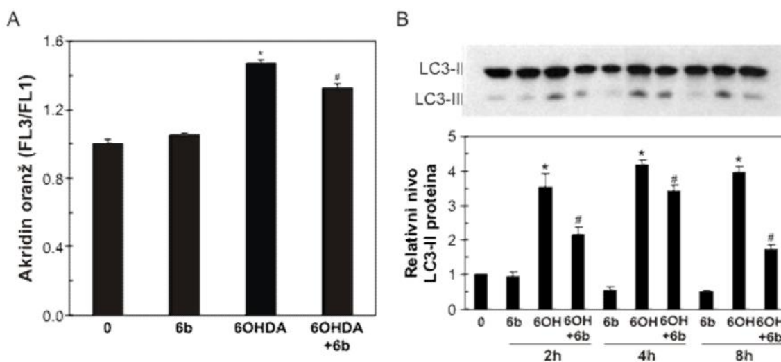
Slika 24. Uticaj arilpiperazina 6b na autofagiju izazvanu 6-hidroksidopaminom u kulturi SH-SY5Y ćelija. (A, B) SH-SY5Y ćelije su tretirane arilpiperazinom 6b (10 \mu M) i zatim izložene dejstvu 6-OHDA (60 \mu M). (A) Nakon 24 časa, ćelije su bojene akridin oranžom i analizirane na protočnom citofluorimetru. (B) Za imunoblot analizu LC3 proteina ćelije su lizirane nakon 2-, 4- i 8-očasovnog tretmana 6-OHDA-om. Rezultati su prikazani kao SV \pm SD iz dva urađena eksperimenta (A), a relativni nivo LC3-II proteina je određen kvantifikacijom traka u ImageJ softveru (B, donji panel). (* p < 0.05 označava statistički značajnu razliku u odnosu na kontrolu, dok # p < 0.05 označava statistički značajnu razliku u odnosu na ćelije tretirane 6-OHDA-om u odgovarajućem terminu).
