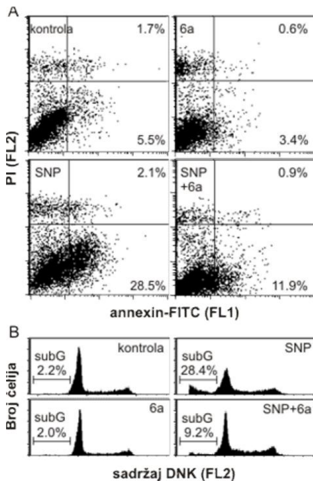
Slika 5. Uticaj arilpiperazina 6a na smrt SH-SY5Y ćelija izazvanu natrijum nitroprusidom. (A, B) SH-SY5Y ćelije su inkubirane u prisustvu ili odsustvu arilpiperazina 6a (10 µM) i u prisustvu ili odsustvu natrijum nitroprusida (2 mM). Nakon 24 časa ćelije su bojene aneksinom V-FITC/PI (A) ili PI (B) i analizirane na protočnom citofluorimetru. Rezultati su prikazani u vidu tačaka koje predstavljaju pojedinačne ćelije (dot plot) (A) ili histograma (B). Prikazani rezultati su iz reprezentativnog, od tri nezavisna eksperimenta.
