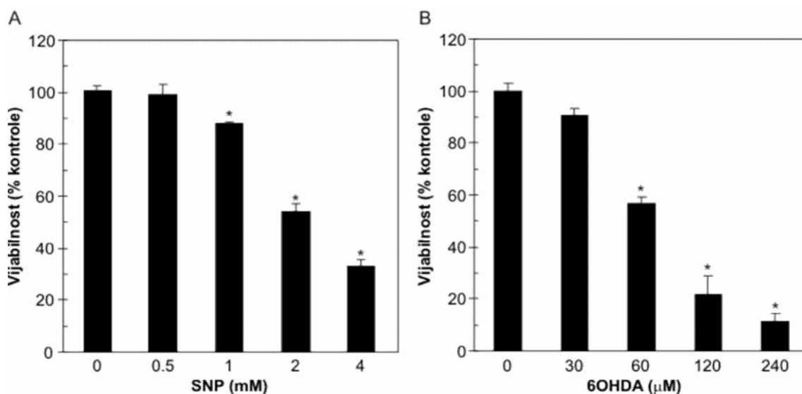
Slika 1. Uticaj natrijum nitroprusida i 6-hidroksidopamina na vijabilnost SH-SY5Y ćelija. SH-SY5Y ćelije su inkubirane sa različitim koncentracijama SNP-a (0.5-4 mM) (A) i 6-OHDA (30-240 \mu M) (B) i vijabilnost je određena testom aktivnosti kisele fosfataze nakon 24 sata. Rezultati su prikazani kao SV \pm SD triplikata kultura iz jednog od 3 eksperimenata. (* p < 0.05 označava statistički značajnu razliku između tretiranih i kontrolnih ćelija). Rezultati vijabilnosti su prikazani kao % kontrole, pri čemu je za kontrolu uzeta vrednost aktivnosti kisele fosfataze u netretiranim kulturama.
