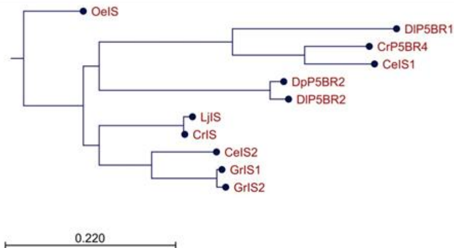
Слика П3. Филогенетска анализа аминокиселинских секвенци ензима CeIS1 и CeIS2 која показује њихову повезаност са осталим познатим иридоид синтазама и прогестерон-5- \beta -редуктазама. Филогенетско стабло је конструисано коришћењем neighbor-joining методе CLC sequence viewer 8.0 софтверског пакета. У Табели П3 прилога приказани су описи коришћених скраћеница за биљне врсте и приступни бројеви ензима у on line базама података.
