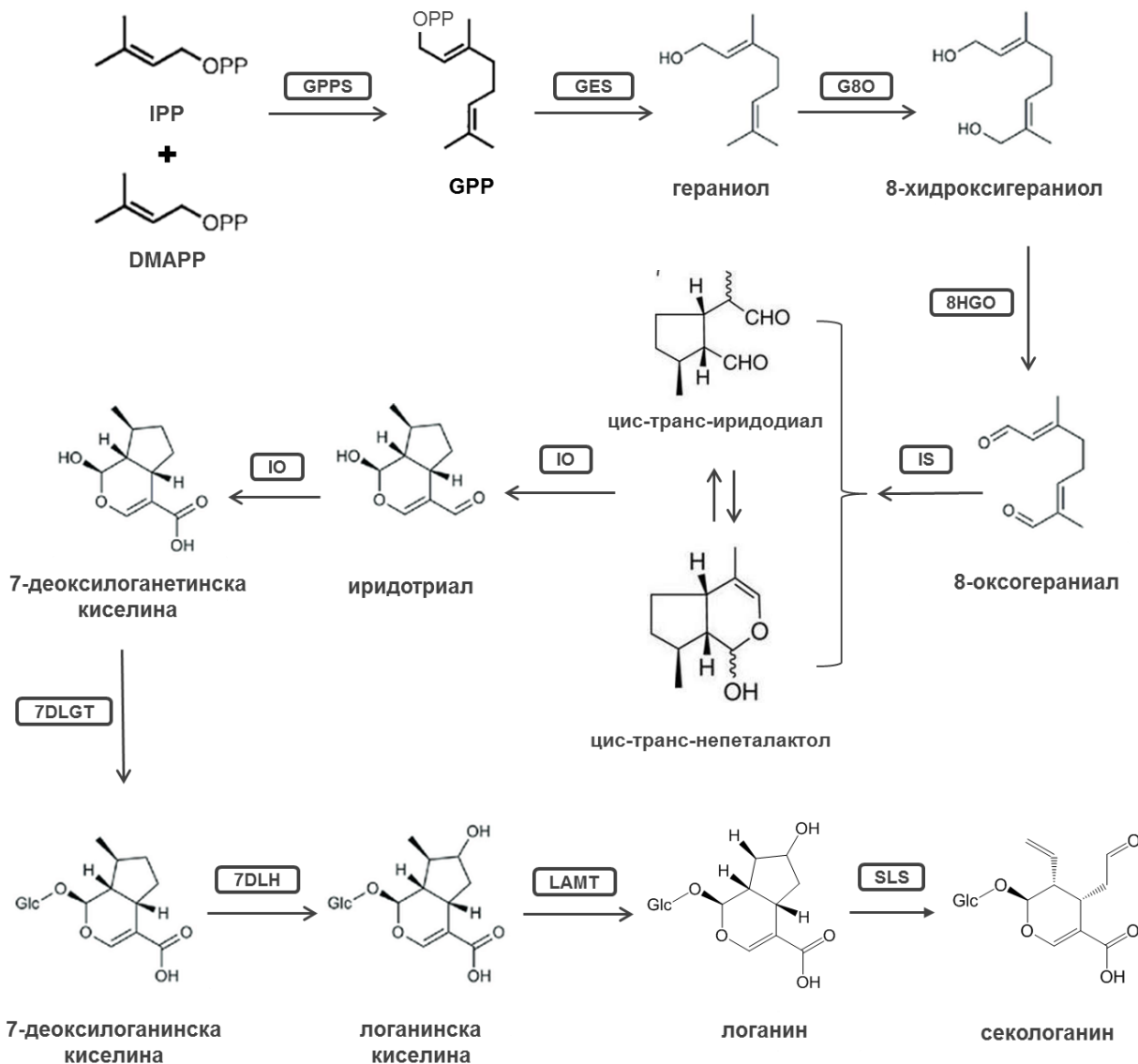
Слика 5. Пут синтезе секоидридоида секологанина (СЛОГ) код врсте C. roseus . Приказана су претпостављена једињења и ензими који посредују у биосинтези. Скраћенице: IPP -изопентенил пирофосфат, DMAPP -диметилалил пирофосфат, GPP геранил дифосфат, GPPS геранил дифосфат синтаза, GES гераниол синтаза, G8O гераниол 8-оксидаза, 8HGO 8-хидроксигераниол оксидоредуктаза, IS иридоид синтаза, IO иридоид оксидаза, 7DLGT глукозил трансфераза 7-деоксилоганетинске киселине, 7DLH хидроксилаза 7-деоксилоганинске киселине, LAMT О-метилтрансфераза логанинске киселине, SLS СЛОГ синтаза.
