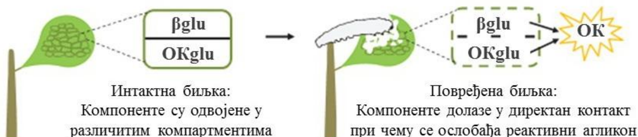
Слика 8. Двокомпонентни одбрамбени одговор биљке у коме се глюкозилована одбрамбена компонента (OKglu) активира у контакту са ензимом \beta -глюкозидазом ( \beta glu) при оштећењу ткива повређивањем (напад хербивора). Након хидролизе OKglu ослобађа се одбрамбена компонента - реактивни агликон (OK) (према Pentzold и сарадници (2014), измењено).
