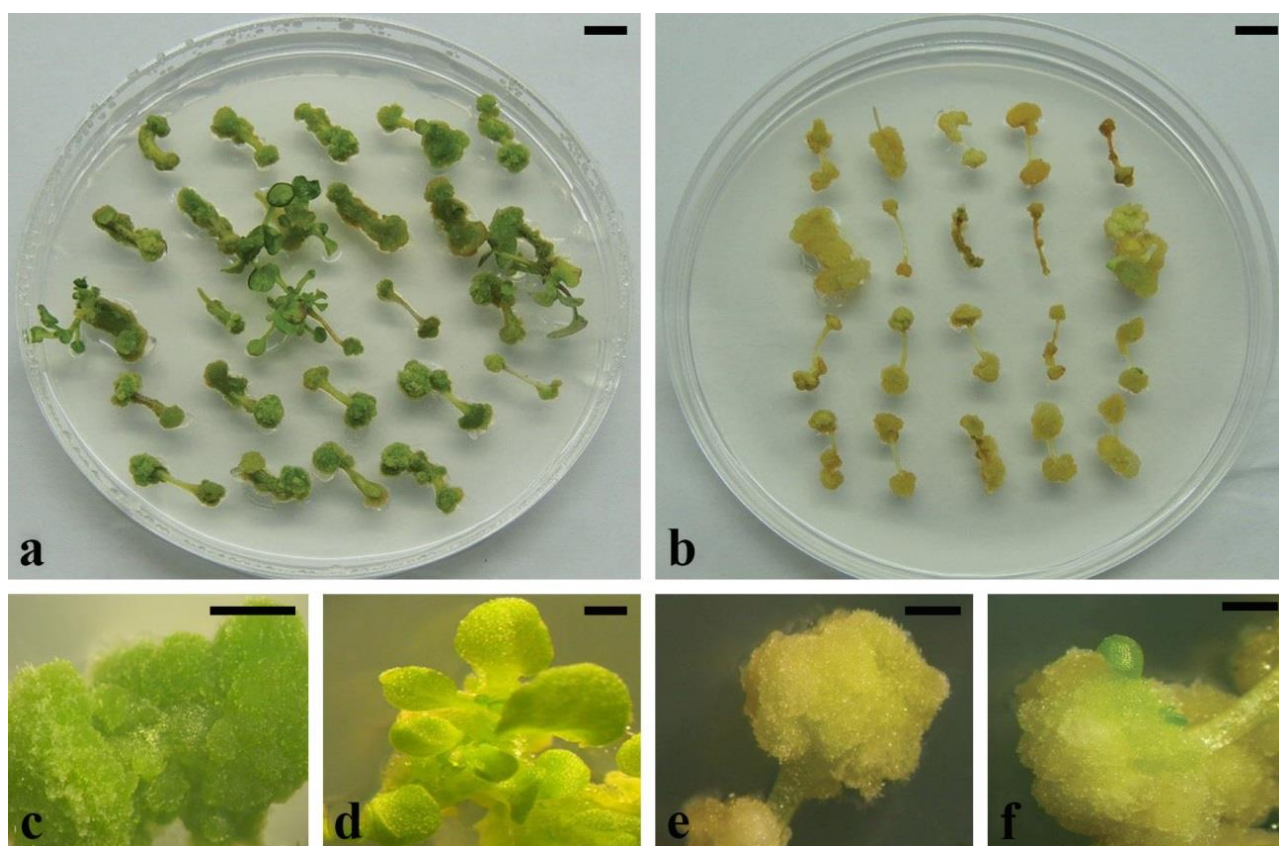
Slika 11. Uticaj svetlosti na indukciju formiranja kalusa i izdanaka na odsećima hipokotila V. cornuta posle 4 nedelje gajenja na \frac{1}{2} MS hranljivoj podlozi sa 0,1 mg/l 2,4-D i 2,0 mg/l BAP. a - odsećci hipokotila gajeni u uslovima dugog dana; b - odsećci hipokotila gajeni 24h u mraku; c - kalus formiran na odsečku hipokotila u uslovima dugog dana; d - adventivni izdanci formirani u uslovima dugog dana; e - formirani kalus na odsečku hipokotila gajenom u mraku; f - adventivni izdanci formirani na eksplantatu hipokotila gajenom u mraku. Bar = 5 mm (a, b); bar = 2 mm (c-f).
