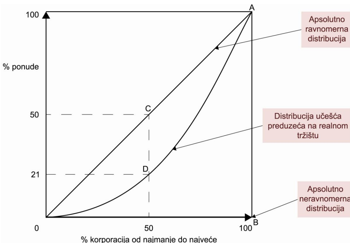
Prikaz 4-5: Lorencova kriva
