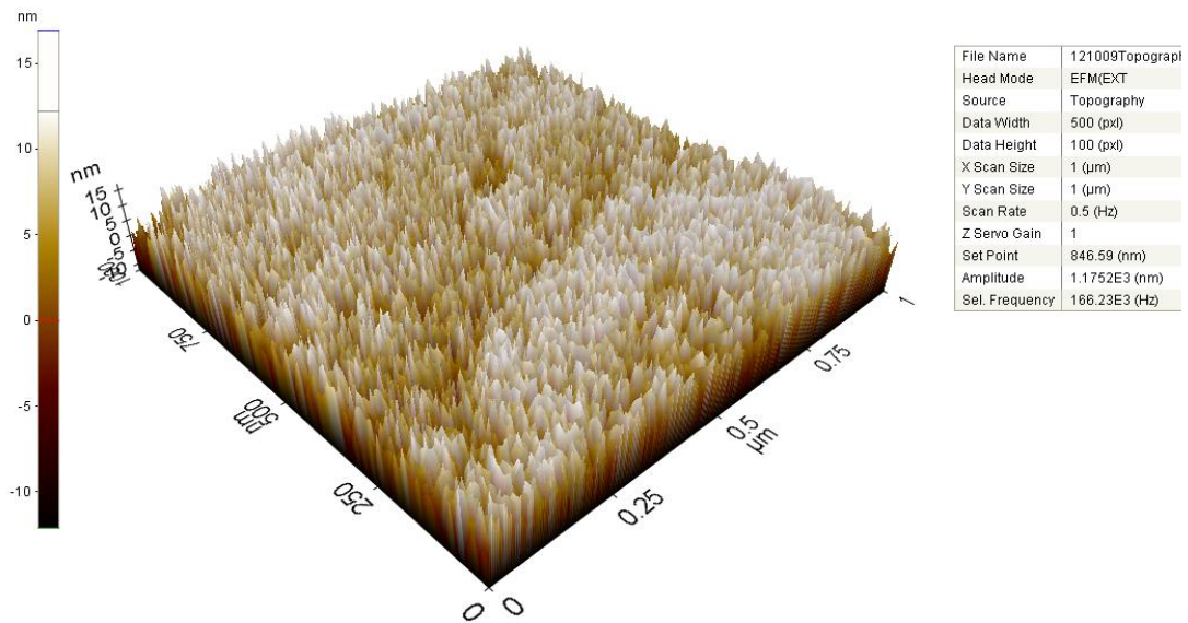
Sl. II-6: Rezultat AFM merenja uzorka koji je tretiran na T=500^\circ\text{C} , w=5\text{mm/s} . Skenirana je površina uzorka od 1\mu\text{m}^2 . Na z-osi data je varijacija visine uzorka na osnovu koje se dobija hrapavost površine uzorka.
