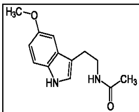
Slika 22. Hemijska struktura melatonina
