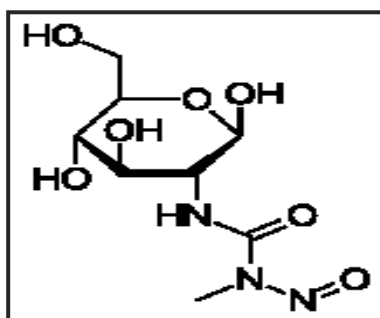
Slika 21. Hemijska struktura streptozotocina.
