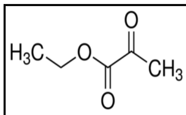
Slika 23. Hemijska struktura etil piruvata
