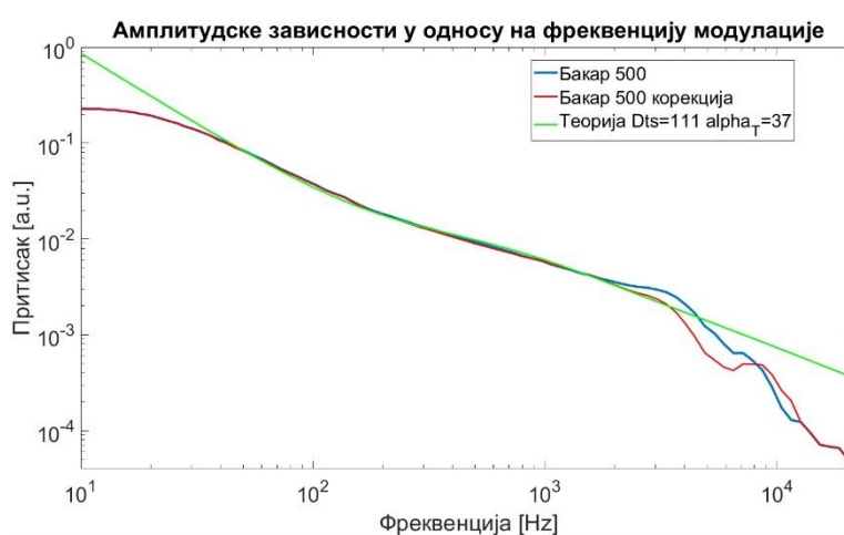
Слика 9.13: Зависност амплитуде ФА одзива од модулационе фреквенције одређена са и без корекције са функцијом преноса ФАМС за бакар дебљине а) 280 \mu\text{m} и б) 500 \mu\text{m} .
