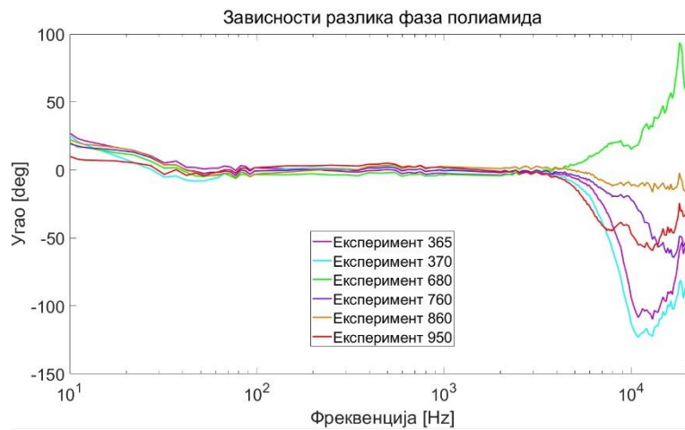
Слика 9.16: Нормализовани \Phi A одзиви узорка полиамида при побуди ласерском диодом: а) однос амплитуда и б) разлика фаза.
