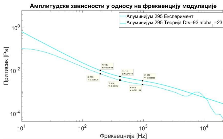
Слика 9.32: Зависност амплитуде притиска од модулационе фреквенције одређена експериментално и теоријски за узорке алуминијума дебљине а) 185 \mu\text{m} и б) 295 \mu\text{m} .
