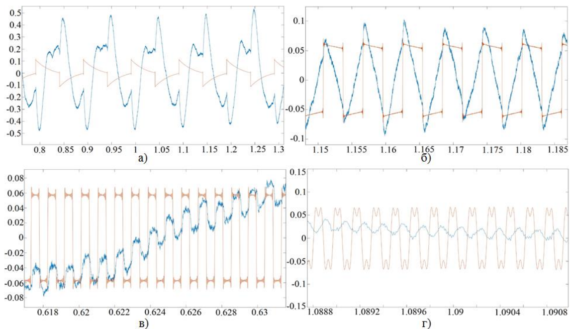
Слика 7.23: Мерењи сигнали ФА одзива узорка алуминијума дебљине 295 \mu\text{m} при модулацији правоугаоним импулсима, побуди ласером и појачању 300. Модулациона фреквенција: а) 10 Hz, б) 170 Hz, в) 1070 Hz и г) 6070 Hz.
