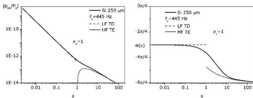
Слика 3.1 (преузето из [32]): Амплитудске и фазне зависности израчунате на основу теоријског модела за узорке а) полиетилена дебљине 10 \mu\text{m} , б) силицијума дебљине 3 \text{mm} и в) силицијума дебљине 250 \mu\text{m} . Апсциса x представља односе модуларне фреквенције и карактеристичне фреквенције узорка, док x_s означава однос пресечне и карактеристичне фреквенције узорка.
