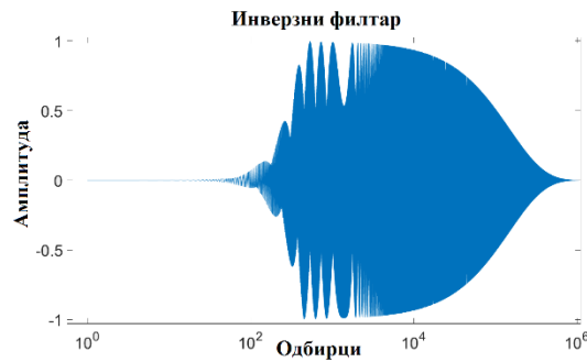
Слика 7.7: Инверзни филтар (логаритамска апсциса).
