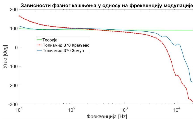
Слика 9.6: Зависност а) амплитуде и б) фазног кашњења у односу на фреквенције модулације код узорка полиамида дебљине 370 \mu\text{m} .
