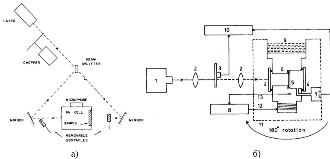
Слика 4.8 (преузето из [73] и [74]): а) Експериментална поставка ФА мерења термичке дифузивности са два ласерска снопа и б) ротирајућом ФА хелијом.
