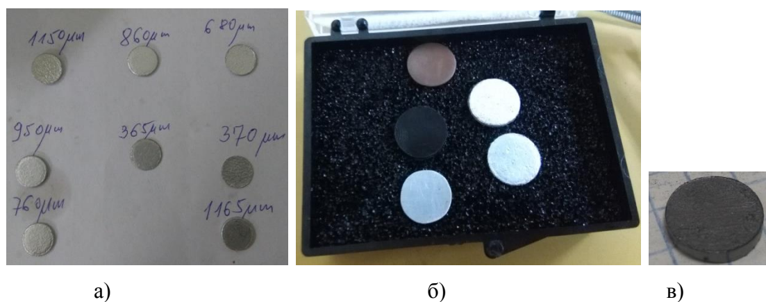
Слика 6.36: Узорци а) од полиамида различитих дебљина, б) пет узорака за упоредна испитивања и в) узорак од графита.
