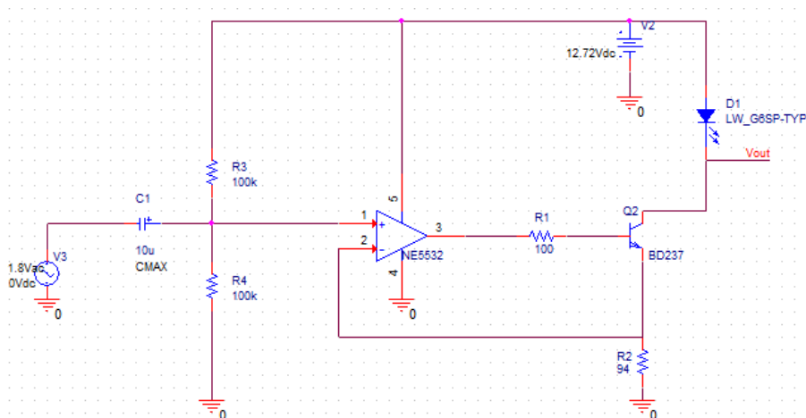
Слика 6.11: Електрична шема другог модулятора, пројектованог само за прикључење ласерске диоде.
