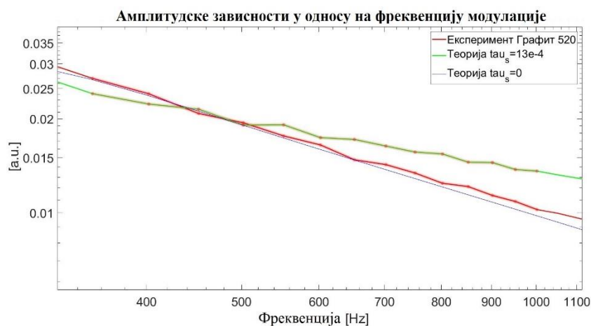
Слика 9.30: Зависност амплитуде ФА одзива од модулационе фреквенције узорка графита дебљине 520 \mu\text{m} фитована према теоријским моделима од којих једна урачунава ефекте топлотне меморије.
