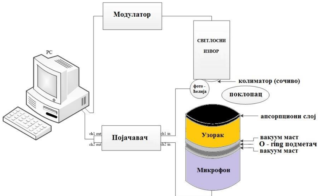
Слика 4.5: Принципијелна шема ФАМС са open-ended трансмисионом ФА ћелијом.
