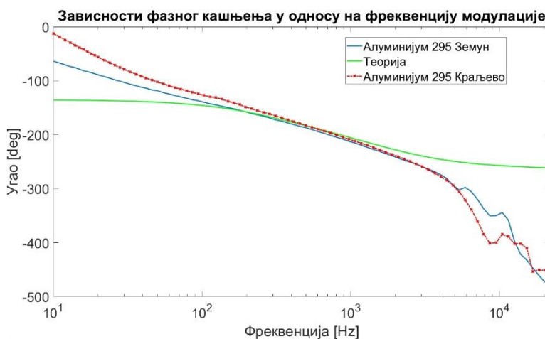
Слика 9.4: Зависност а) амплитуде и б) фазног кашњења у односу на фреквенције модулације код узорка алуминијума.
