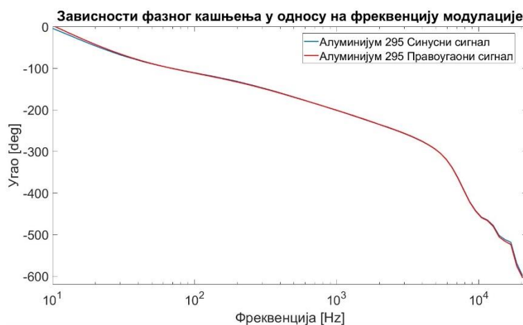
Слика 9.14: Упоредни приказ резултата приликом примене синусних и правоугаоних побудних сигнала на узорак алуминијума дебљине 295 \mu\text{m} за зависности а) амплитуде и б) фазног кашњења у односу на фреквенцију модулације.
