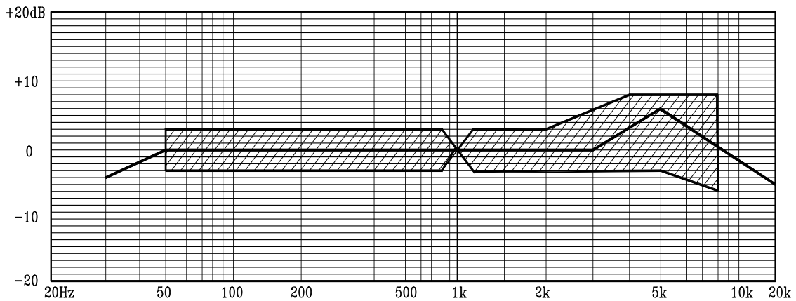
Слика 5.2: Типична амплитудско-фреквенцијска карактеристика микрофона [80].
