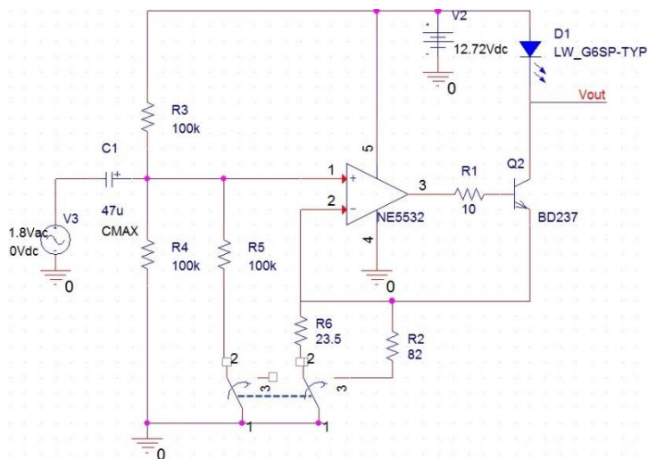
Слика 6.10: Електрична шема првог модулатора, који може напајати LED и ласерске диоде.
