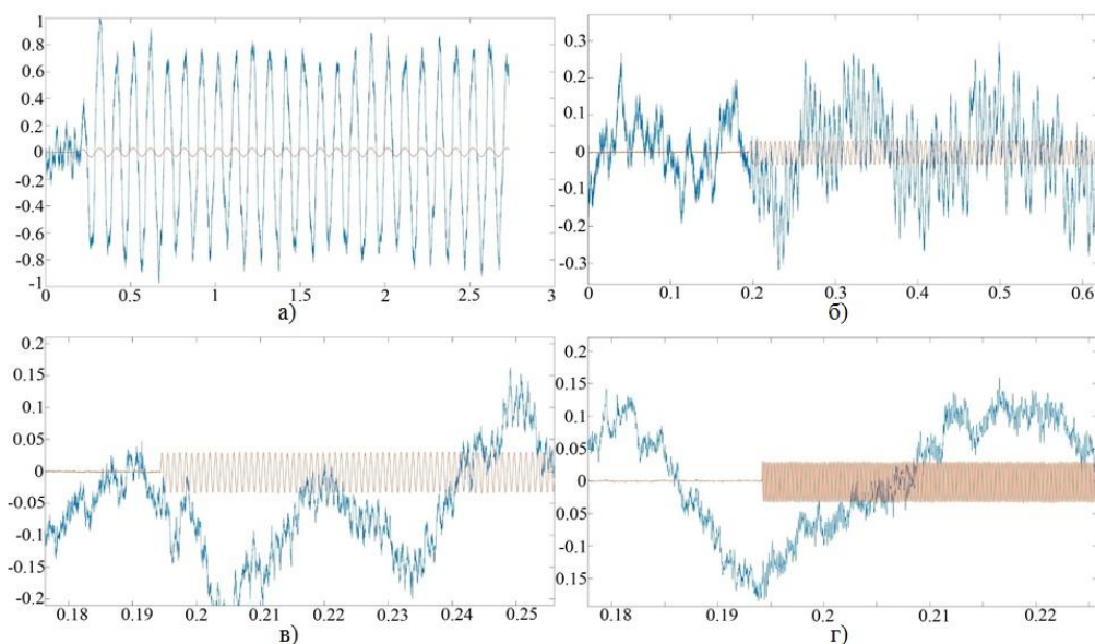
Слика 7.19: Мерени сигнали ФА одзива узорка полиамида дебљине 370 \mu\text{m} при хармонијској модулацији, побуди LED и појачању 300. Модулациона фреквенција: а) 10 Hz, б) 170 Hz, в) 1070 Hz и г) 6070 Hz.
