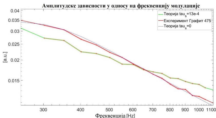
Слика 9.29: Зависност амплитуде ФА одзива од модулатионе фреквенције узорка графита дебљине 475 микрон фитована према теоријским моделима од којих једна урачунава ефекте топлотне меморије.
