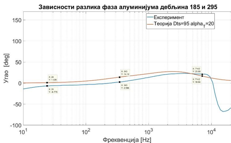
Слика 9.17: Усаглашавање поклапања зависности а) односа амплитуда и б) разлике фаза, са теоријским зависностима код алуминијума на две дебљине, ради добијања јединственог резултата за термичке параметре.
