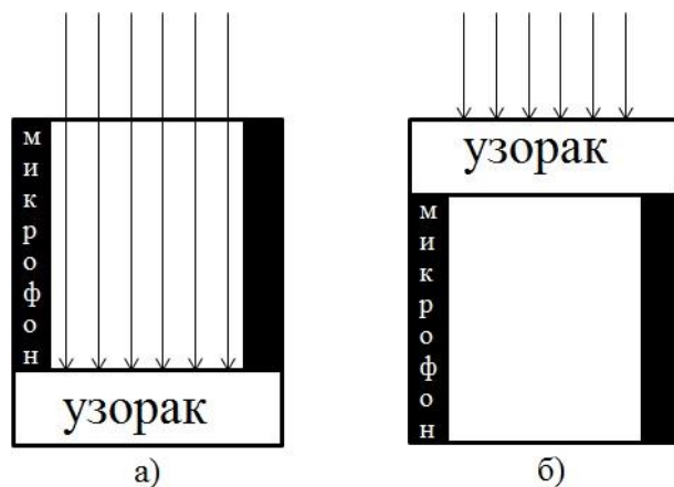
Слика 4.2: Концепт ФА мерења у а) рефлексионој и трансмисионој конфигурацији.
