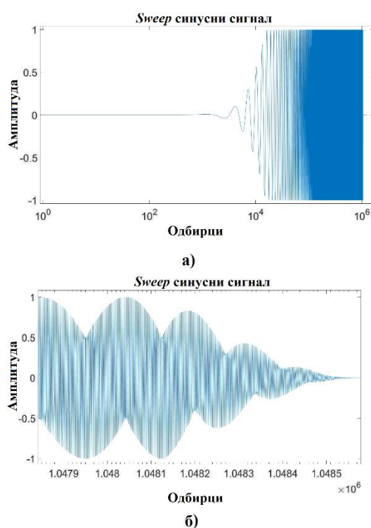
Слика 7.6: Sweep сигнал, а) „fade-in“ и б) „fade-out“ (оба графикаона имају логаритамске апсцисе).
