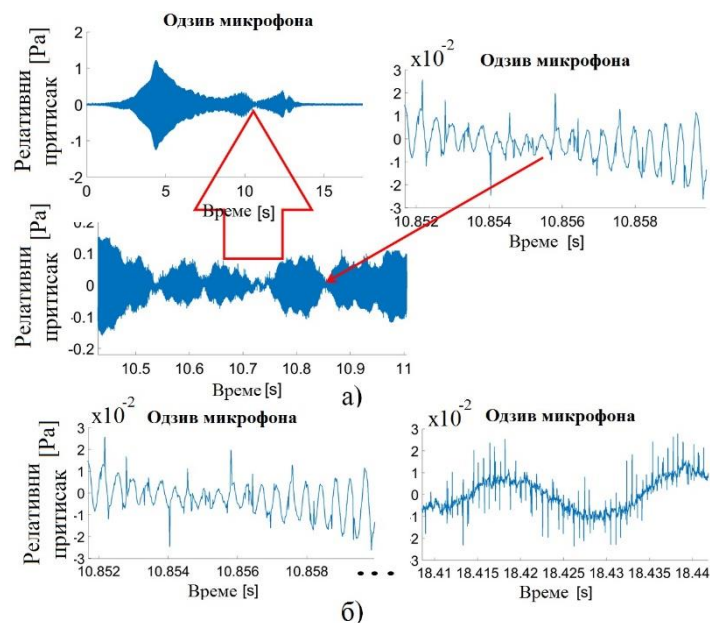
Слика 8.5: Сигнал измерен микрофоном KECG2742TBL-A пречника 6 mm а) место са најмањом амплитудом сигнала и б) упоредни приказ сигнала најмање амплитуде и шума.
