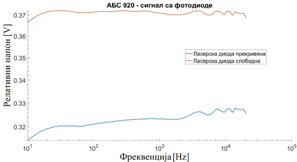
Слика 7.20: Зависност мерене амплитуде сигнала фотодиоде од модулационе фреквенције при откривеном и прекривеном светлосном извору.
