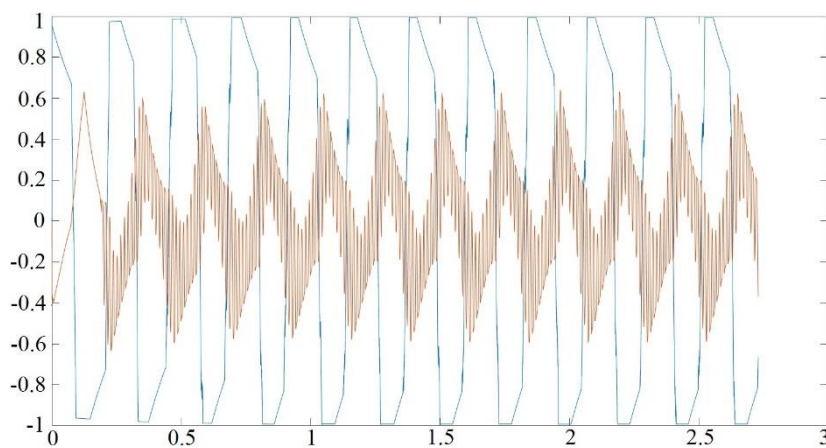
Слика 7.22: Појава „микрофоније“ приликом мерења са ФАМС.
