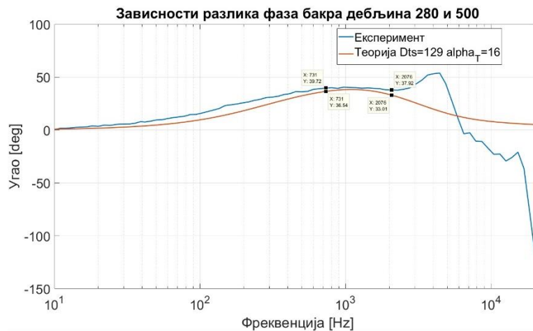
Слика 9.18: Усаглашавање поклапања зависности а) односа амплитуда и б) разлике фаза, са теоријским зависностима код бакра на две дебљине, ради добијања јединственог резултата за термичке параметре.
