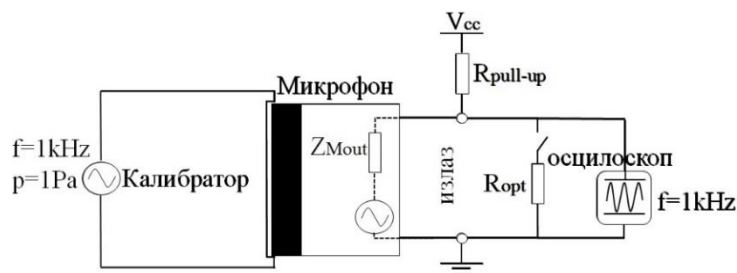
Слика 7.13: Електрична шема експерименталне апаратуре за одређивање излазне импедансе микрофона.
