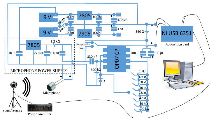
Слика 7.5: Шема експерименталне апаратуре за карактеризацију микрофона помоћу sweep сигнала.
