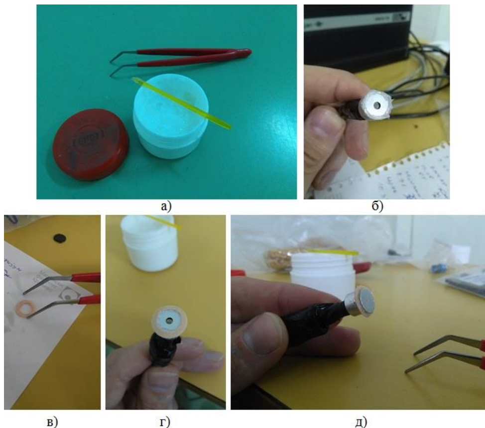
Слика 7.28: Техника и поступак наношења узорка, а) вакуум маст, б) вакуум маст нанесена на микрофон, в) наношење вакуум масти на O-ring подметач, г) O-ring подметач постављен на микрофон и д) узорак стављен на O-ring подметач.
