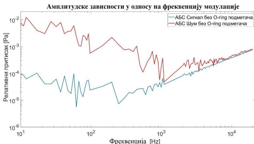
Слика 9.24: Зависност амплитуде ФА одзива од модулационе фреквенције мерена на узорку од АБС пластике дебљине 920 \mu\text{m} без O-ring подметача.
