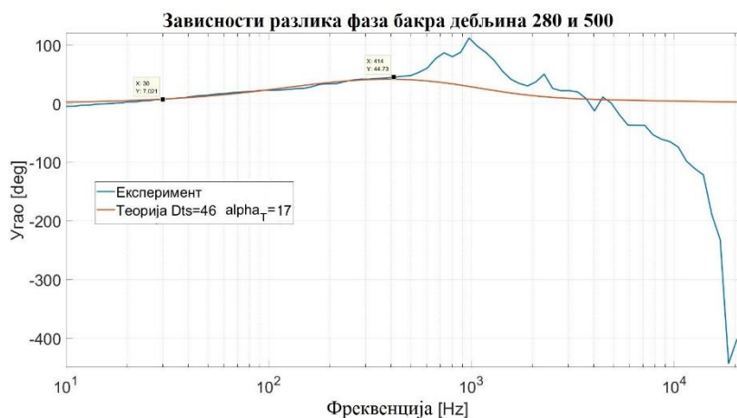
Слика 9.22: Нормиране зависности \Phi A одзива од модулационе фреквенције за две дебљине бабра, приказане упоредо са теоријским зависностима, а при побуди ласерске диоде од 35 mW оптичке снаге.
