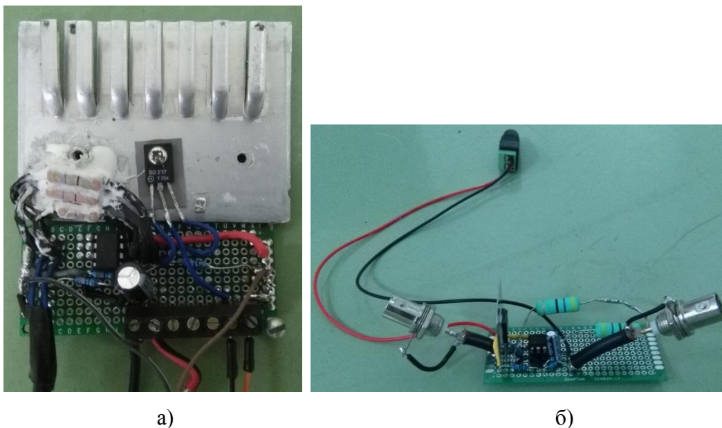
Слика 6.17: Електрична кола залемљена на плочицама а) првог модулатора и б) другог направљеног модулатора.
