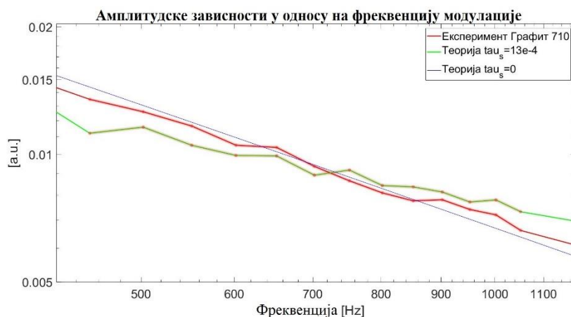
Слика 9.31: Зависност амплитуде ФА одзива од модулационе фреквенције узорка графита дебљине 710 \mu\text{m} фитована према теоријским моделима од којих једна урачунава ефекте топлотне меморије.
