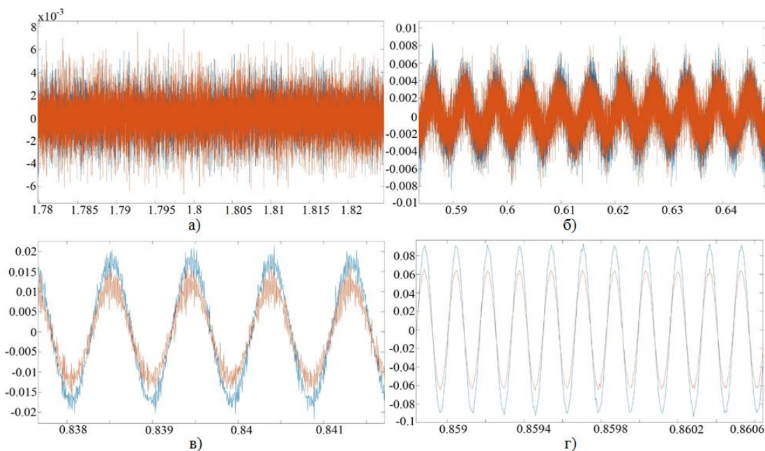
Слика 7.15: Експериментално одређени сигнали на отвореним микрофонским улазима када се на отворени излаз звучне картице пошаљу сигнали фреквенције: а) 10 Hz, б) 170 Hz, в) 1070 Hz и г) 6070 Hz.
