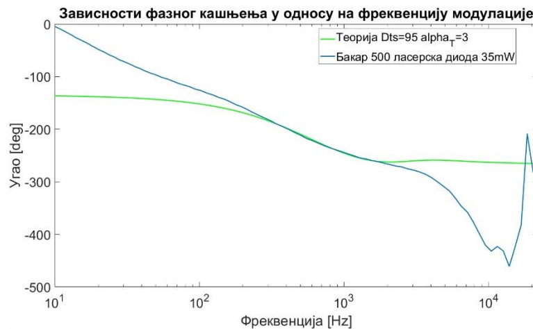
Слика 9.21: Зависности \Phi A одзива од модулационе фреквенције за узорак од бакра дебљине 500 \mu\text{m} , који је побуђен ласерском диодом од 35 mW.
