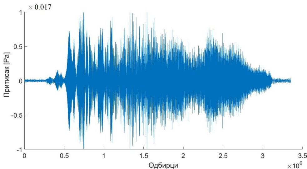
Слика 7.12: Временски одзив са микрофона, експериментално одређен за sweep побуду.
