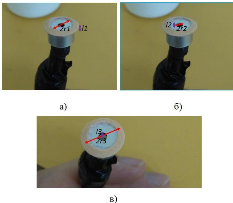
Слика 6.21: Запремину ФА ћелије чине три запремине: а) запремина коју ограничавају O-ring подметач, узорак и спољна површина капсуле микрофона, б) запремина отвора на микрофону и в) запремина у микрофону (налази се испод отвора, а простире се до мембране).
