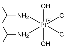
Pt(ipa)(OH) 2 Cl 2
