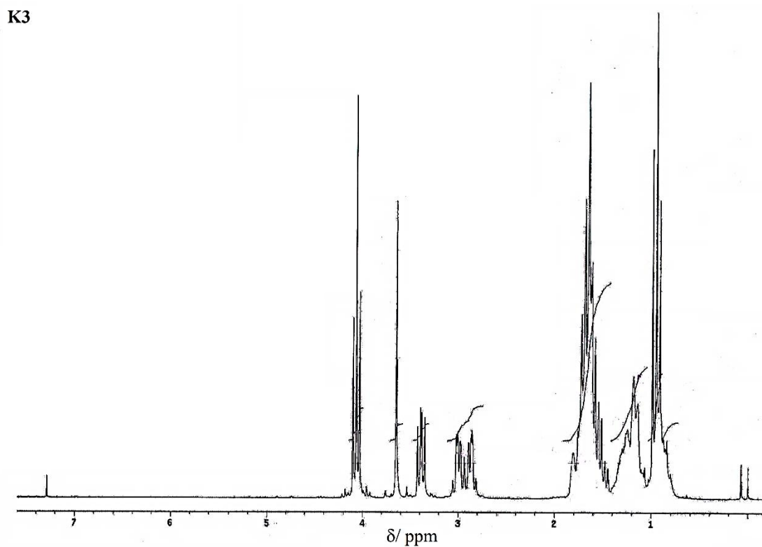
Slika P44. 1 H NMR spektar kompleksa K3 .
