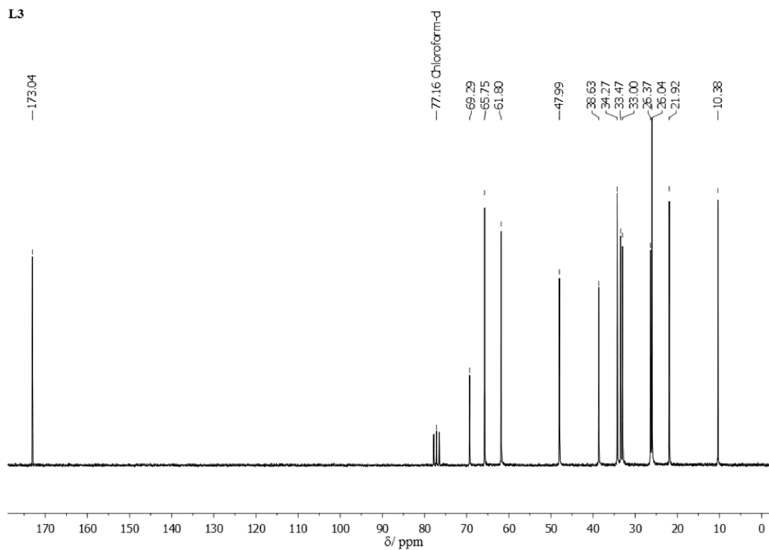
Slika P14. ^{13}\text{C} NMR spektar liganda L3.
