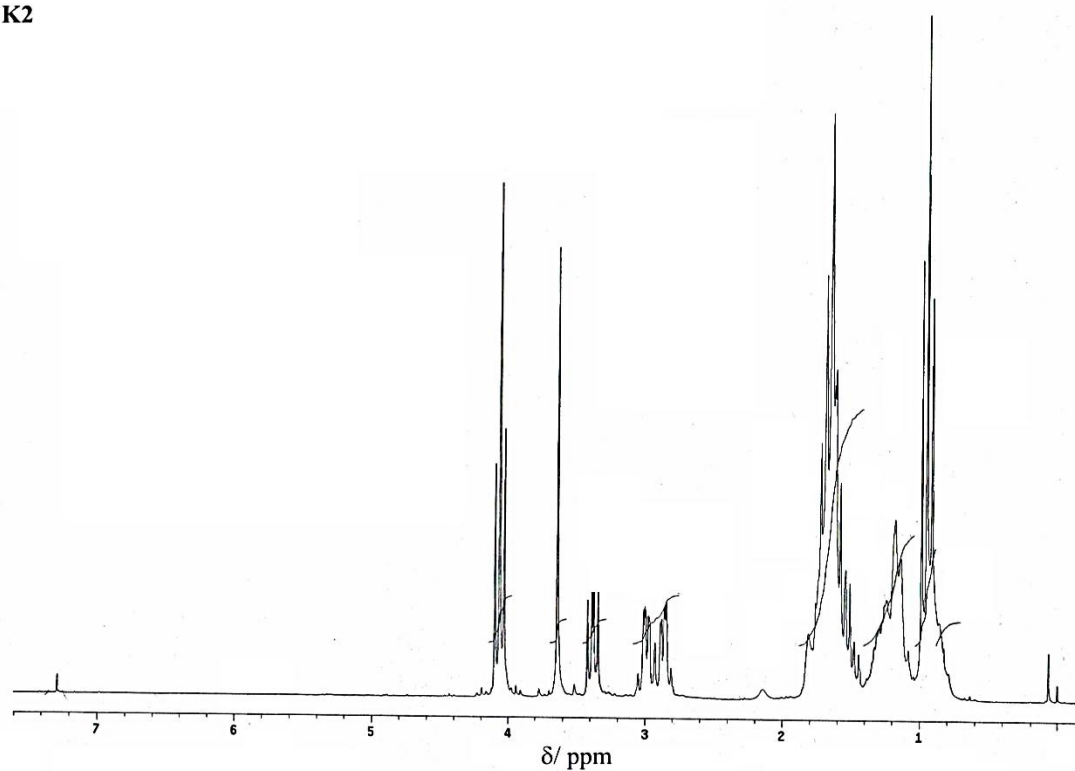
Slika P39. ^1\text{H} NMR spektar kompleksa K2.
