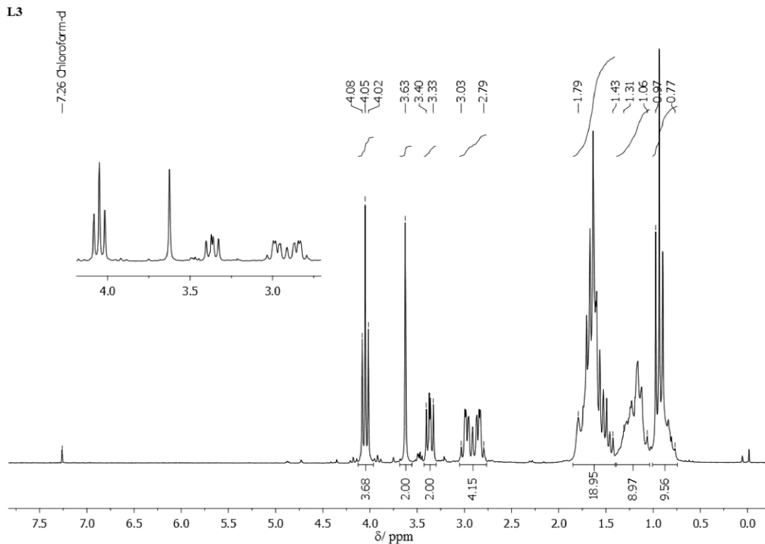
Slika P13. ^1\text{H} NMR spektar liganda L3.
