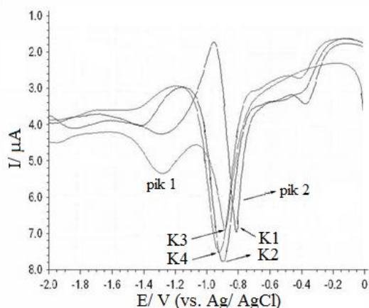
Slika 30. DP voltamogrami 0,1 mmol/dm 3 rastvora kompleksa K1-4 u DMSO-u; pomoćni elektrolit LiClO 4 .
