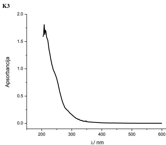
Slika P48. Ultraljubičasti spektar kompleksa K3 .
