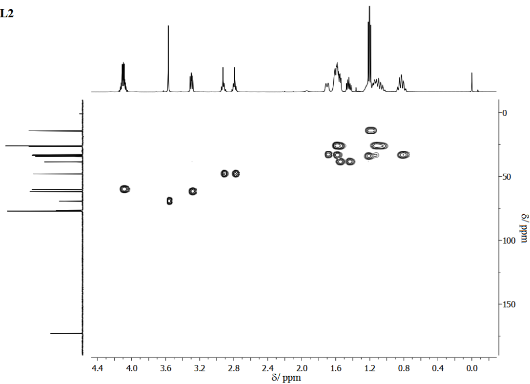
Slika P9. HSQC NMR spektar liganda L2.
