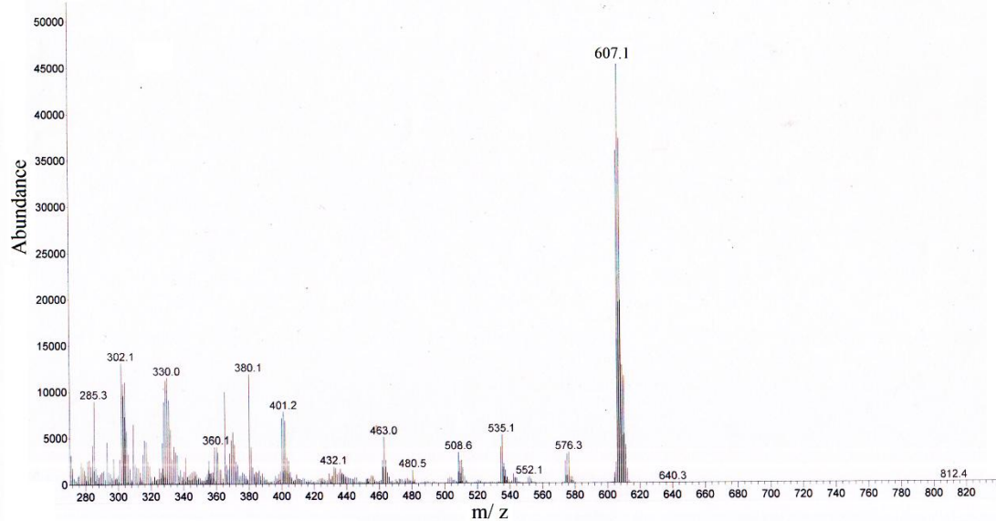
Slika P56. Maseni spektar kompleksa K5.
