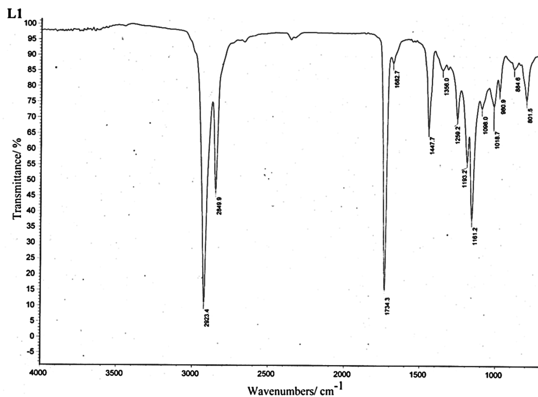
Slika P4. Infracrveni spektar liganda L1.
