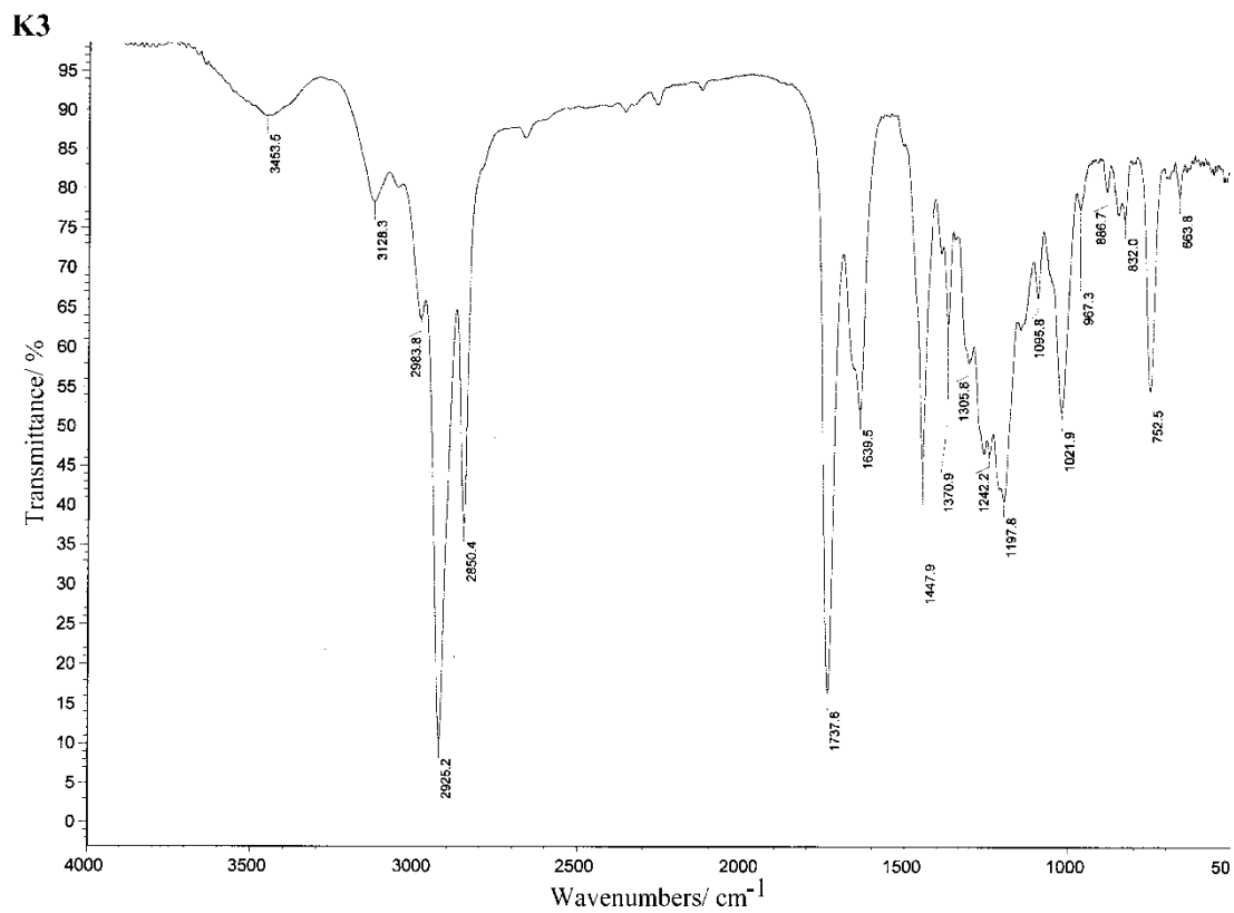
Slika P47. Infracrveni spektar kompleksa K3 .
