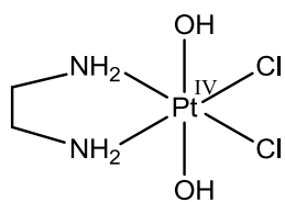
Pt(en)(OH) 2 Cl 2
