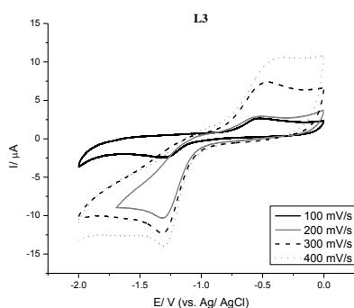
Slika 27. a) Ciklični voltamogrami 0,1 \text{ mmol}/\text{dm}^3 rastvora liganda L3 u DMSO-u pri različitim vrednostima brzina polarizacije (100, 200, 300 i 400 \text{mV/s} ); b) zavisnost jačine struje oksidacionog i redukcionog pika od kvadratnog korena brzine snimanja.
