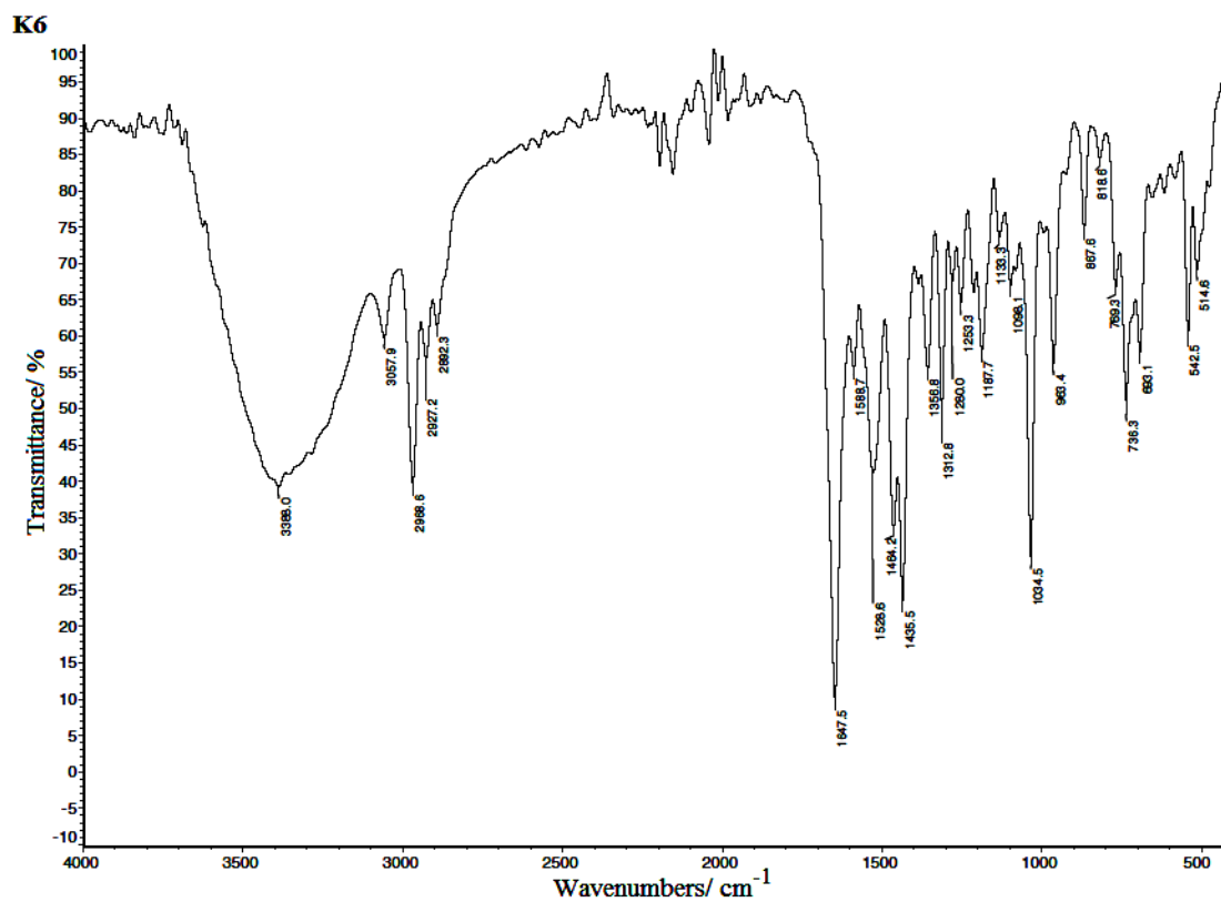
Slika P62. Infracrveni spektar kompleksa K6 .
