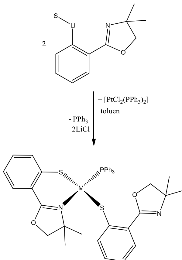
Šema 11. Sinteza kompleksa K6 , [Pt( \eta^2 S-Phoz)( \eta^1 S-Phoz)(PPh 3 )].
