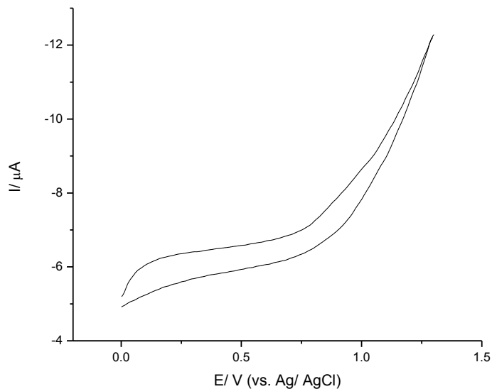
Slika P63. Ciklični voltamogram 0,1 mmol/dm 3 rastvora elektrolita LiClO 4 u DMSO-u u oblasti potencijala 0 < E < 1,3 \text{ V} pri brzini polarizacije 25 mV/s.
