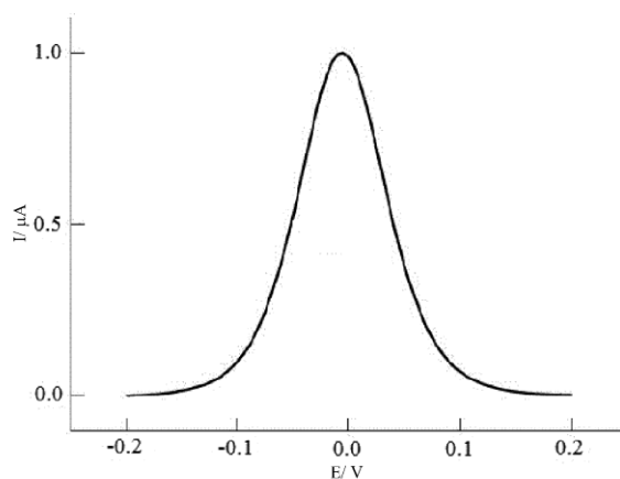
Slika 16. Oblik pika u diferencijalnoj pulsnoj voltimetriji.
