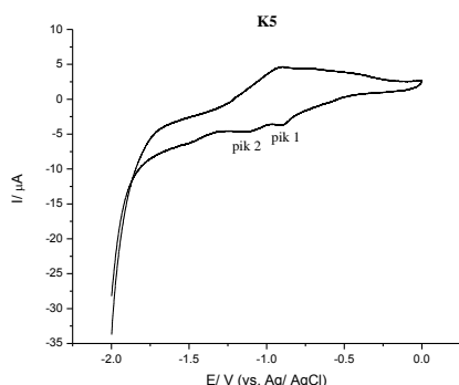
Slika 31. Ciklični voltamogrami 0,1 mmol/dm 3 rastvora kompleksa K5 u DMSO-u u oblasti potencijala: a) -2 < E < 0 V; b) -1,2 < E < 1,0 V; brzina polarizacije 100 mV/s; pomoćni elektrolit LiClO 4 .
