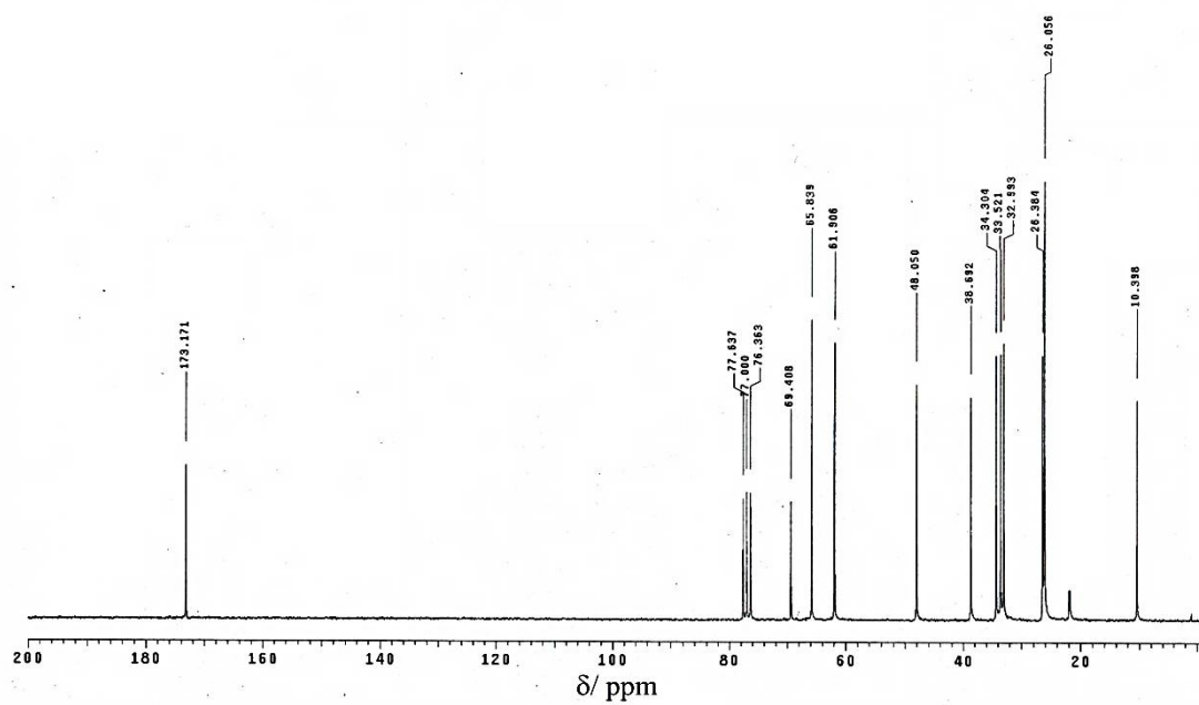
Slika P40. ^{13}\text{C} NMR spektar kompleksa K2.
