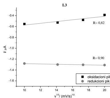
Slika 27. a) Ciklični voltamogrami 0,1 \text{ mmol}/\text{dm}^3 rastvora liganda L3 u DMSO-u pri različitim vrednostima brzina polarizacije (100, 200, 300 i 400 \text{mV/s} ); b) zavisnost jačine struje oksidacionog i redukcionog pika od kvadratnog korena brzine snimanja.
