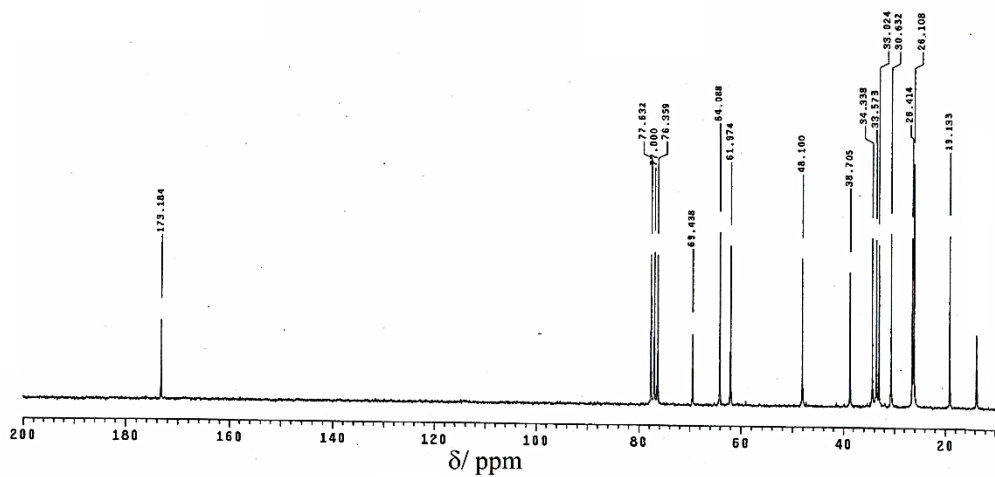
Slika P50. ^{13}\text{C} NMR spektar kompleksa K4.
