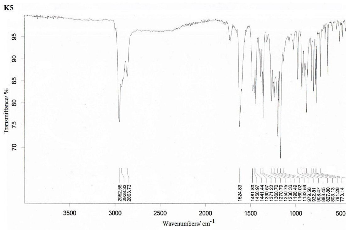
Slika P57. Infracrveni spektar kompleksa K5 .
