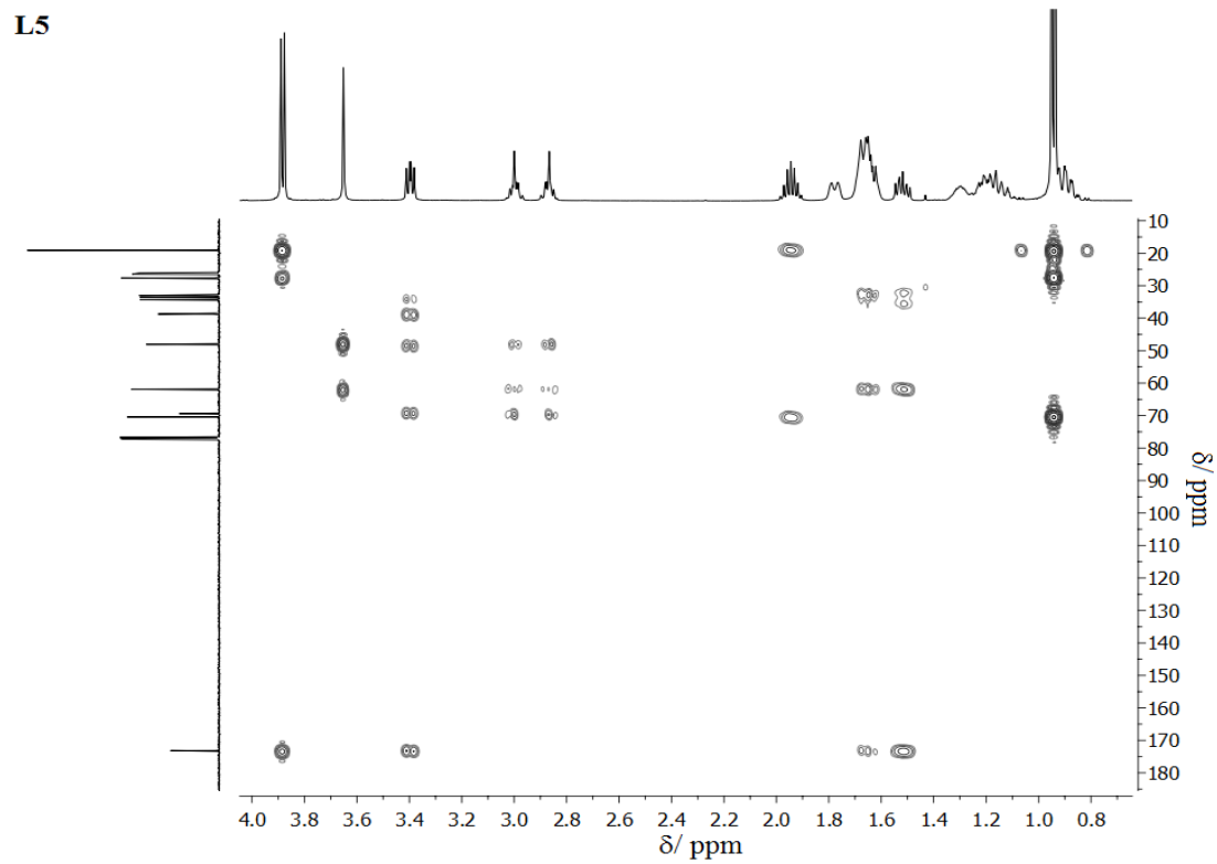
Slika P23. HSQC NMR spektar liganda L5 .
