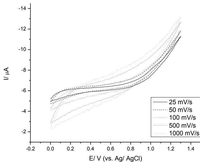
Slika P64. Ciklični voltamogram 0,1 mmol/dm 3 rastvora kompleksa K 2 [PtCl 6 ] u DMSO-u u oblasti potencijala 0 < E < 1,3 \text{ V} pri različitim vrednostima brzina polarizacije (25, 50, 100, 500, 1000 mV/s).
