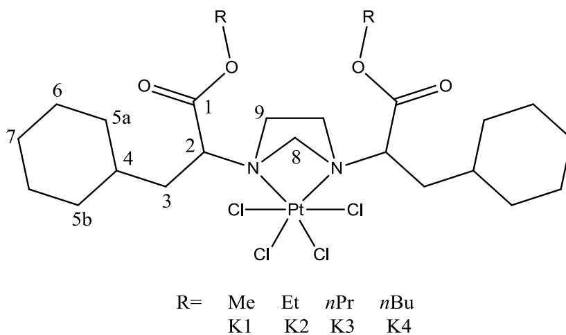
Slika 19. Struktura Pt(IV) kompleksa K1-4 sa odgovarajućom numeracijom C atoma.
