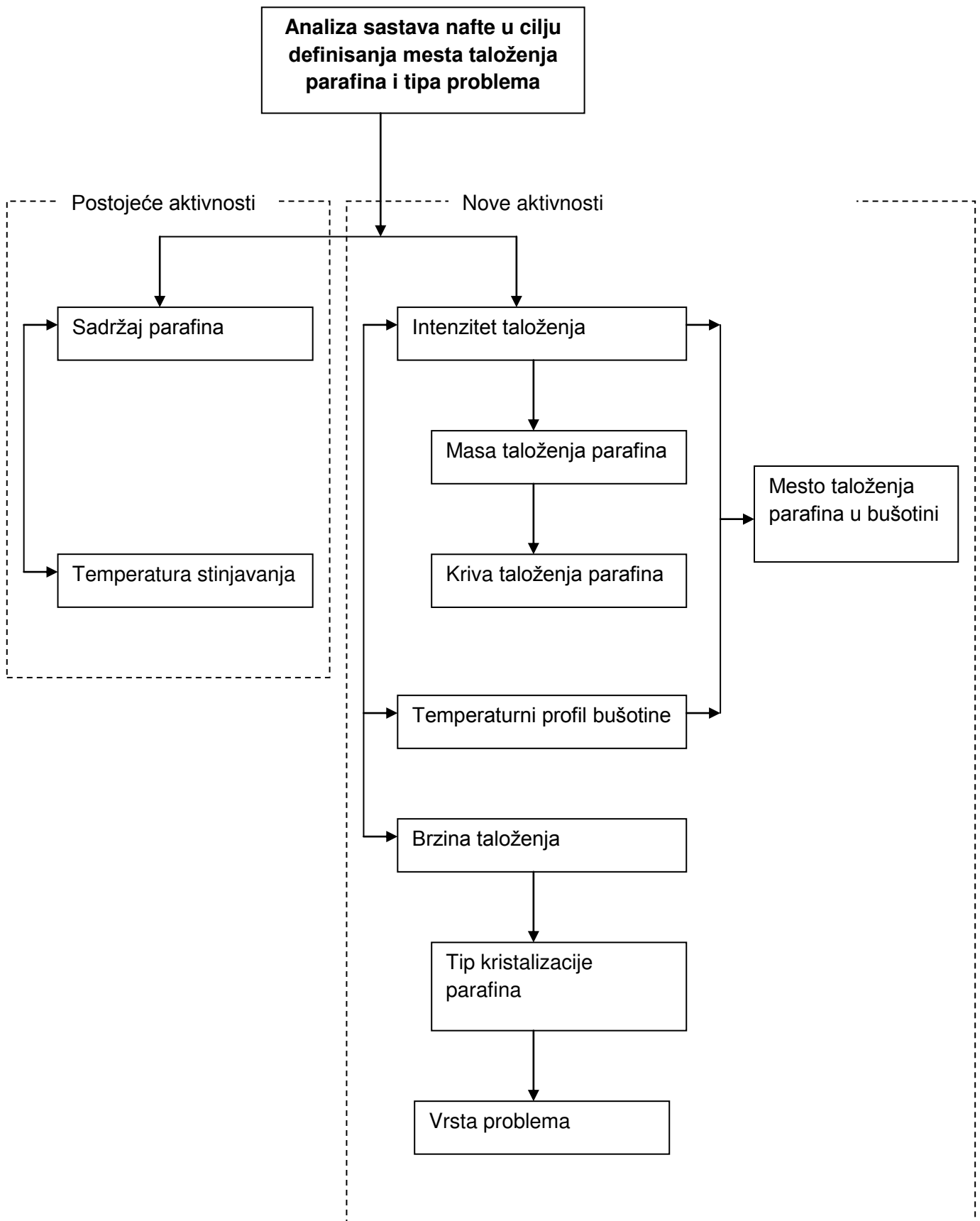
Slika 5.2. Analiza sastava nafte u cilju definisanja mesta taloženja parafina u proizvodnom sistemu i tip problema
