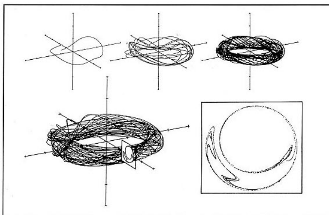
Слика 11.: Приказ чудног атрактора и Поенкареове мапе (Преузето из: Gleick, James. Chaos: Making a New Science . New York: Penguin Books, 1987, p 143)
