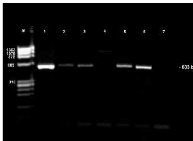
Slika 10. Elektroforeza u agaroznom gelu amplifikovanog fragmenta mecA gena veli ine 533-bp: M- X174 DNA/BsuRI (HaeIII) Marker, 9; 1-3 mecA pozitivni izolati S. haemolyticus ;4- mecA negativan izolat; 5- mecA pozitivan izolat S. capitis ; 6- pozitivna kontrola MRSA ATCC 43300; 7- negativna kontrola S. aureus ATCC 25923
