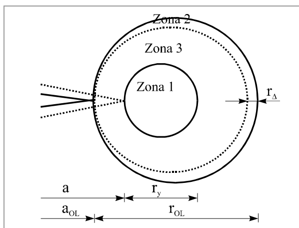
Slika 4.7 Definisane zone oko vrha prsline i parametara za formulisanje matematičkog modela u slučaju dejstva nadopterećenje/podopterećenje
