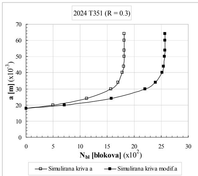
Slika 6.27 Analiza širenja prsline CT uzorka pri dejstvu spektra opterećenja.
