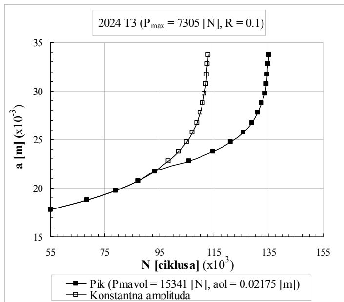
Slika 6.33 Funkcionalna zavisnost između broja ciklusa opterećenja do pojave loma N i dužine prsline a u slučaju opterećenja konstantne amplitude bez i sa pikom ( P_{\max ol} = 1534 [N], a_{ol} = 21.75 [mm]).
