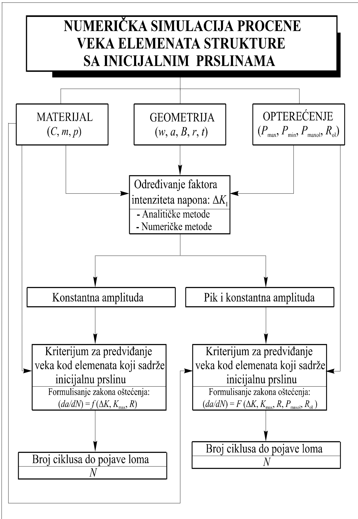
Slika 5.4 Algoritam matematičkog modela za simulaciju širenja prsline u uslovima dejstva pika opterećenja.
