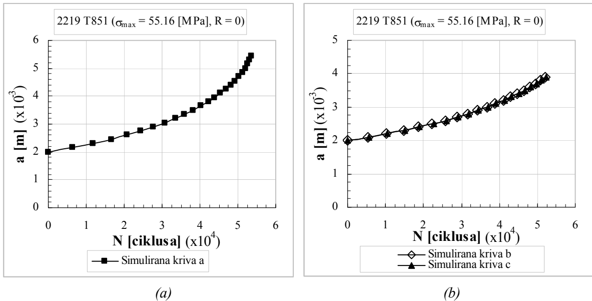
Slika 6.19 Funkcionalna zavisnost između broja ciklusa N do loma i dužine prsline a (kriva a - bazirana na jednačini (3.3.16) i analitičkoj relaciji (Tabela 3.1), kriva b - bazirana na jednačinama (3.3.16), (3.3.51) i (6.1.1), kriva c - bazirana na jednačinama (3.3.16), (3.3.51) i (6.1.2)).
