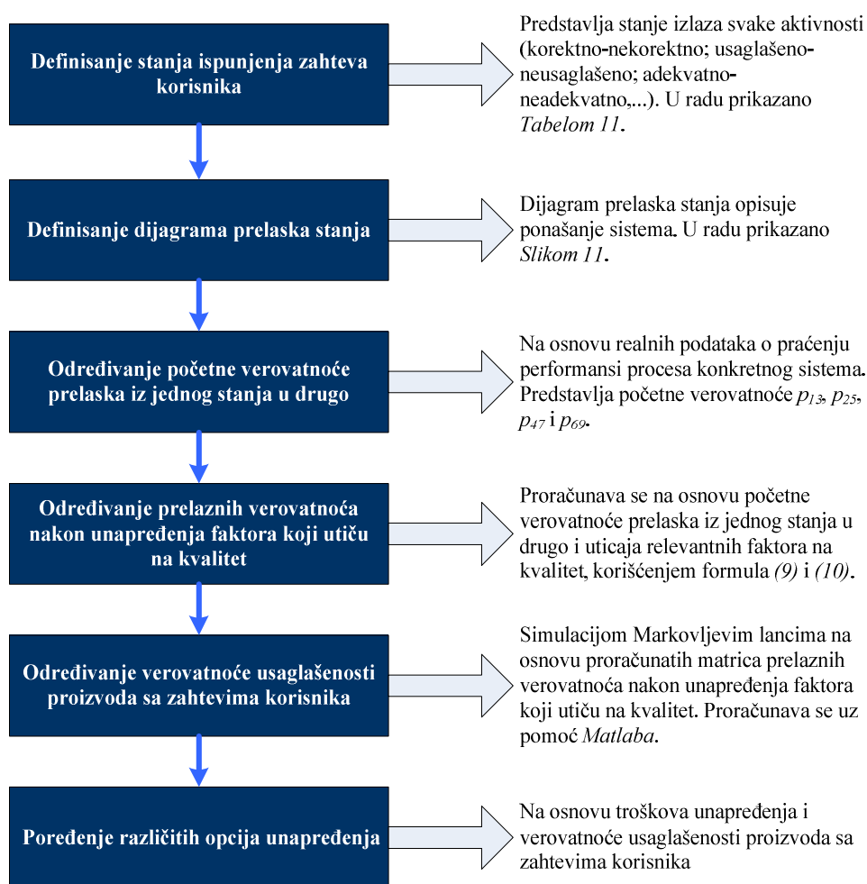
Slika 10 Algoritam izbora optimalne strategije
