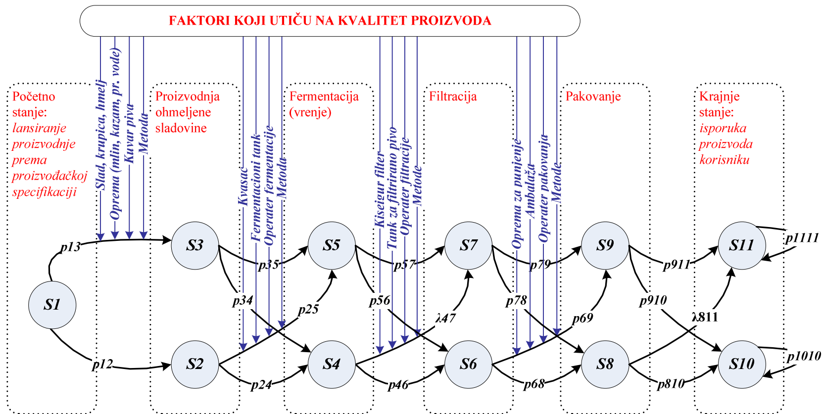
Slika 13 Validacija modela - dijagram prelaska stanja
