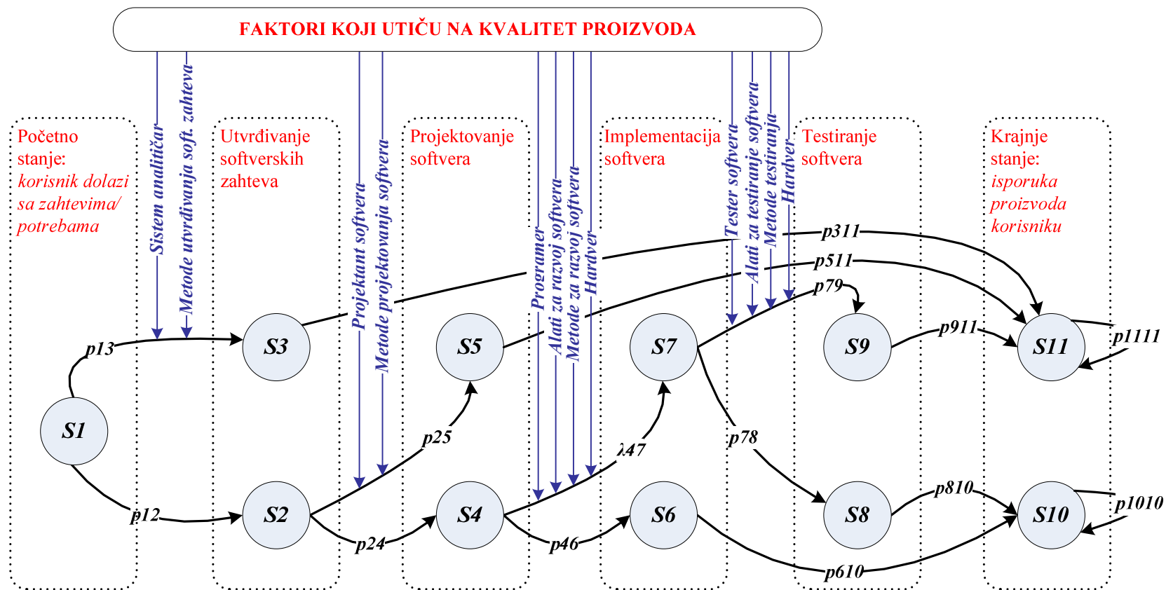
Slika 20 Dijagram prelaska stanja na primeru softvera
