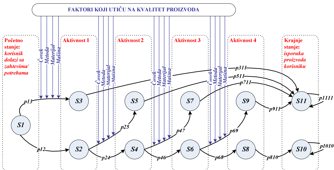
Slika 11 Dijagram prelaska stanja
