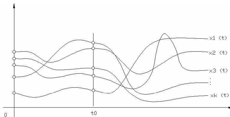
Slika 1 Trajektorija stohastičkog procesa (Izvor: Zečević, 1974)
